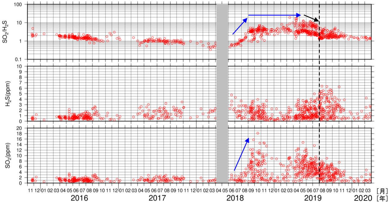
図9 吾妻山 火山ガス観測装置による観測（2015年11月～2020年3月）
