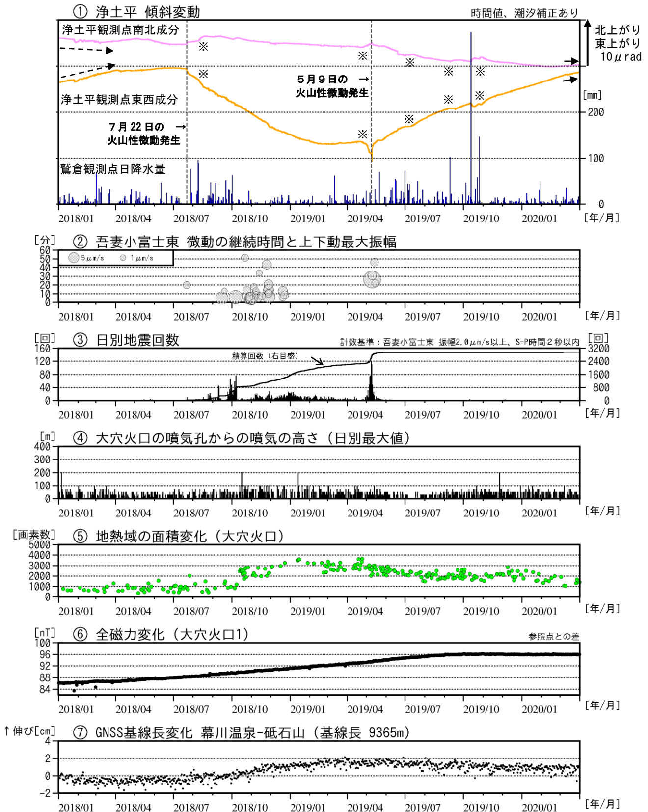
図1 吾妻山 火山活動経過図 (2018年1月~2020年3月)
