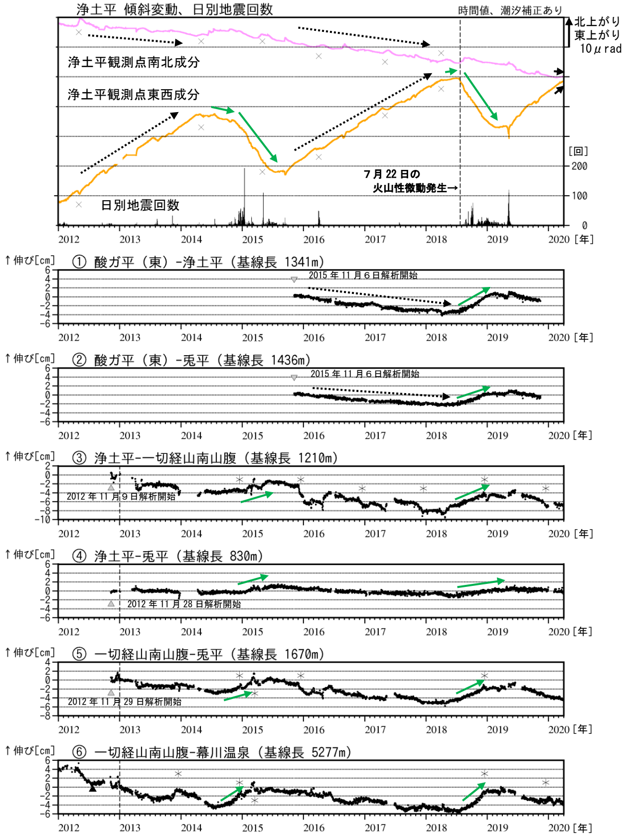
図3 吾妻山 傾斜変動及びGNSS基線長変化図（2012年1月～2020年3月）
