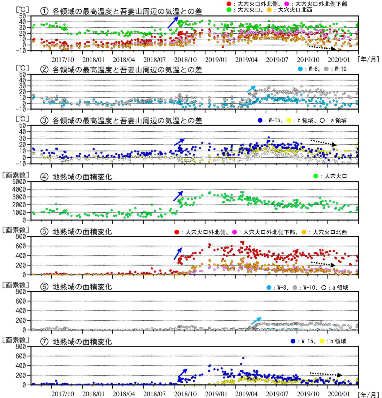
図7 吾妻山 監視カメラによる大穴火口周辺の地熱域の経過（2017年8月～2020年3月）
