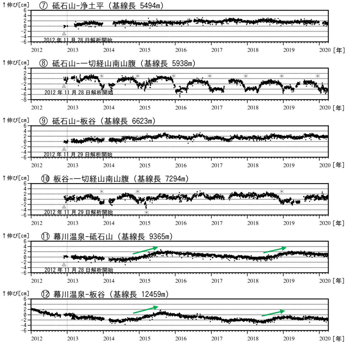
図4 吾妻山 GNSS 基線長変化図（2012年1月～2020年3月）
