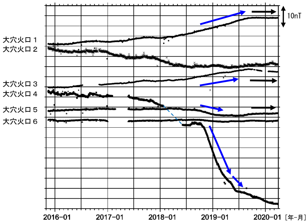
図11 吾妻山 全磁力連続観測点の全磁力値変化（2015年11月～2020年3月）
