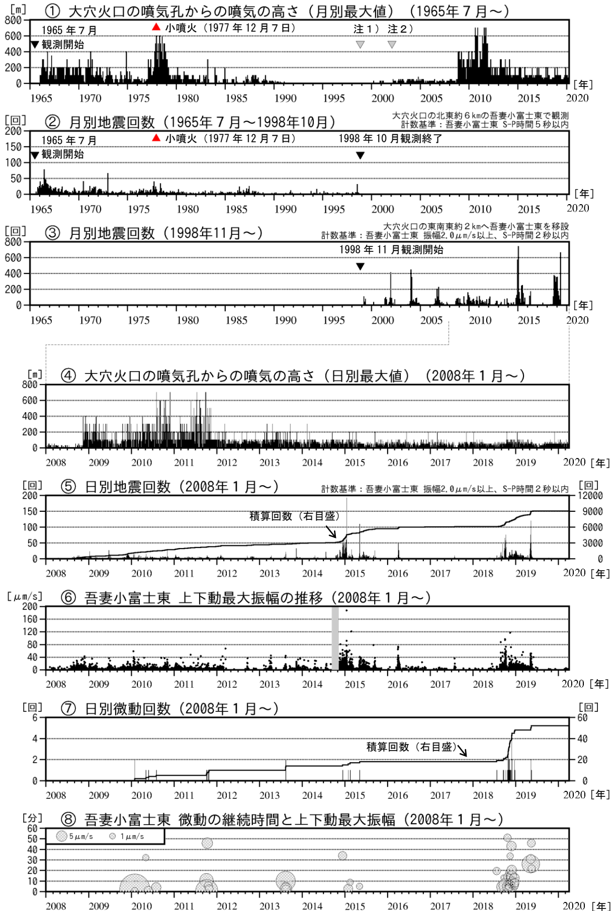
図2 吾妻山 火山活動経過図（1965年7月～2020年3月）
