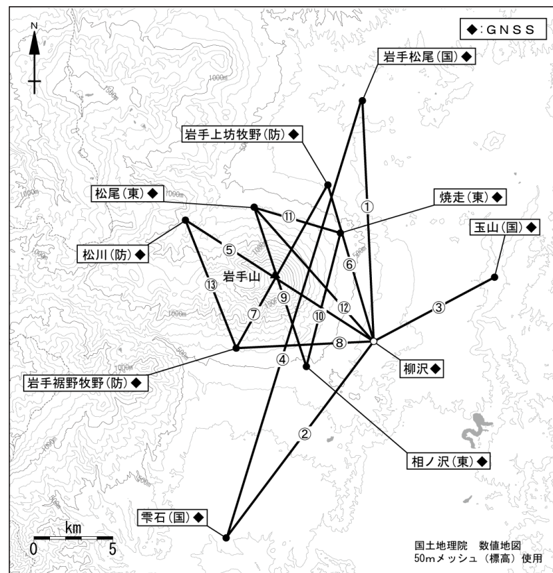
図7 岩手山 GNSS 観測基線図
