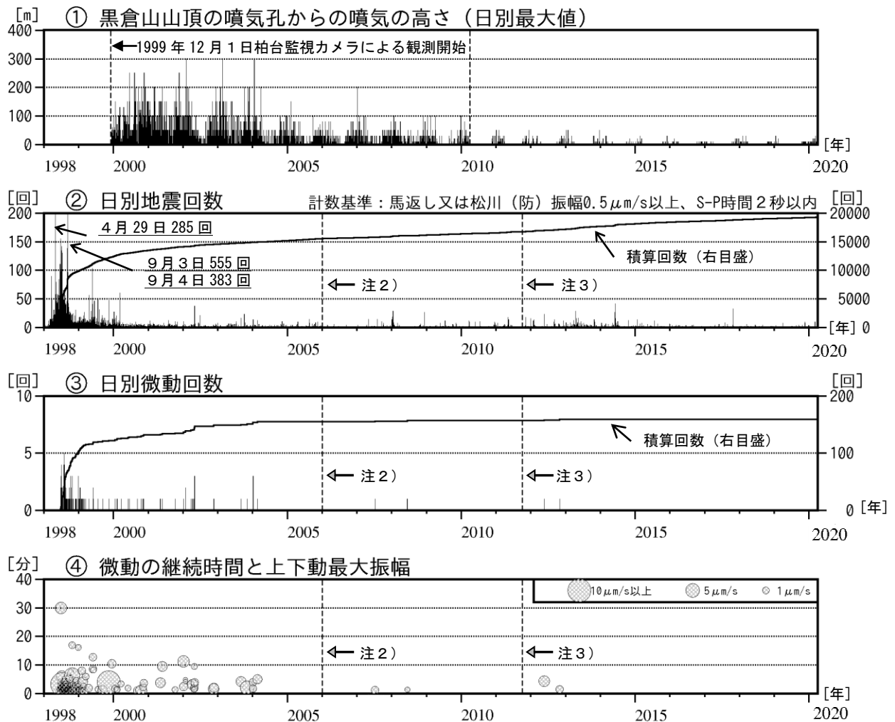
図2 岩手山 火山活動経過図（1998年1月～2020年3月）
