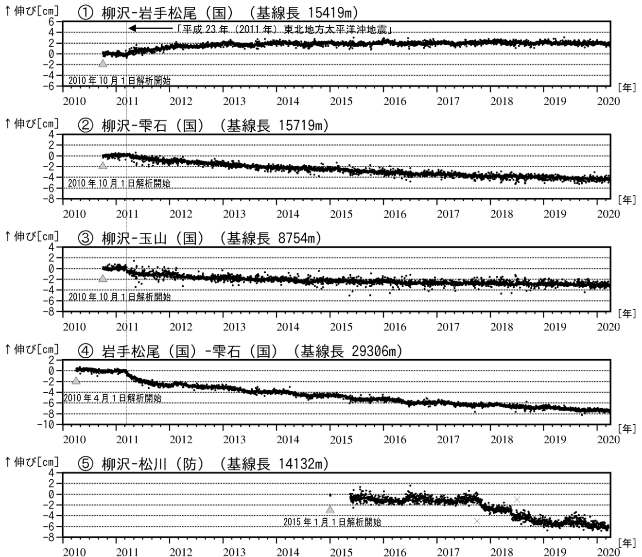
図4 岩手山 GNSS 基線長変化図（2010年4月～2020年3月）
