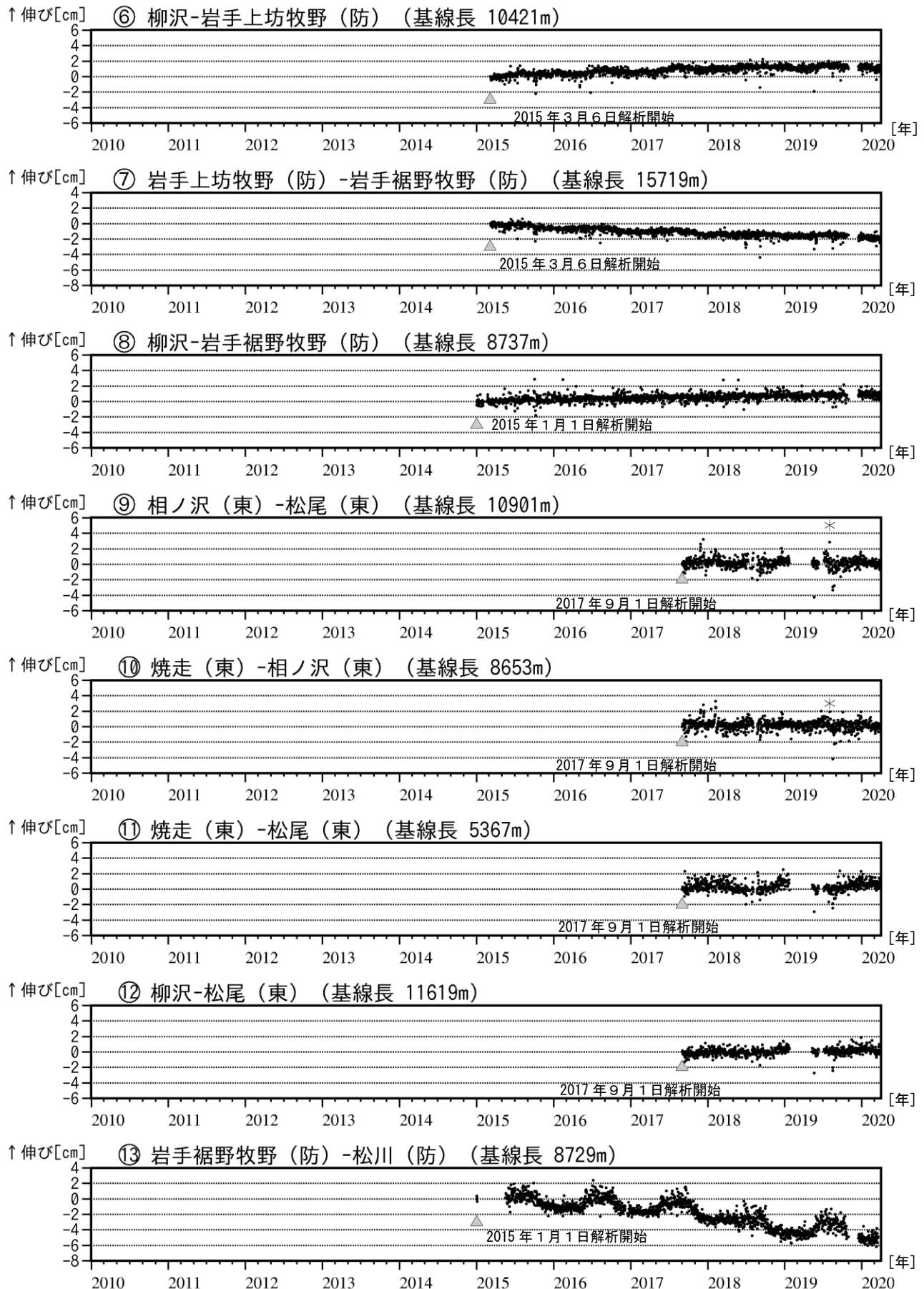
図5 岩手山 GNSS 基線長変化図 (2015年1月～2020年3月)
