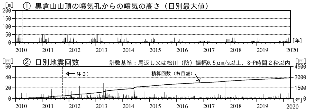
図3 岩手山 噴気の高さ及び日別地震回数（2010年1月～2020年3月）
