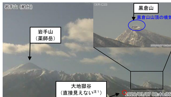
図1 岩手山 黒倉山の噴気の状況（3月7日）
