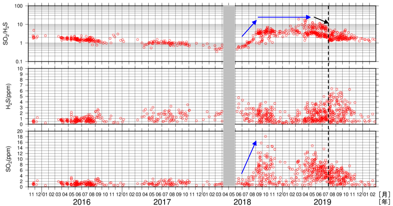
図 12 吾妻山 火山ガス観測装置による観測（2015年11月～2020年2月）
