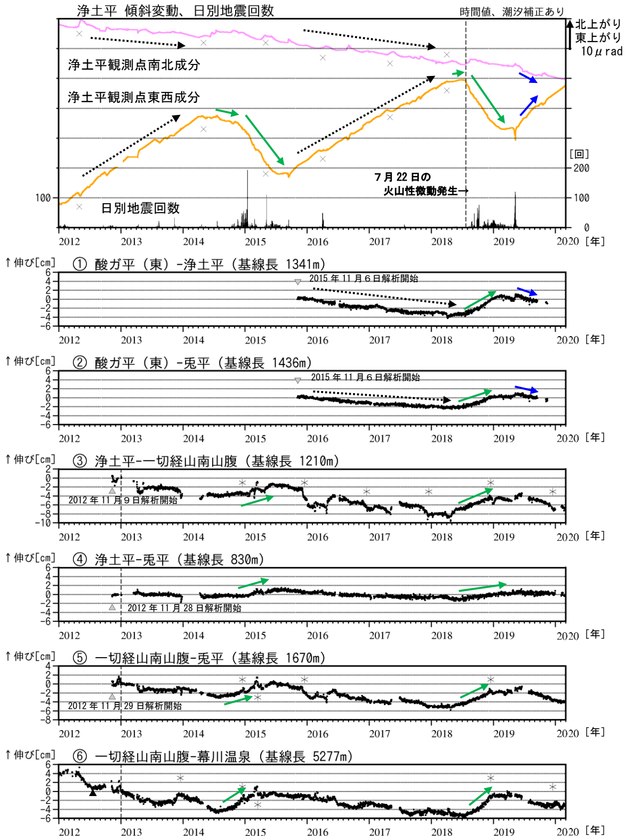
図3 吾妻山 傾斜変動及びGNSS基線長変化図（2012年1月～2020年2月）
