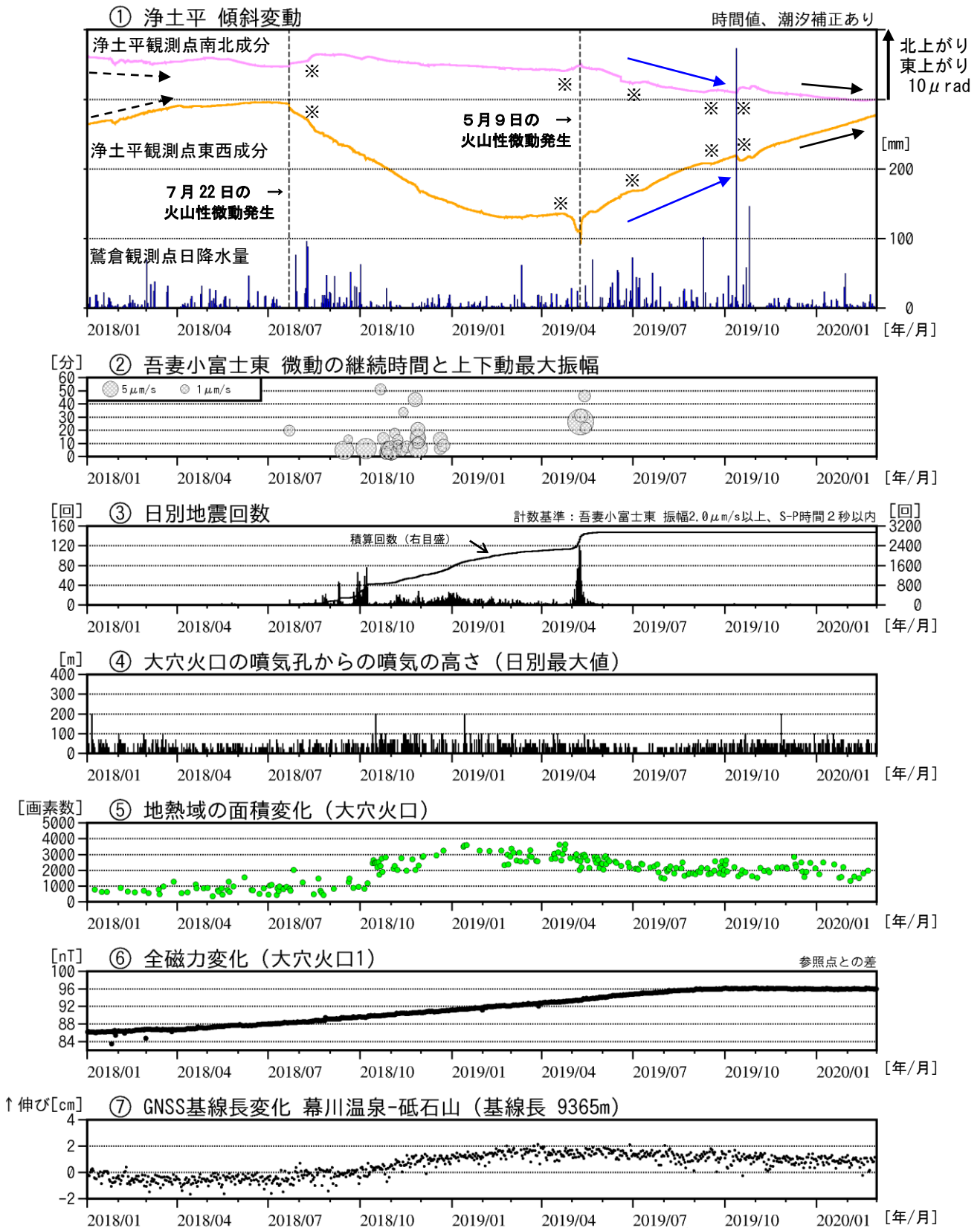
図1 吾妻山 火山活動経過図（2018年1月～2020年2月）
