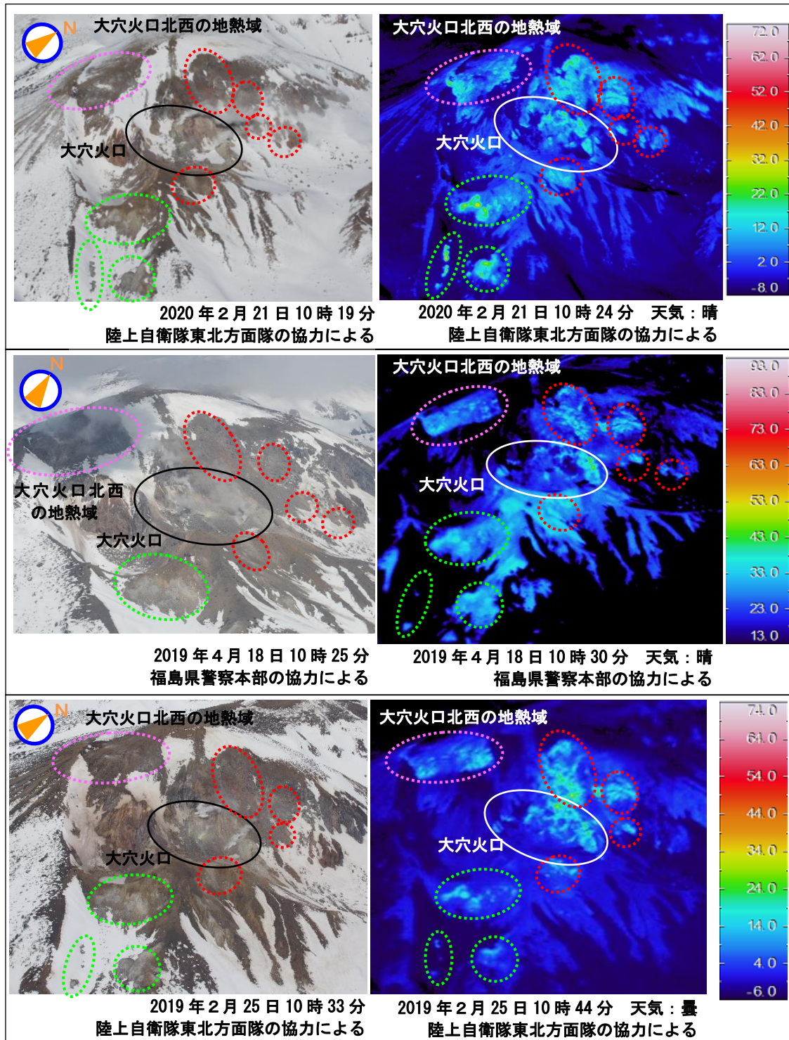
図10 吾妻山 上空から撮影した大穴火口及びその周辺の状況と地表面温度分布 ・大穴火口付近とその周辺に大きな変化は認められず、熱活動が継続していることを確認しました。 ・図中の破線の色は図9の破線の色に対応します。 ※日射の影響により、裸地等では表面温度が高めに表示されています。
