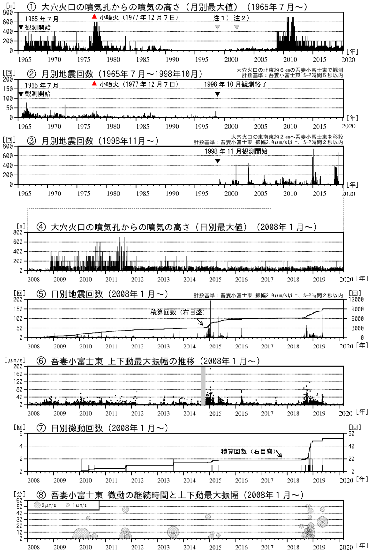
図2 吾妻山 火山活動経過図（1965年7月～2020年2月）
