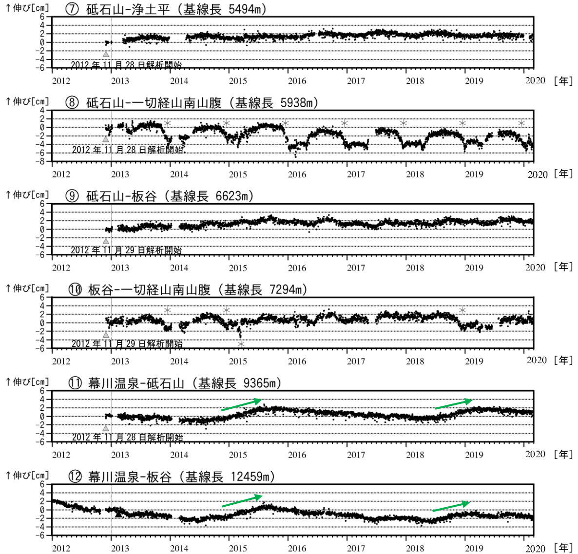
図4 吾妻山 GNSS 基線長変化図（2012年1月～2020年2月）
