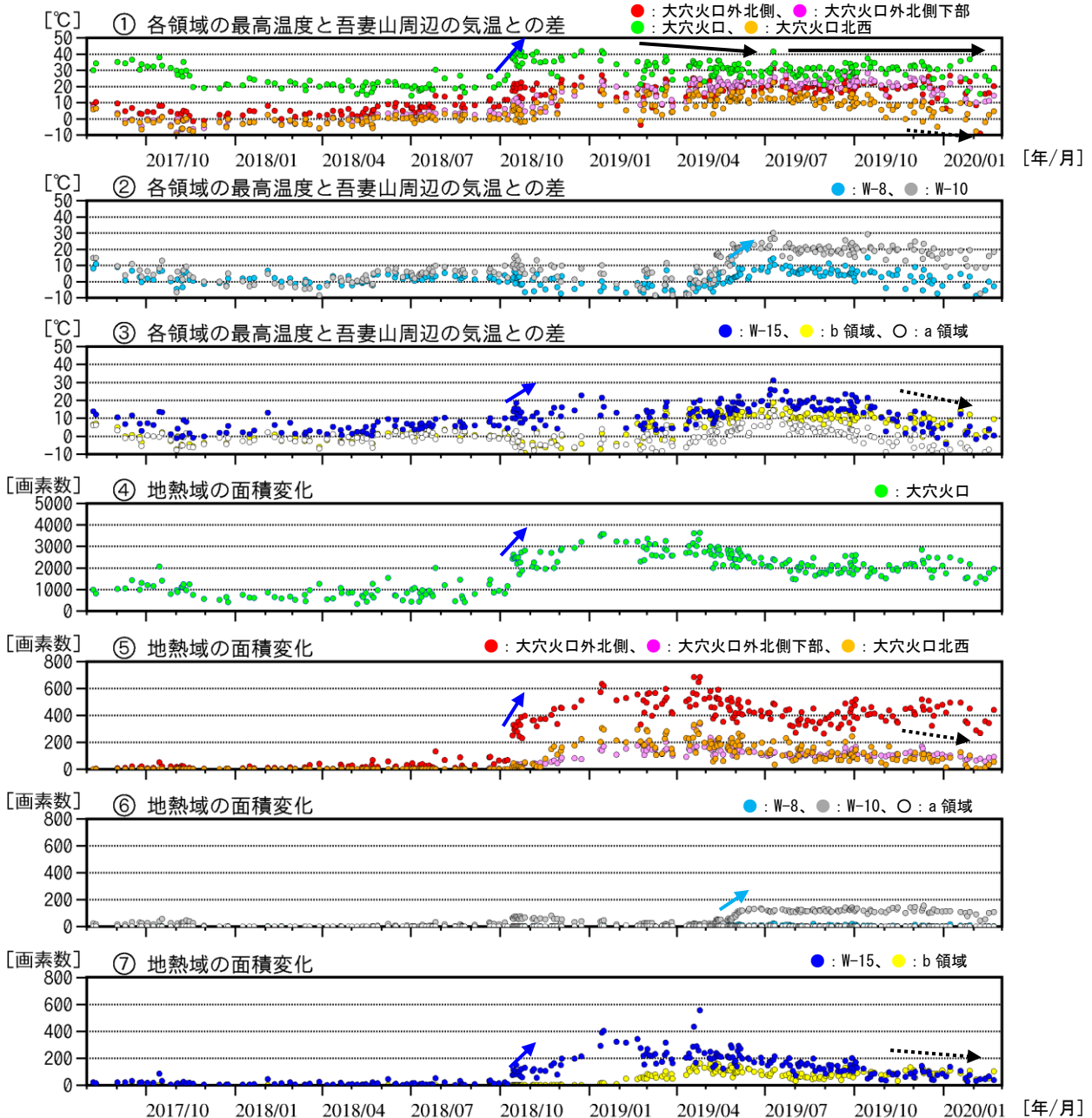
図7 吾妻山 監視カメラによる大穴火口周辺の地熱域の経過（2017年8月～2020年2月）
