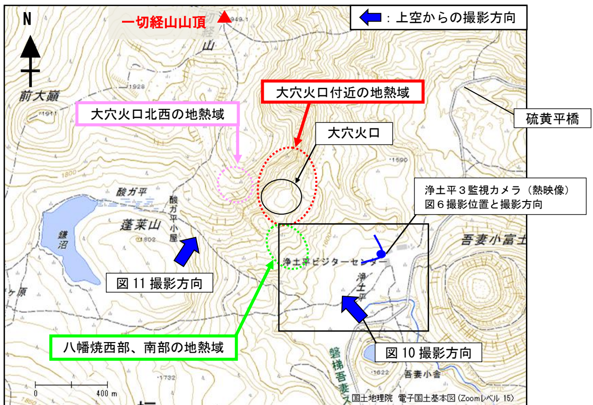
図9 吾妻山 大穴火口周辺の噴気と地熱域の分布及び写真と地表面温度分布撮影方向
