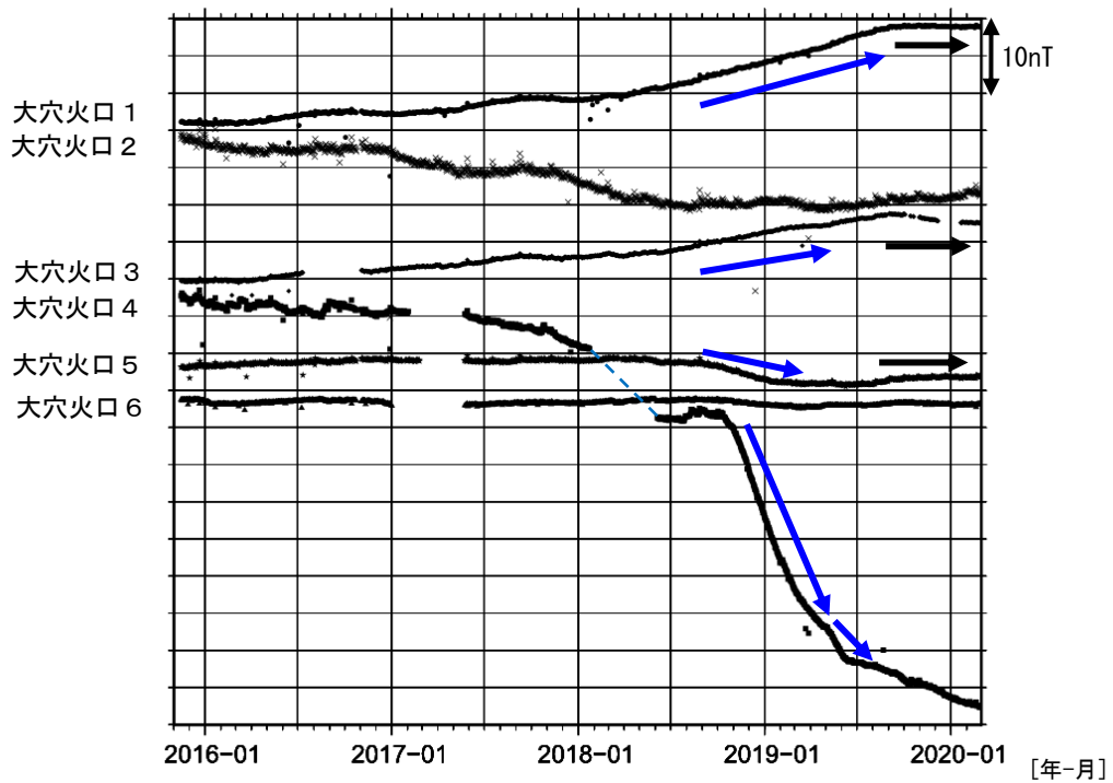
図14 吾妻山 全磁力連続観測点の全磁力値変化（2015年11月～2020年2月）
