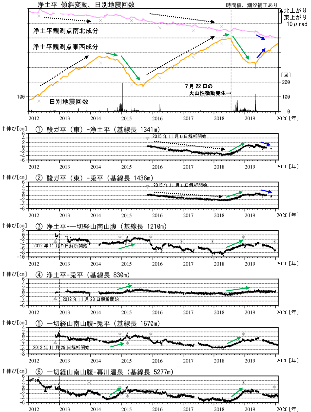
図3 吾妻山 傾斜変動及びGNSS基線長変化図(2012年1月~2020年1月)
