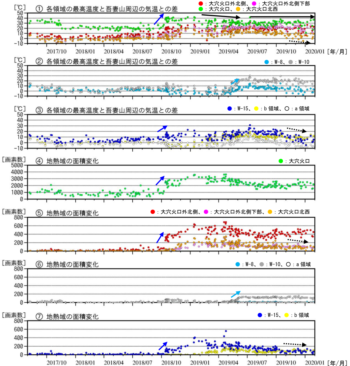
図7 吾妻山 監視カメラによる大穴火口周辺の地熱域の経過（2017年8月～2020年1月）
