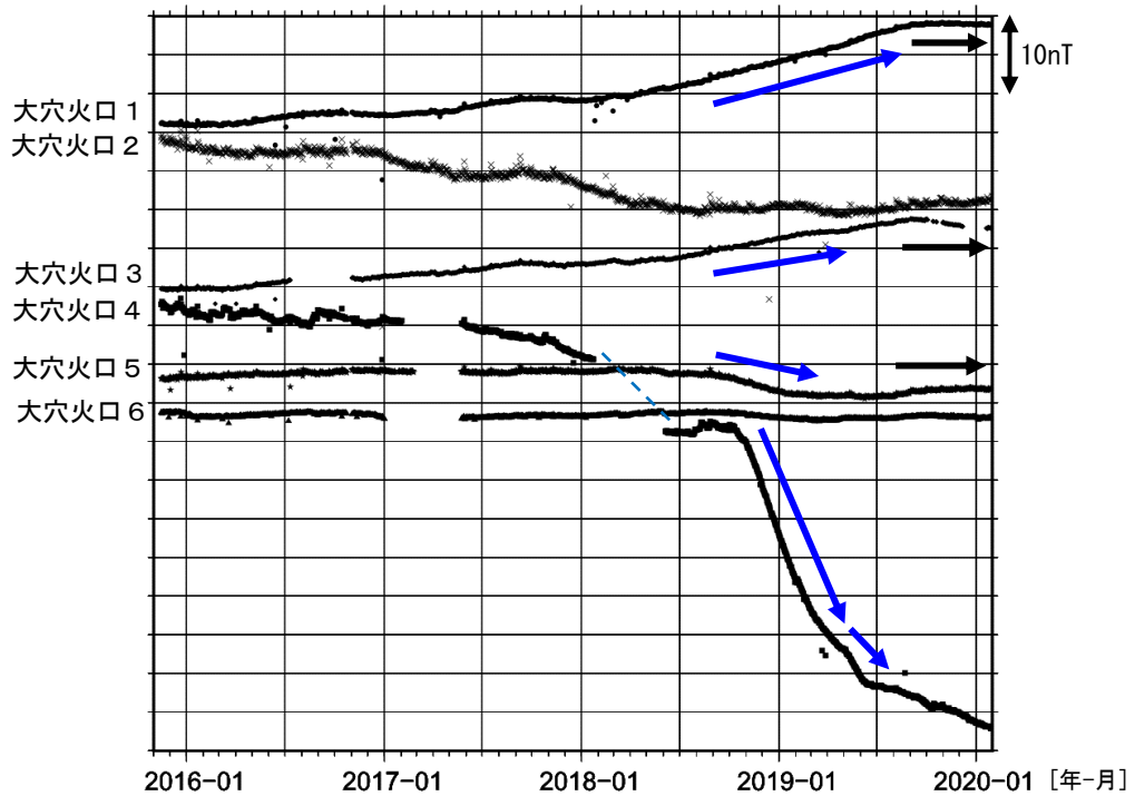
図11 吾妻山 全磁力連続観測点の全磁力値変化（2015年11月～2020年1月）
