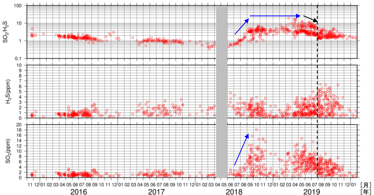
図9 吾妻山 火山ガス観測装置による観測（2015年11月～2020年1月）
