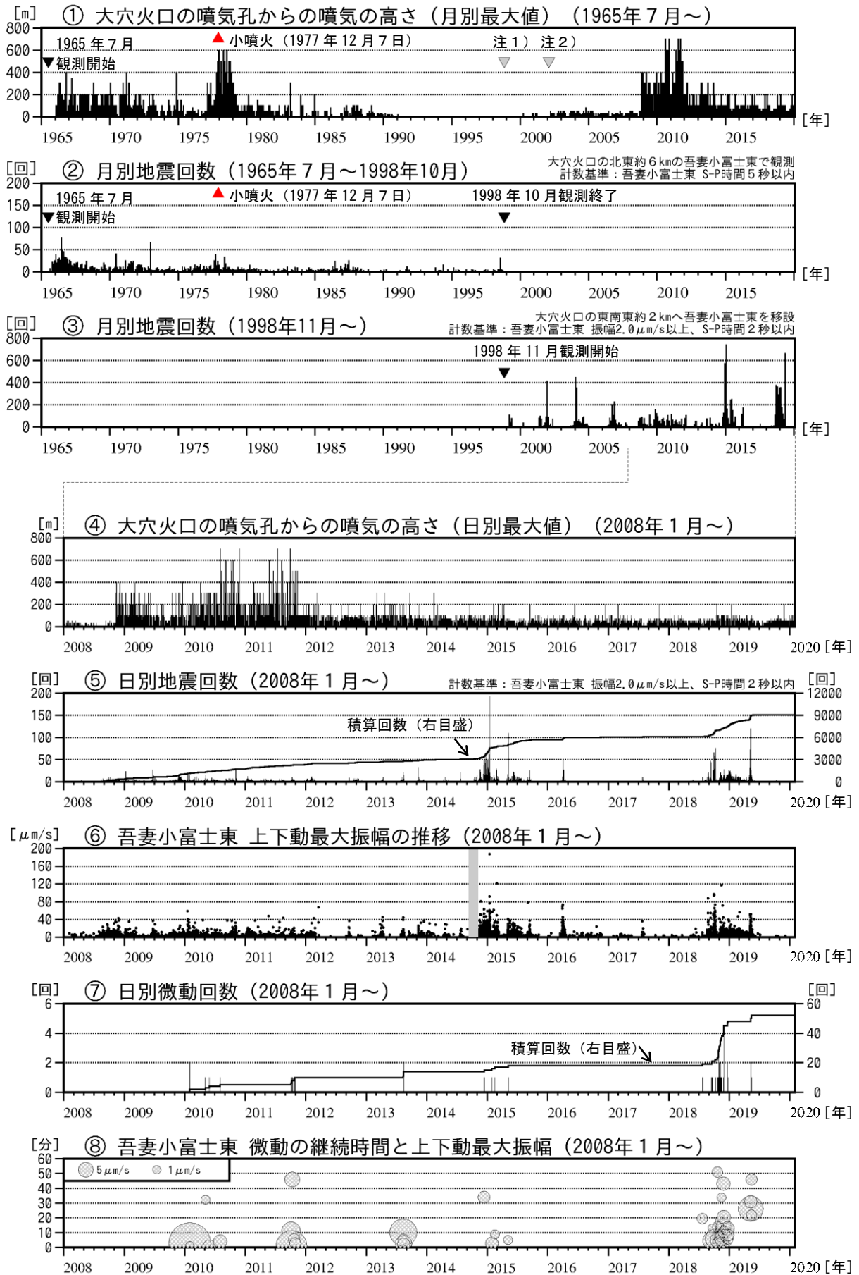
図2 吾妻山 火山活動経過図（1965年7月～2020年1月）
