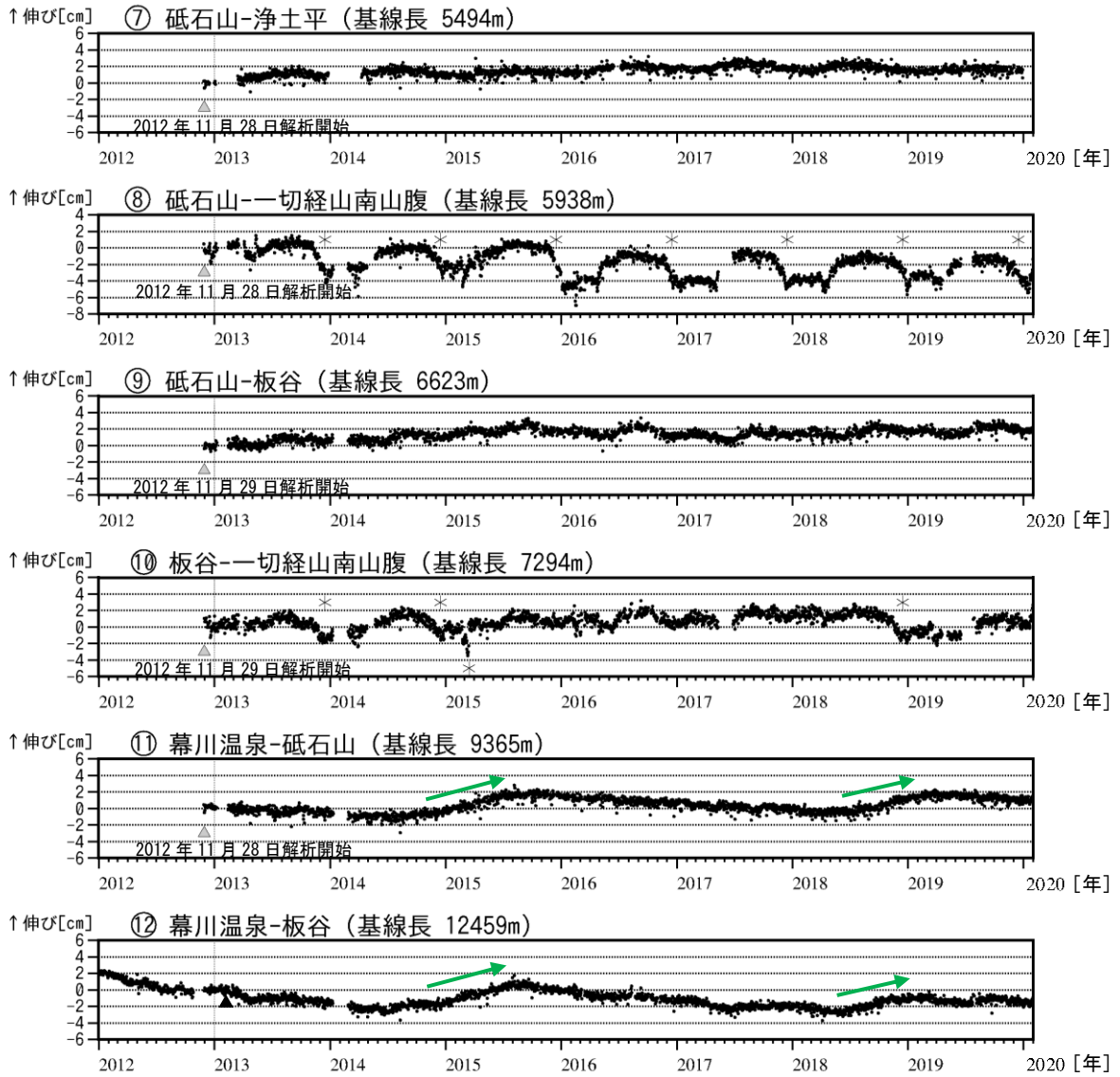
図4 吾妻山 GNSS 基線長変化図（2012年1月～2020年1月）
