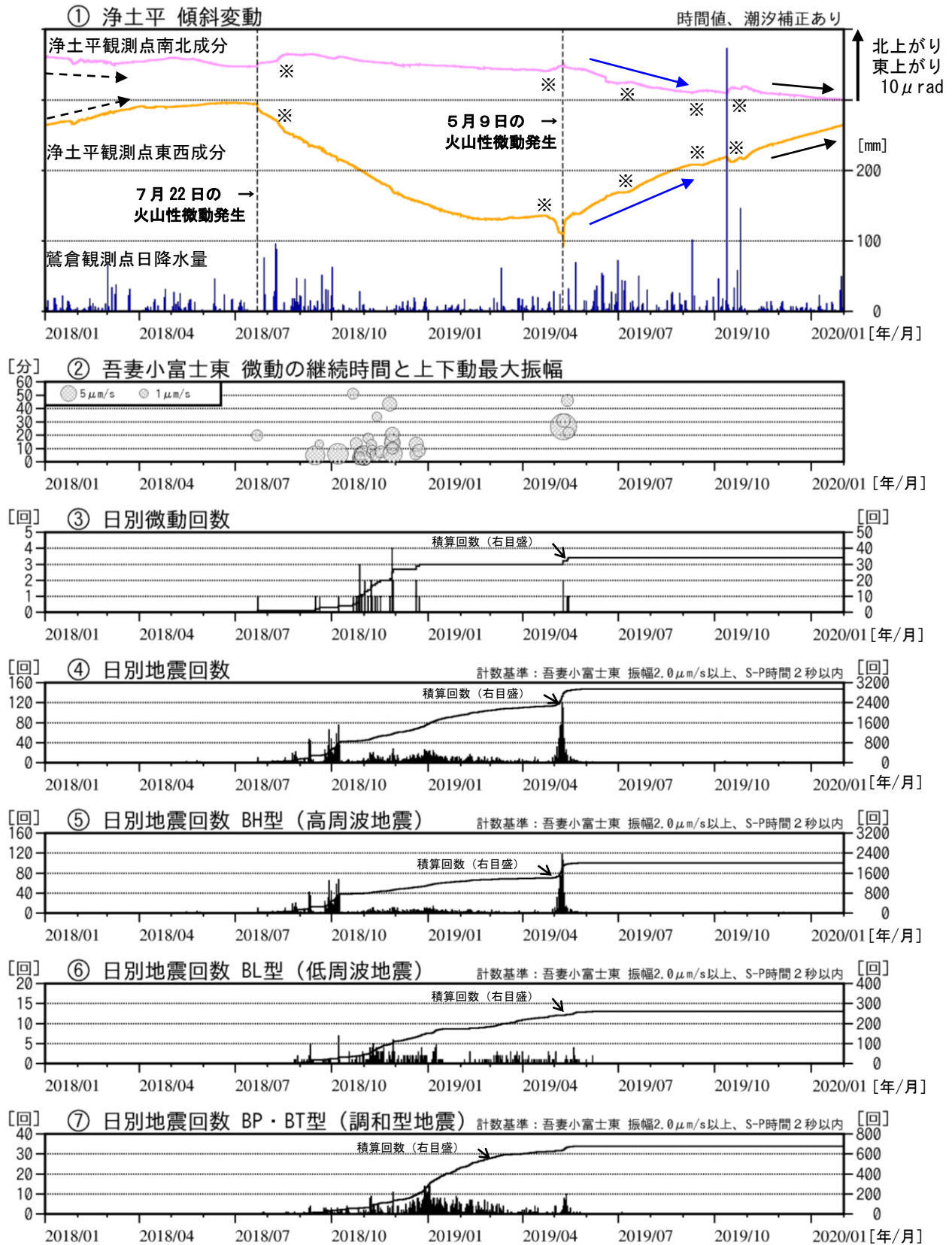
図1 吾妻山 浄土平観測点における傾斜変動、火山性微動の発生状況及び日別地震回数 (2018年1月~2020年1月)
