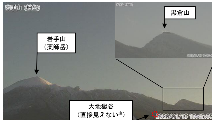
図1 岩手山 黒倉山の噴気の状況（1月13日）
