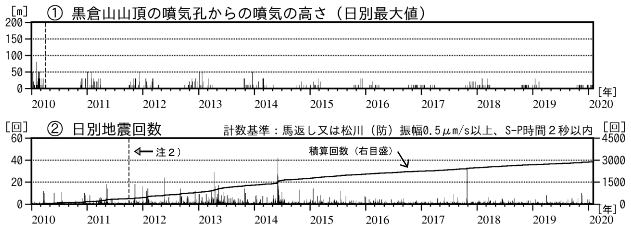
図3 岩手山 噴気の高さ及び日別地震回数（2010年1月～2020年1月）
