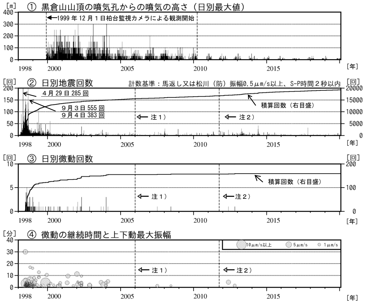
図2 岩手山 火山活動経過図（1998年1月～2020年1月）
