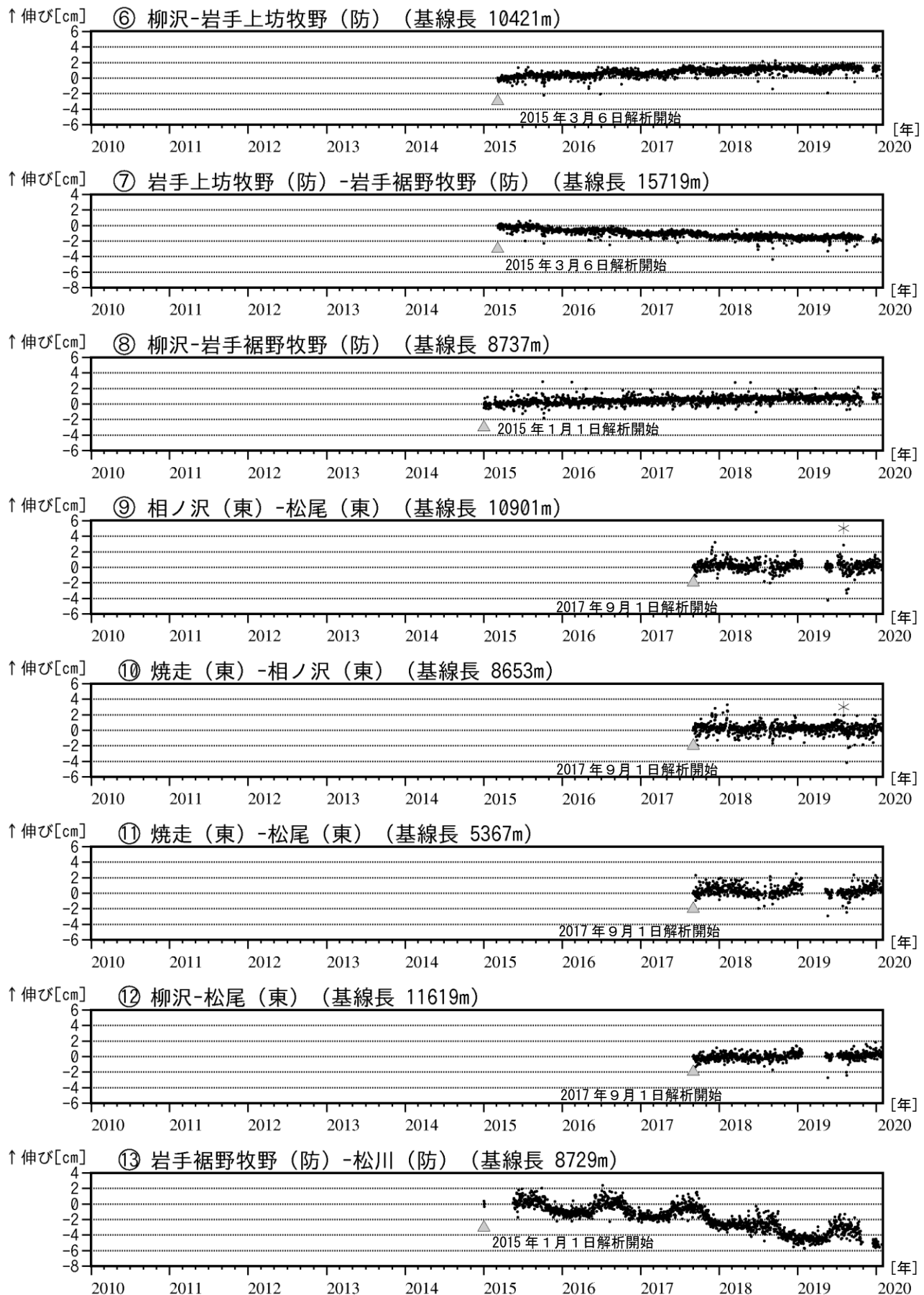
図5 岩手山 GNSS 基線長変化図（2015年1月～2020年1月）
