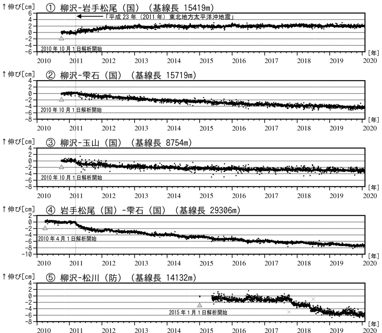
図4 岩手山 GNSS 基線長変化図（2010年4月～2020年1月）
