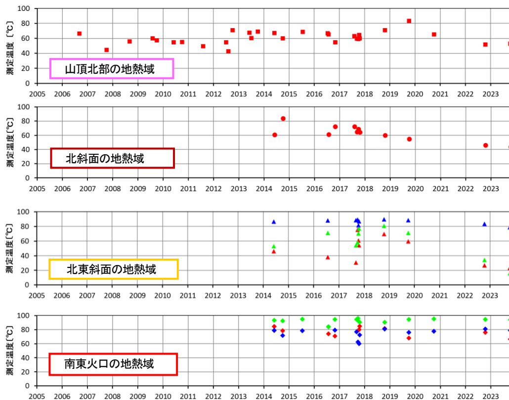
図10 女岳の地熱域における地中温度 (2006年9月～2023年10月)
