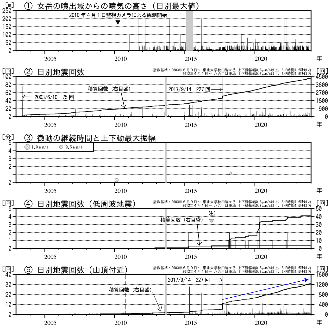
図11 秋田駒ヶ岳 火山活動経過図（2003年6月～2023年12月）
