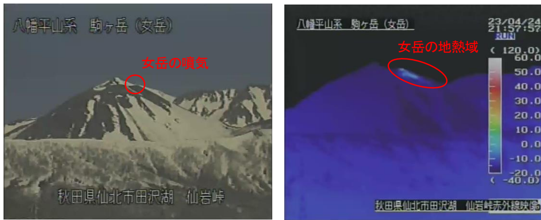
図1 秋田駒ヶ岳 女岳周辺の噴気と地表面温度分布の状況（可視：4月2日、赤外：4月24日） ・東北地方整備局が設置している仙岩峠監視カメラ（女岳山頂の南約5km）の可視及び赤外映像です。
