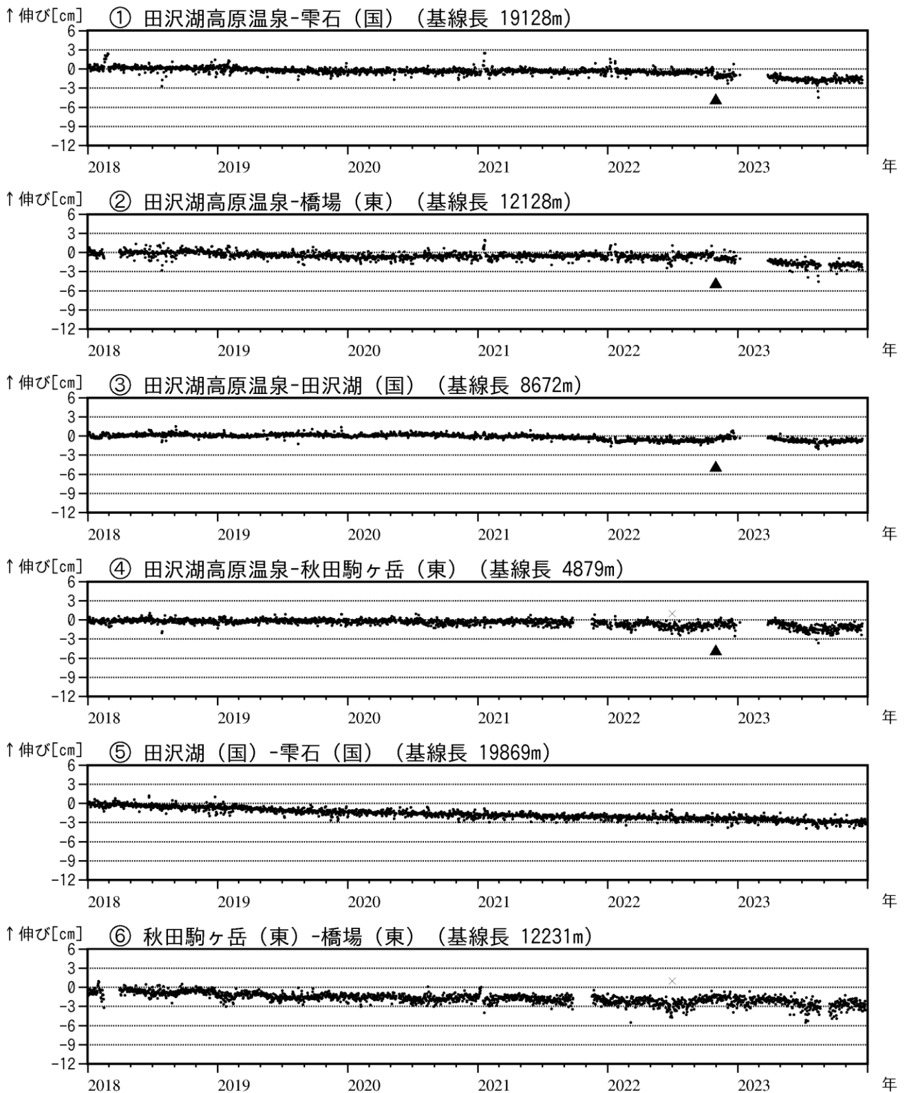
図14 秋田駒ヶ岳 GNSS 基線長変化図 (2018年1月~2023年12月)
