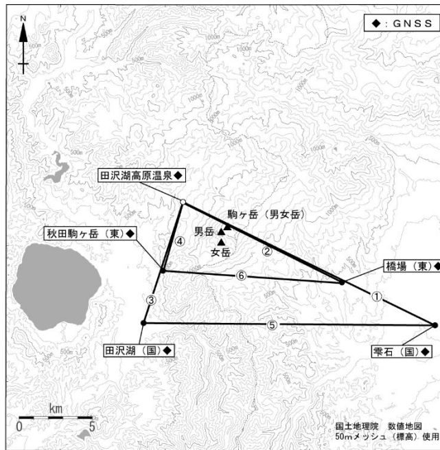
図 16 秋田駒ヶ岳 GNSS 観測基線図
