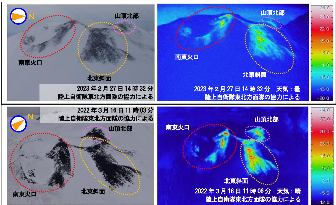
図8 秋田駒ヶ岳 上空からの南東火口の状況と地表面温度分布
