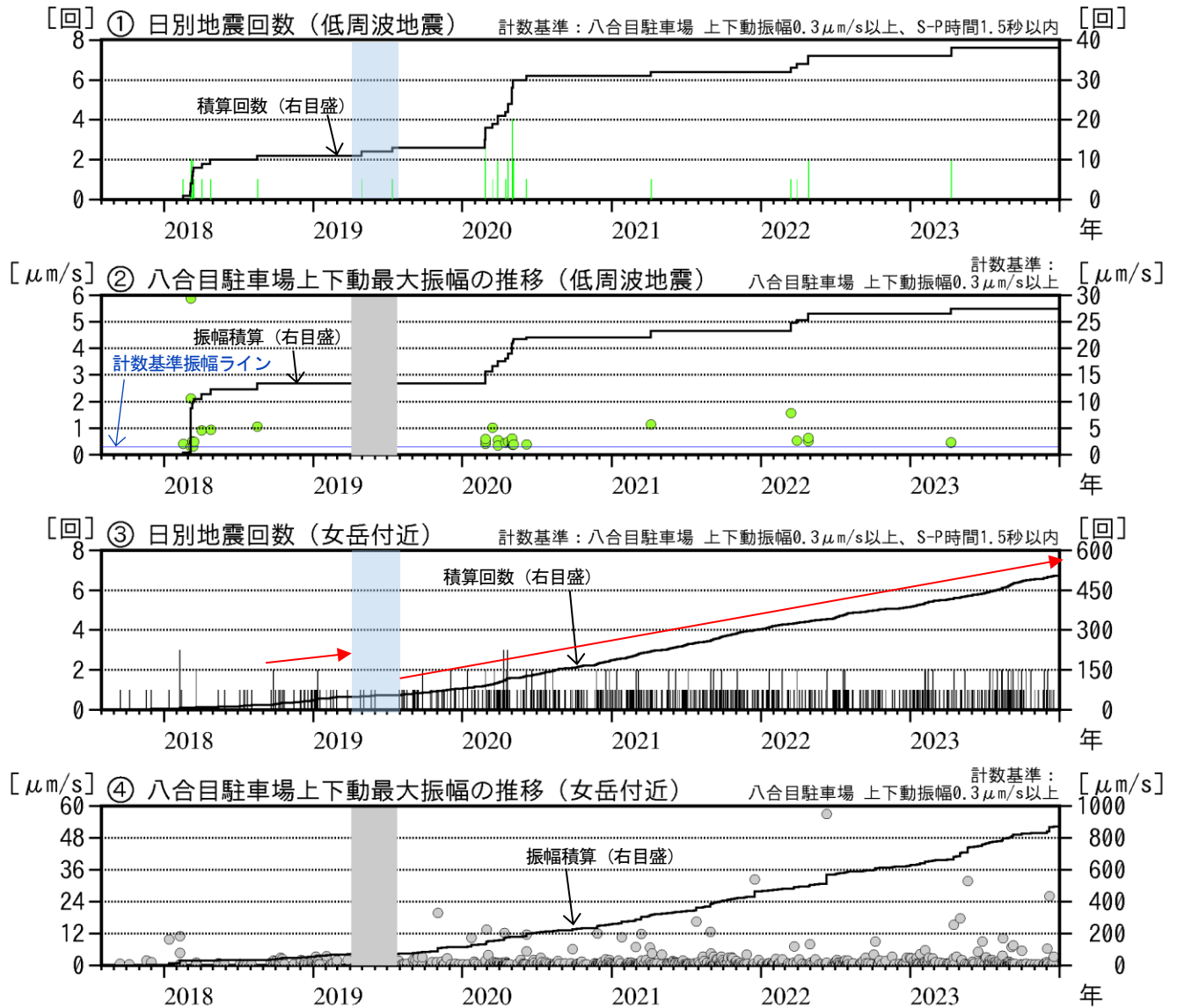
図12 秋田駒ヶ岳 低周波地震及び女岳付近の日別回数と最大振幅（2017年8月～2023年12月）
