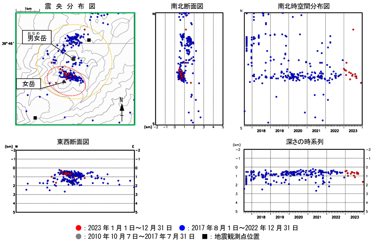
図13 秋田駒ヶ岳 地震活動 (2010年10月～2023年12月)
