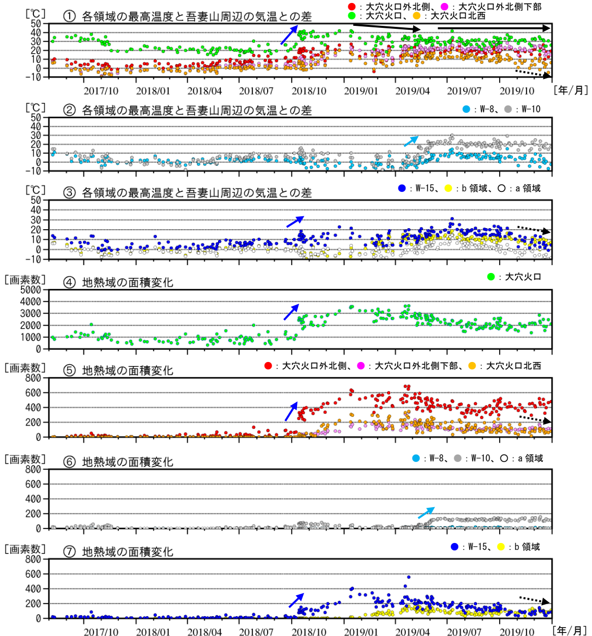
図7 吾妻山 監視カメラによる大穴火口周辺の地熱域の経過（2017年8月～2019年12月）
