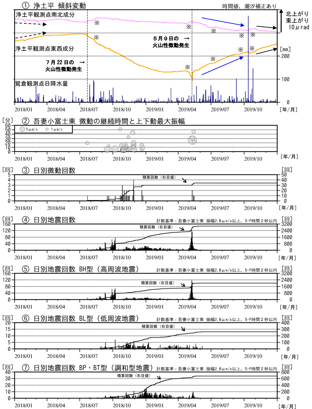
図1 吾妻山 浄土平観測点における傾斜変動、火山性微動の発生状況及び日別地震回数 (2018年1月~2019年12月)
