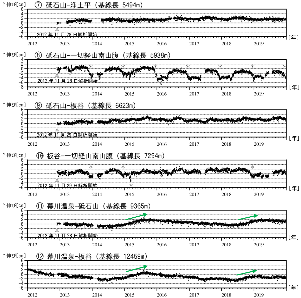
図4 吾妻山 GNSS 基線長変化図（2012年1月～2019年12月）
