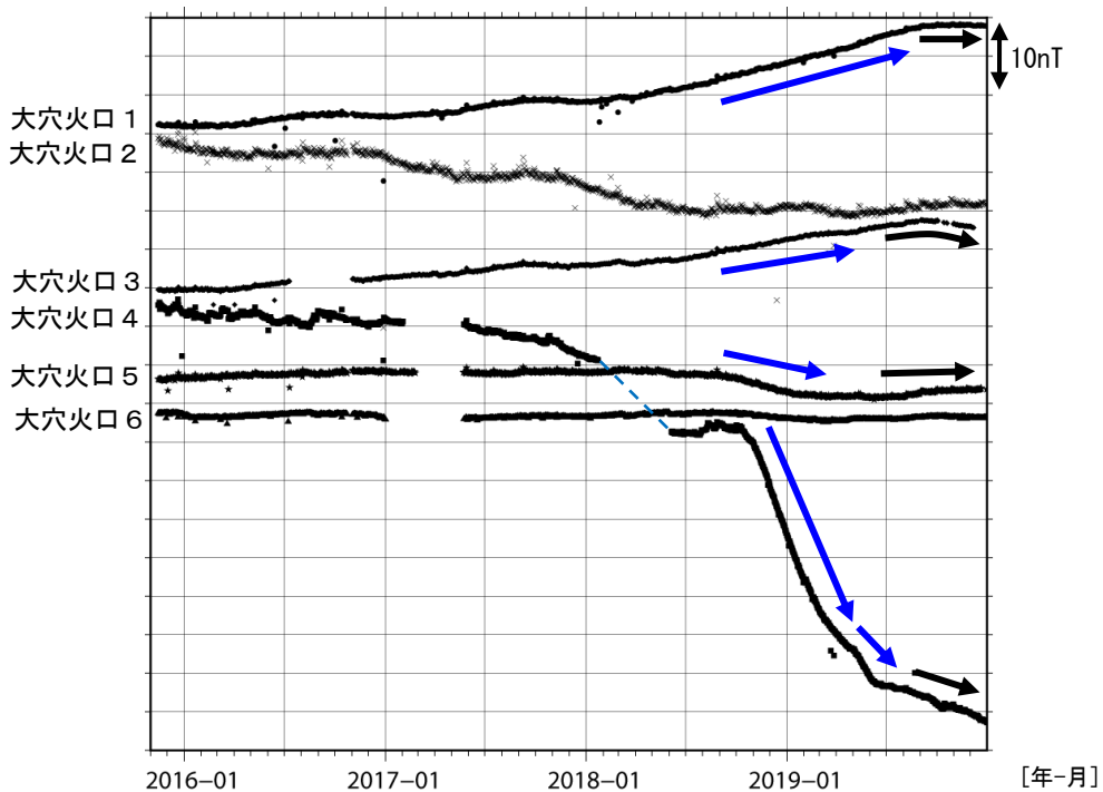
図 11 吾妻山 全磁力連続観測点の全磁力値変化（2015 年 11 月～2019 年 12 月）
