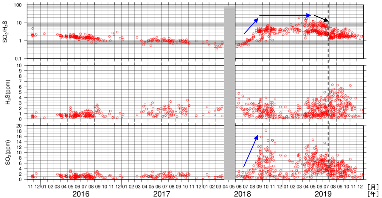
図9 吾妻山 火山ガス観測装置による観測（2015年11月～2019年12月）
