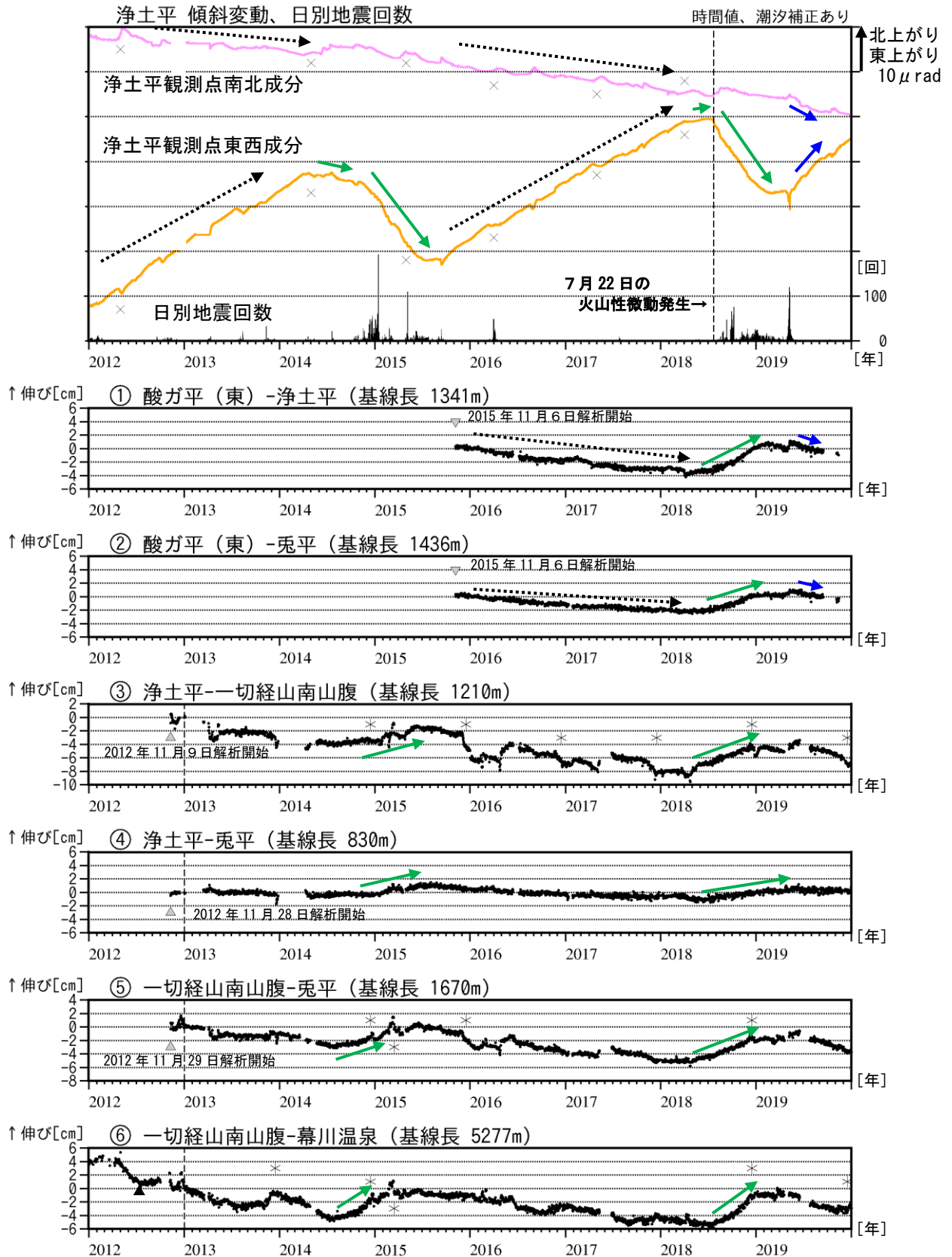
図3 吾妻山 傾斜変動及びGNSS基線長変化図（2012年1月～2019年12月）
