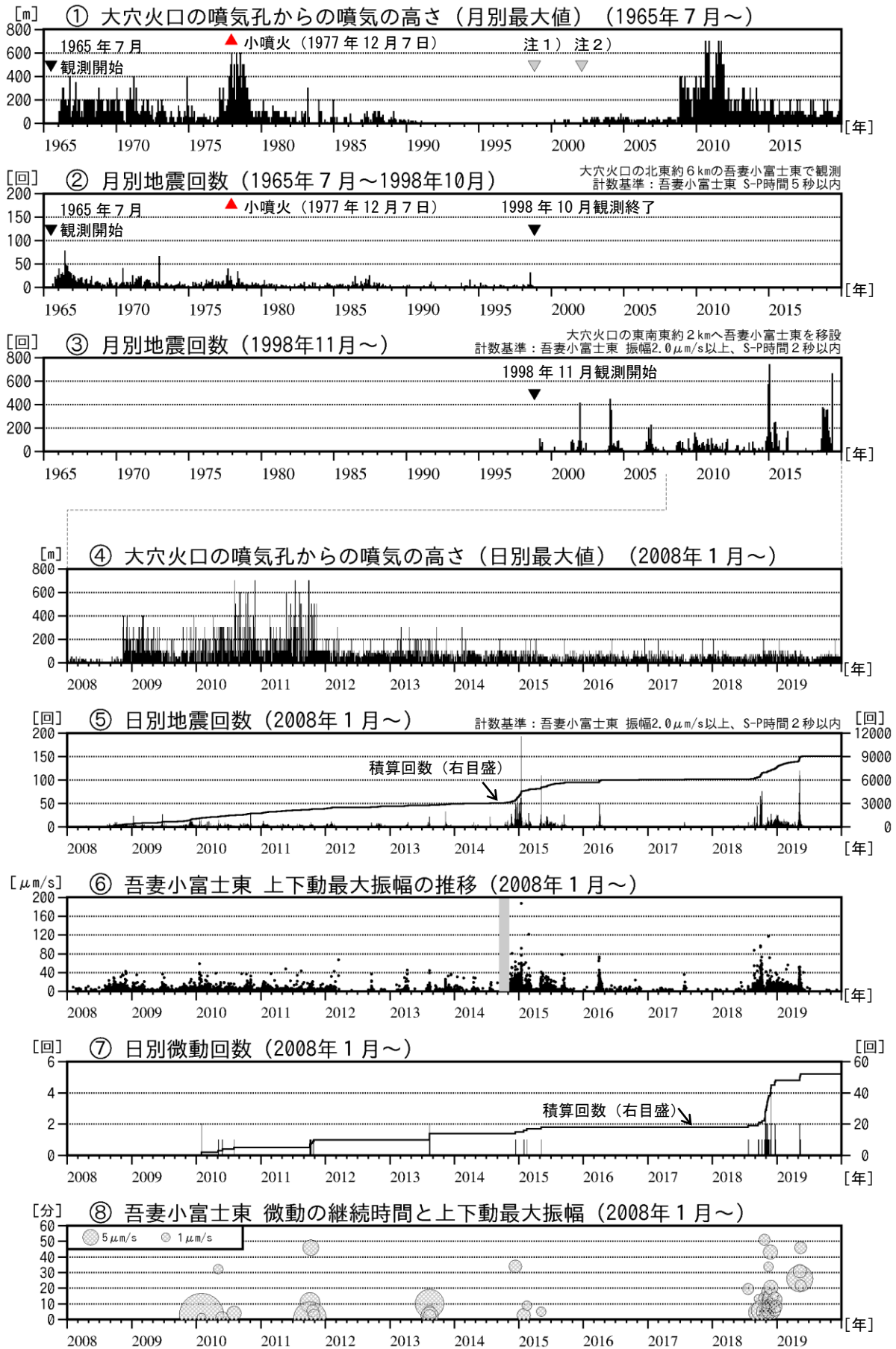
図2 吾妻山 火山活動経過図（1965年7月～2019年12月）
