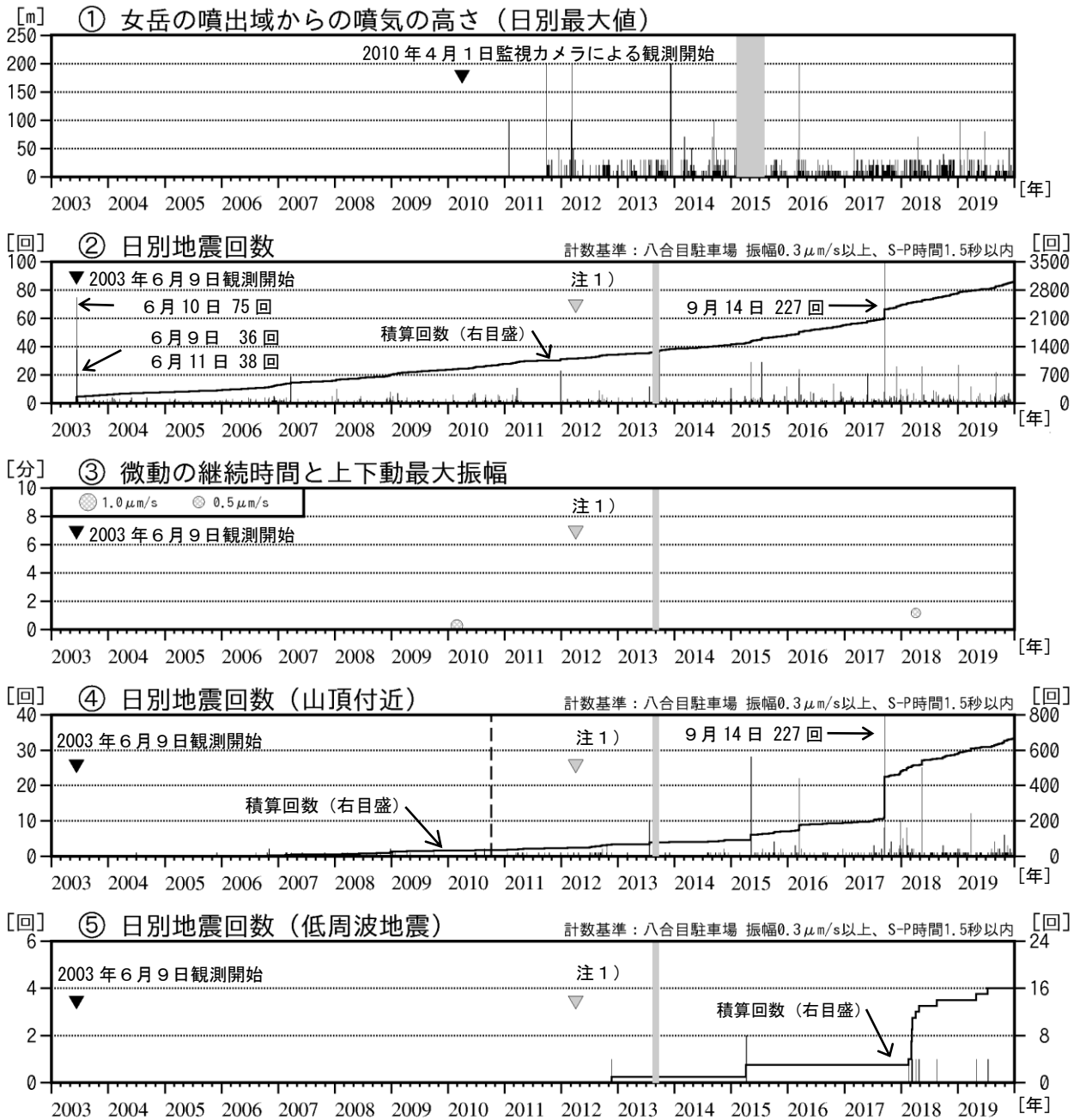
図2 秋田駒ヶ岳 火山活動経過図（2003年6月～2019年12月）
