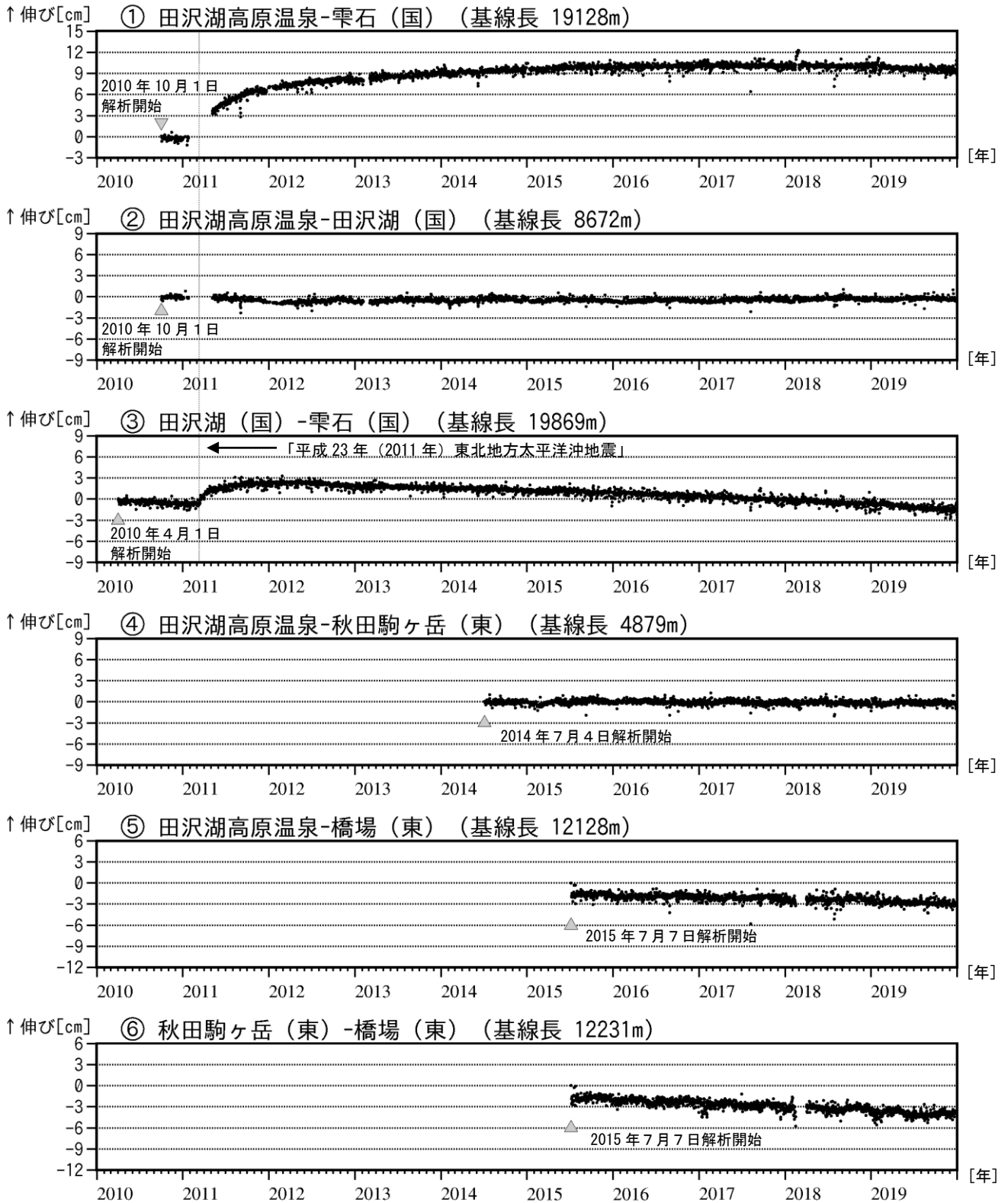
図4 秋田駒ヶ岳 GNSS 基線長変化図（2010年4月～2019年12月）
