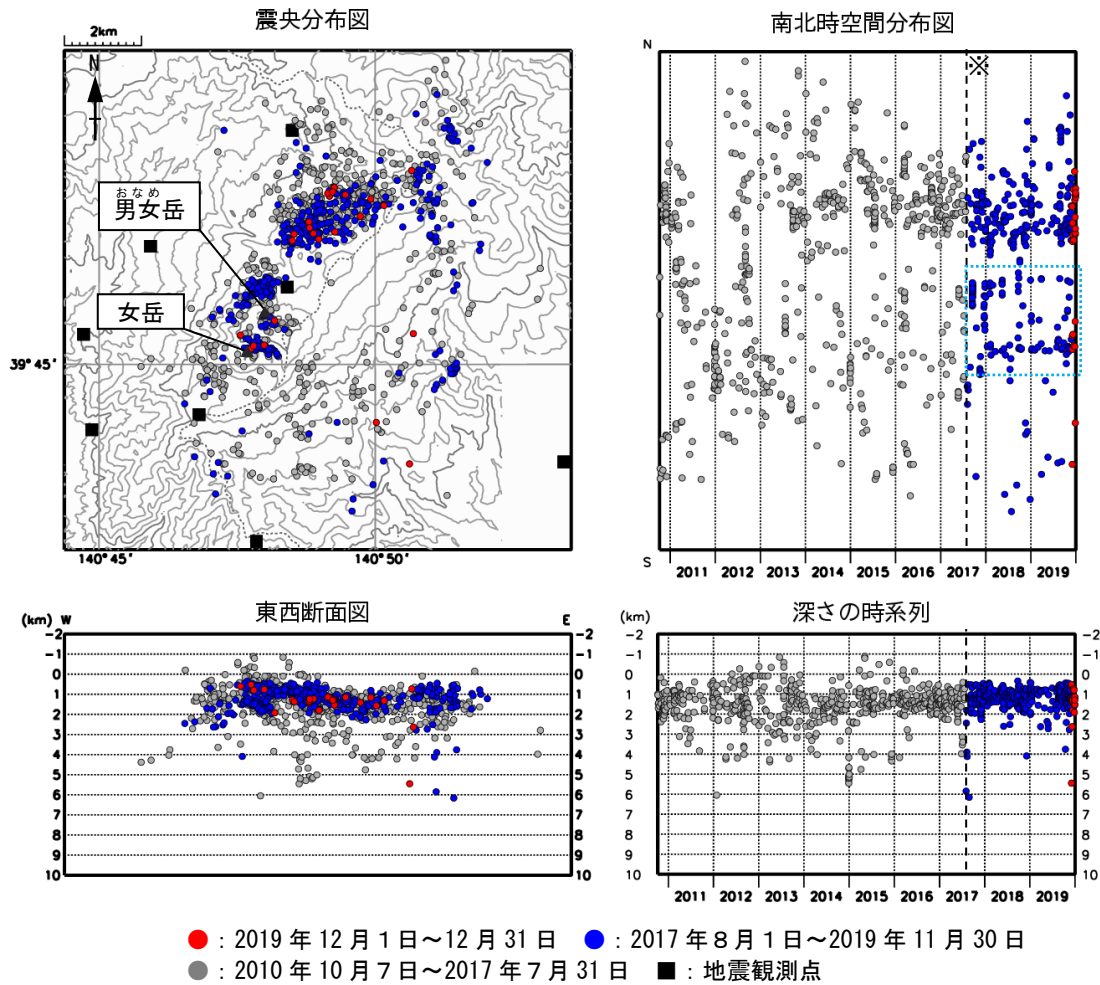
図3 秋田駒ヶ岳 地震活動（2010年10月～2019年12月）
