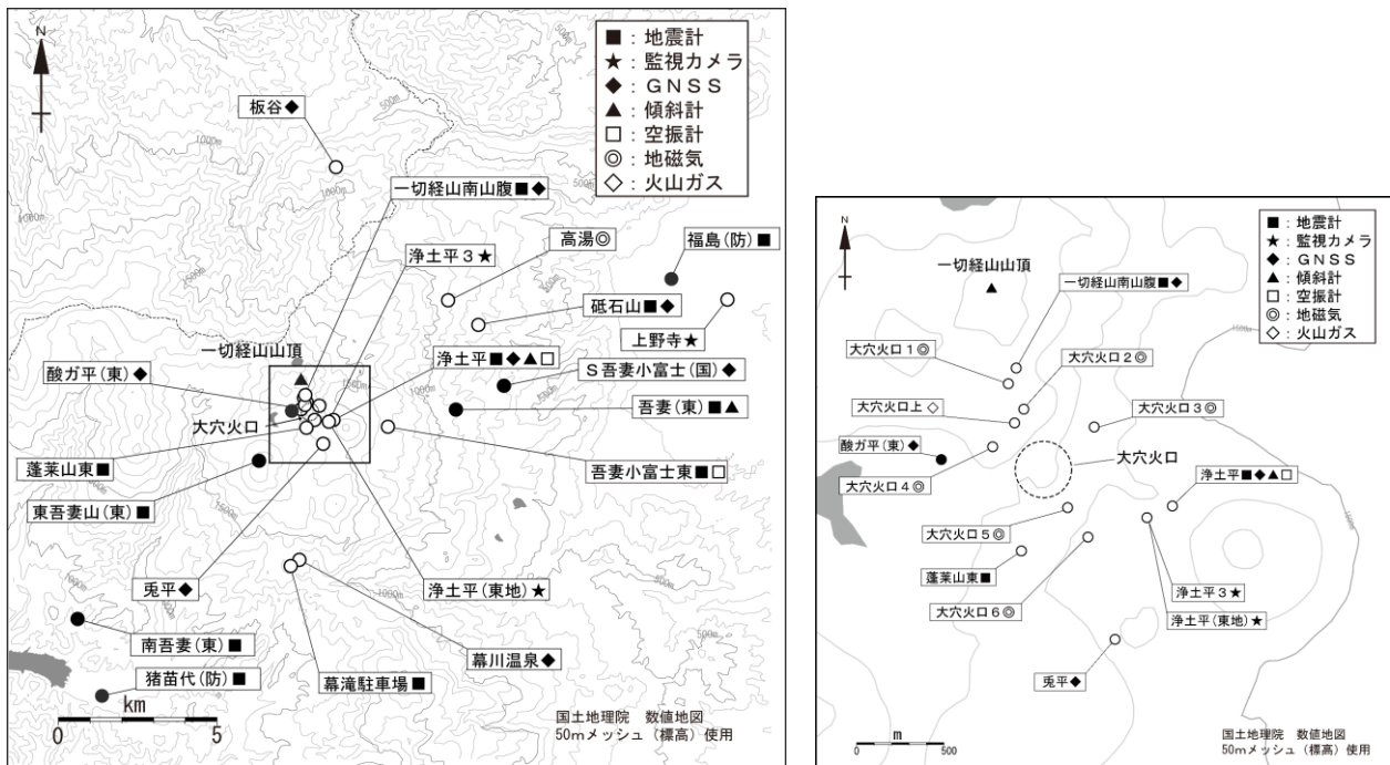
図 16 吾妻山 観測点配置図
