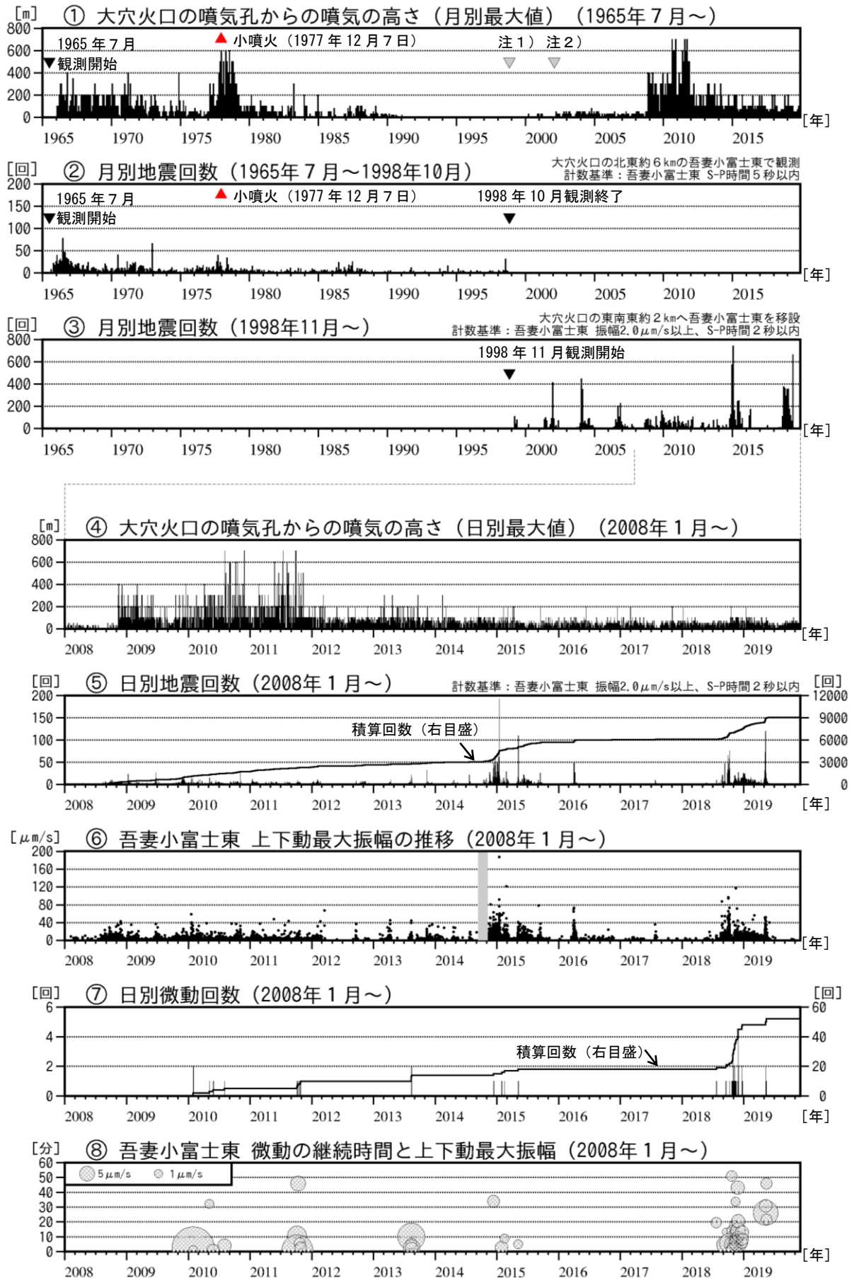
図2 吾妻山 火山活動経過図（1965年7月～2019年11月）
