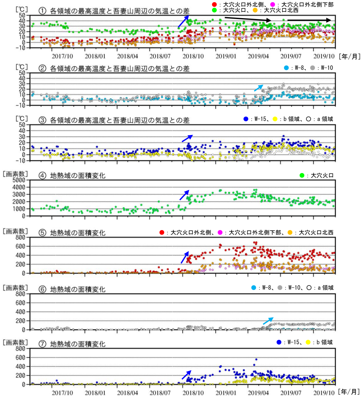
図7 吾妻山 監視カメラによる大穴火口周辺の地熱域の経過（2017年8月～2019年11月）
