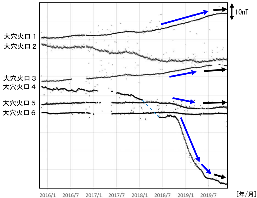
図 13 吾妻山 全磁力連続観測点の全磁力値変化（2015年11月～2019年11月）
