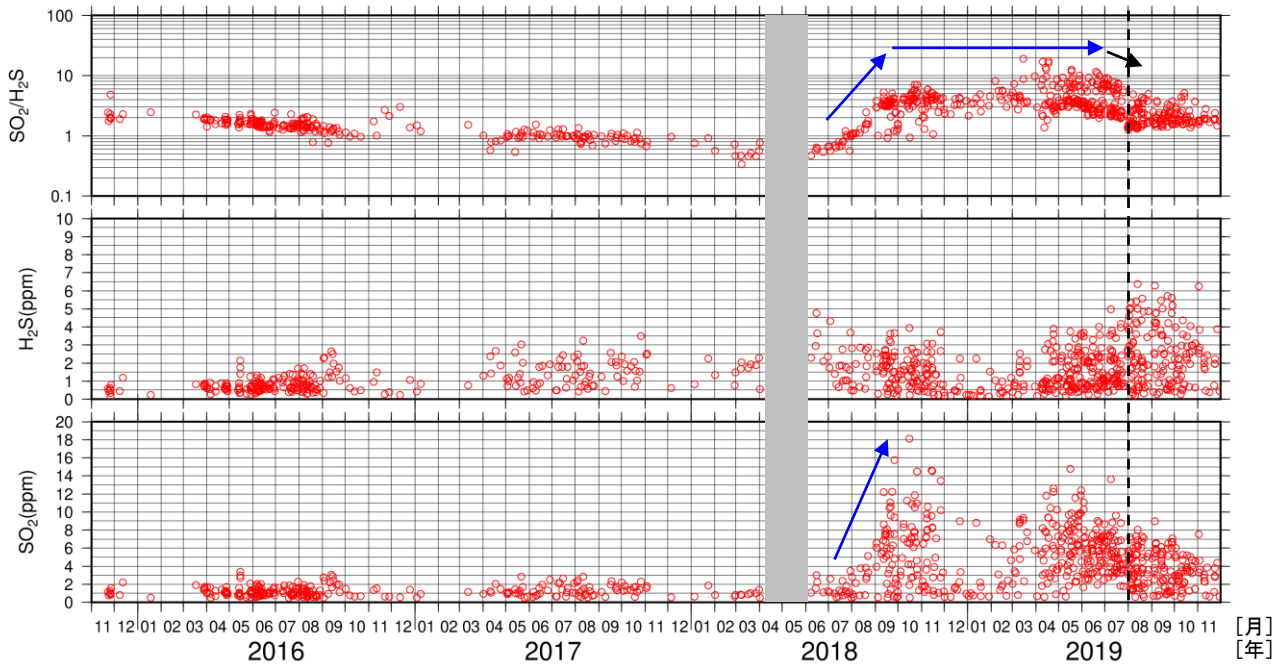
図 11 吾妻山 火山ガス観測装置による観測（2015年11月～2019年11月）
