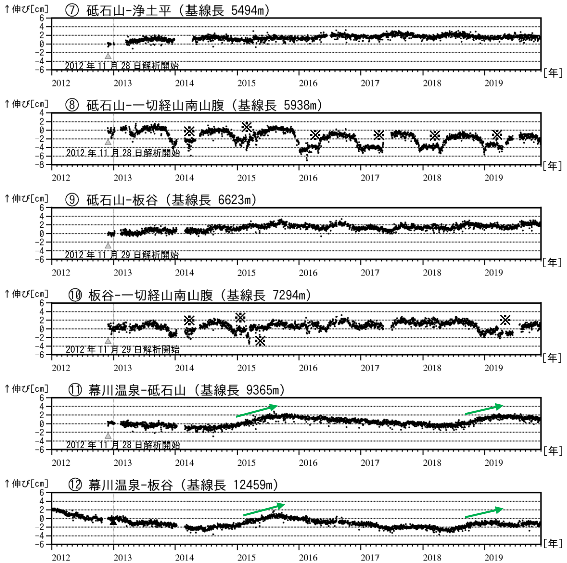
図4 吾妻山 GNSS 基線長変化図（2012年1月～2019年11月）
