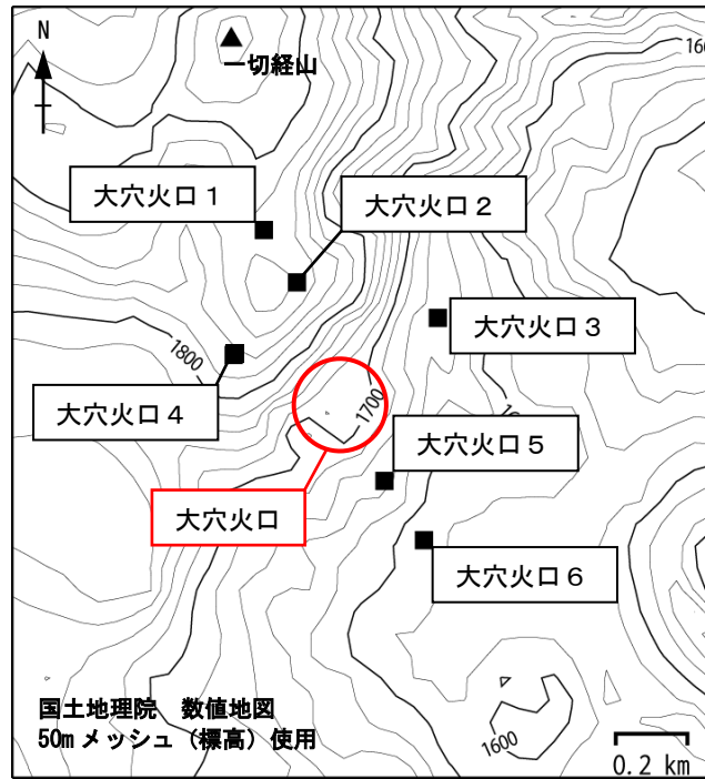
図 12 吾妻山 全磁力観測点配置図 ■ : 全磁力観測点
