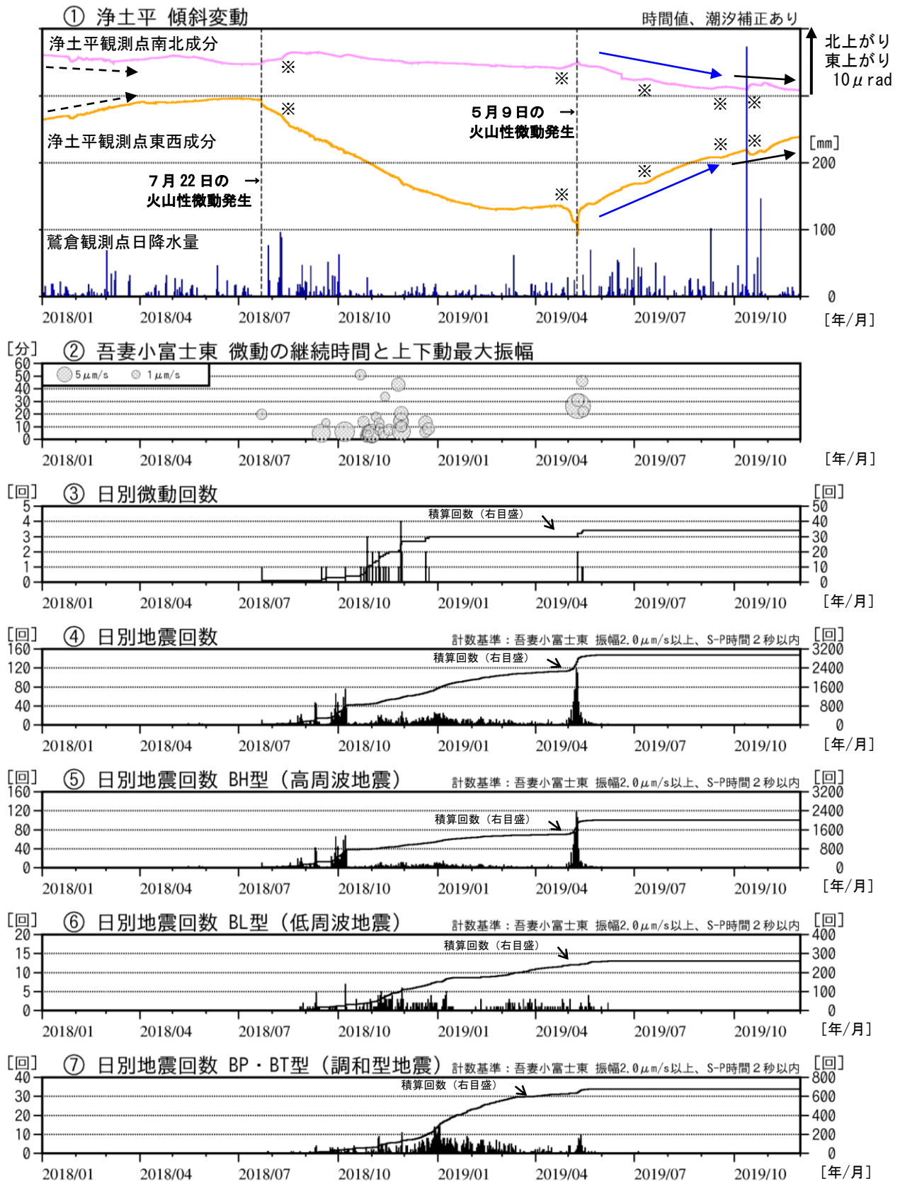
図1 吾妻山 浄土平観測点における傾斜変動、火山性微動の発生状況及び日別地震回数 (2018年1月~2019年11月)
