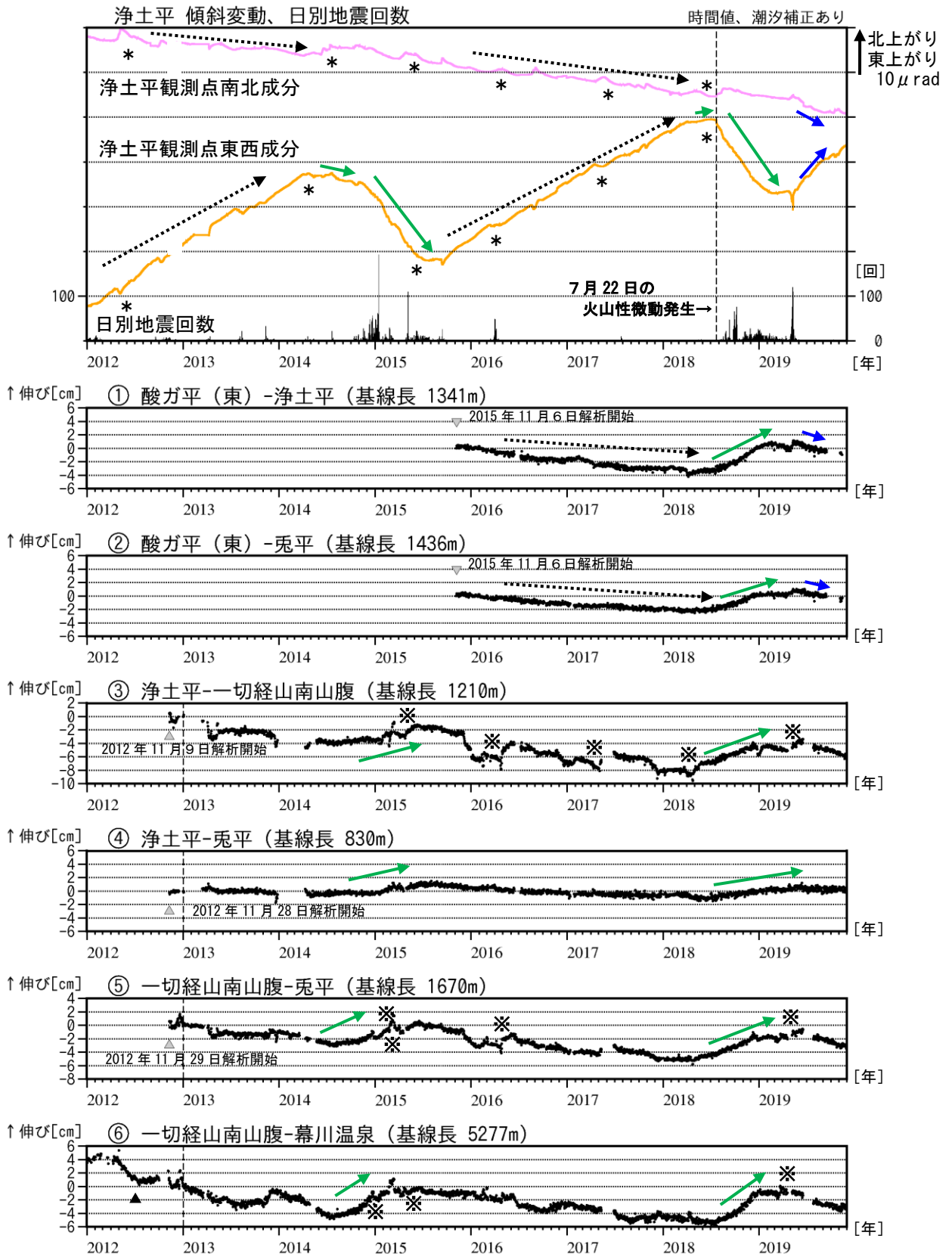
図3 吾妻山 傾斜変動及びGNSS基線長変化図（2012年1月～2019年11月）
