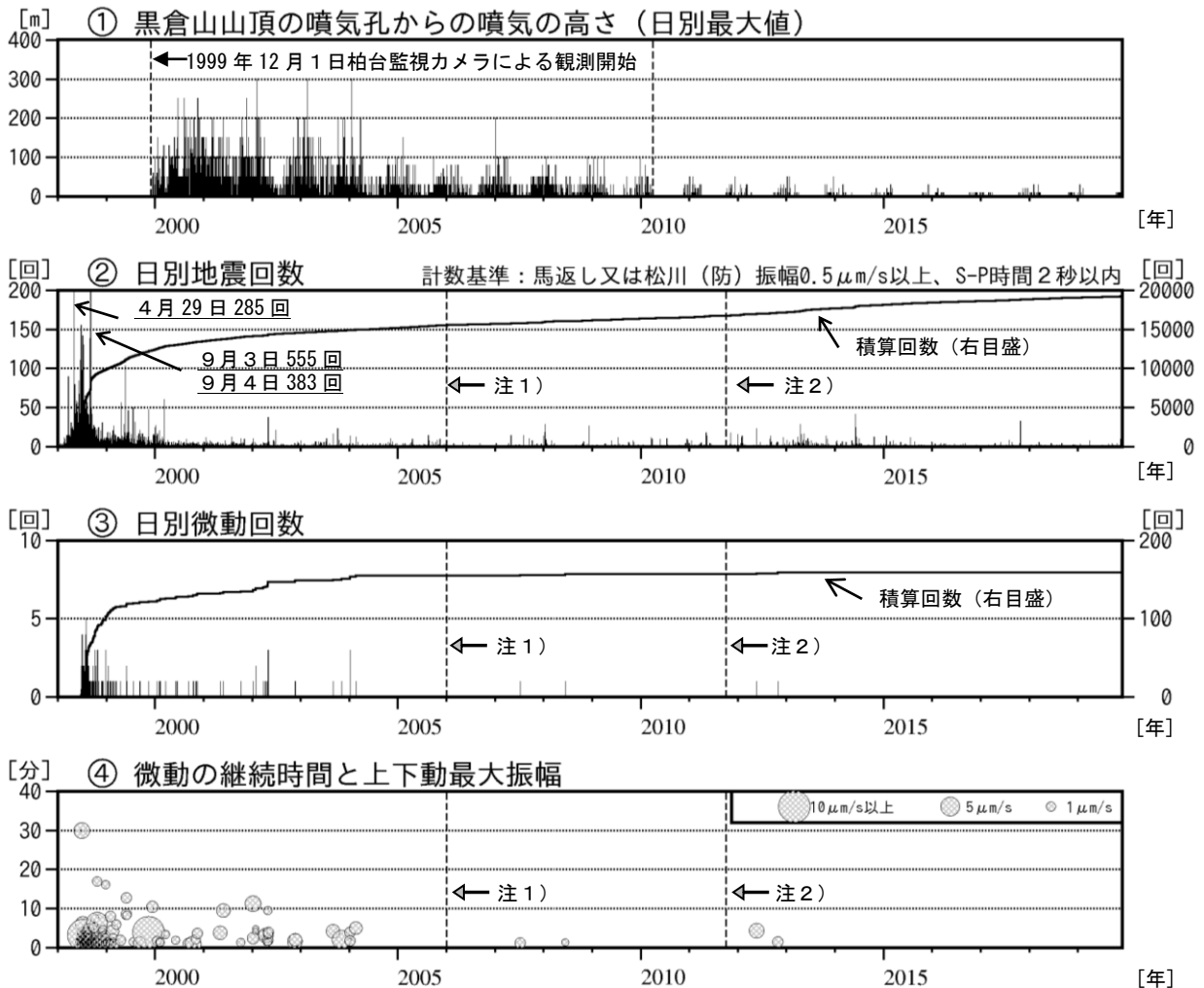
図3 岩手山 火山活動経過図（1998年1月～2019年11月） ・①2010年3月までは黒倉山のみの観測値を、2010年4月1日以降は岩手山全体の観測値を示しています。 ・②～④地震及び微動の計数基準観測点の変更は次のとおりです。 観測開始 1998年1月1日～ 東北大学松川観測点 注1) 2006年1月1日～ 焼切沢観測点 注2) 2011年10月1日～ 馬返し観測点及び防災科学技術研究所松川観測点 ・②2000年1月以降は滝ノ上付近の地震など山体以外の地震を除外した回数です。（1998年から1999年までは滝ノ上付近の地震など山体以外の地震を含みます）
