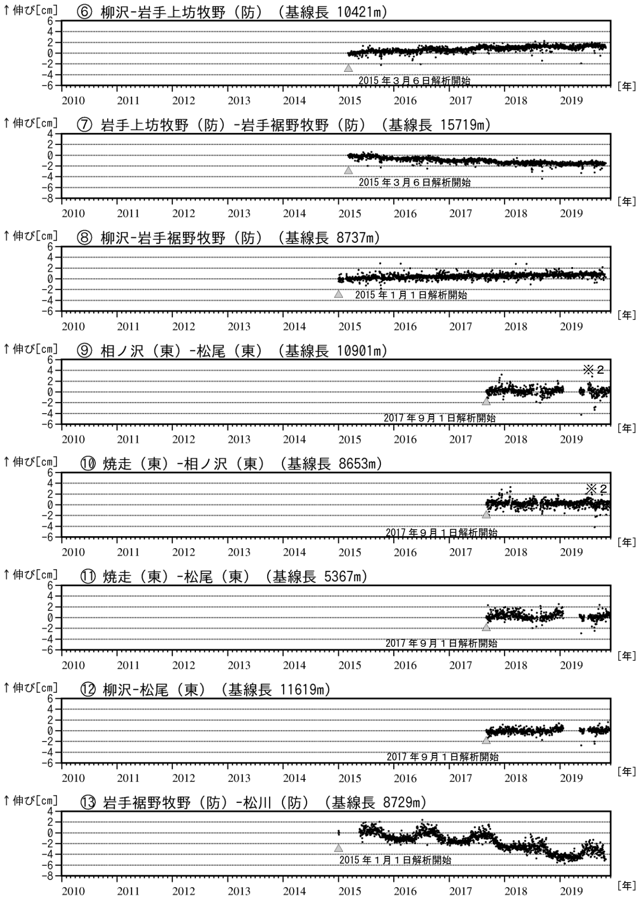
図6 岩手山 GNSS 基線長変化図（2015年1月～2019年11月）
