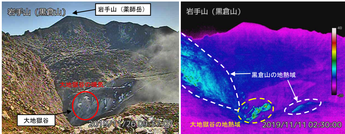
図2 岩手山 黒倉山と大地獄谷の状況（11月26日）と地表面温度分布（11月11日） ・黒倉山監視カメラ（大地獄谷の西約500m）の映像です。 ・大地獄谷で弱い噴気が認められました。 ・大地獄谷（黄破線）及び黒倉山（白破線）の地熱域に特段の変化は認められませんでした。
