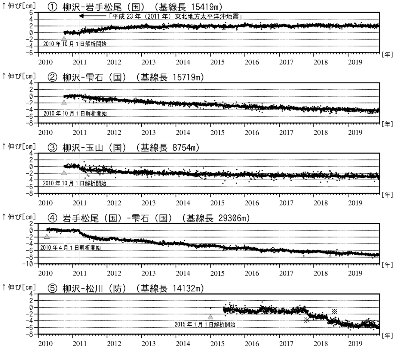
図5 岩手山 GNSS 基線長変化図（2010年4月～2019年11月）
