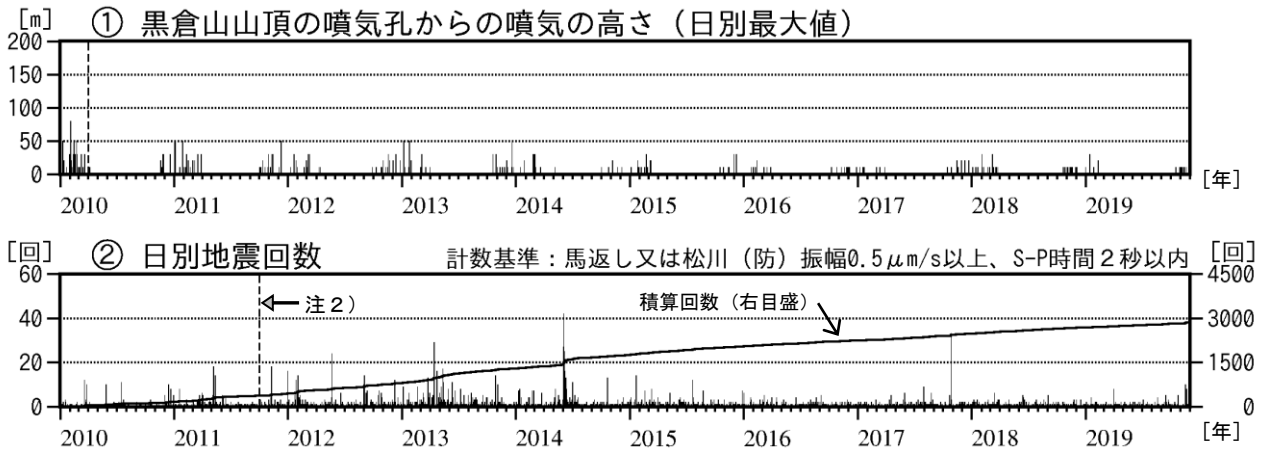
図4 岩手山 噴気の高さ及び日別地震回数（2010年1月～2019年11月）
