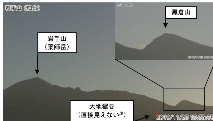
図 1 岩手山 黒倉山の噴気の状況（11 月 26 日）
