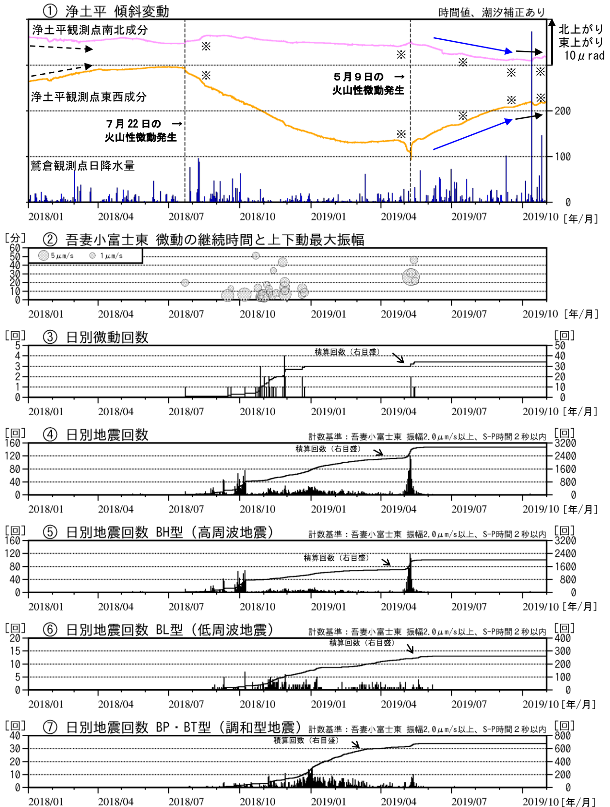
図1 吾妻山 浄土平観測点における傾斜変動、火山性微動の発生状況及び日別地震回数（2018年1月～2019年10月）
