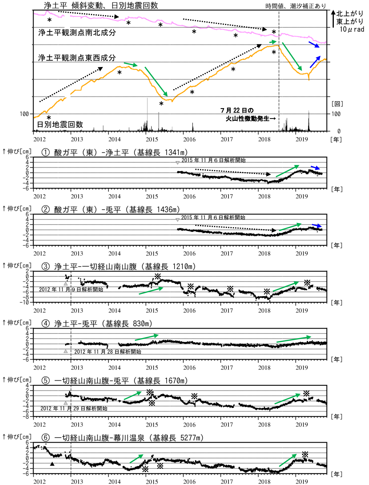
図3 吾妻山 傾斜変動及びGNSS基線長変化図（2012年1月～2019年10月）
