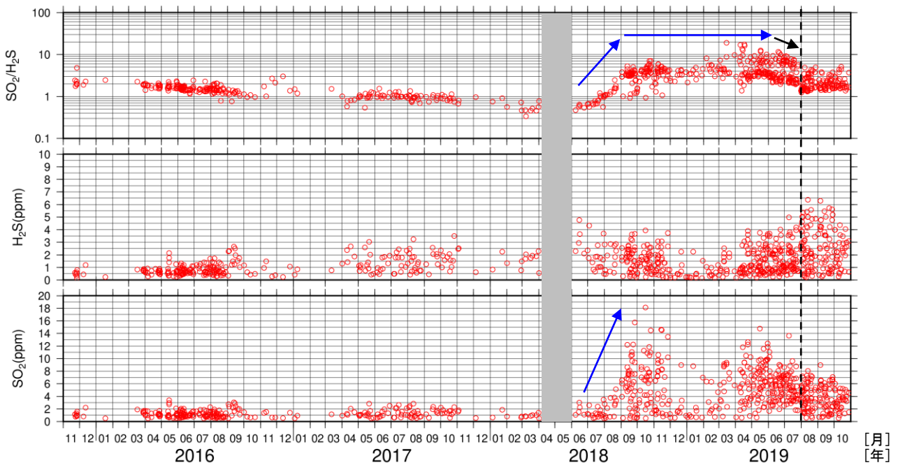
図9 吾妻山 火山ガス観測装置による観測（2015年11月～2019年10月）
