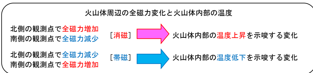
図 12 熱消磁に伴う全磁力変化のモデル
