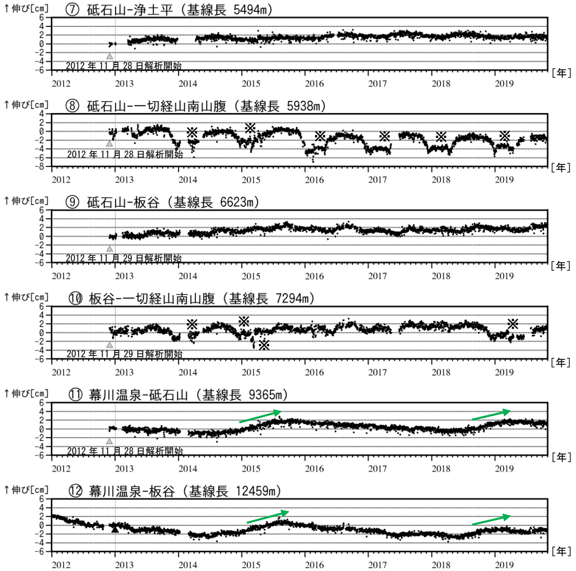
図4 吾妻山 GNSS 基線長変化図（2012年1月～2019年10月）
