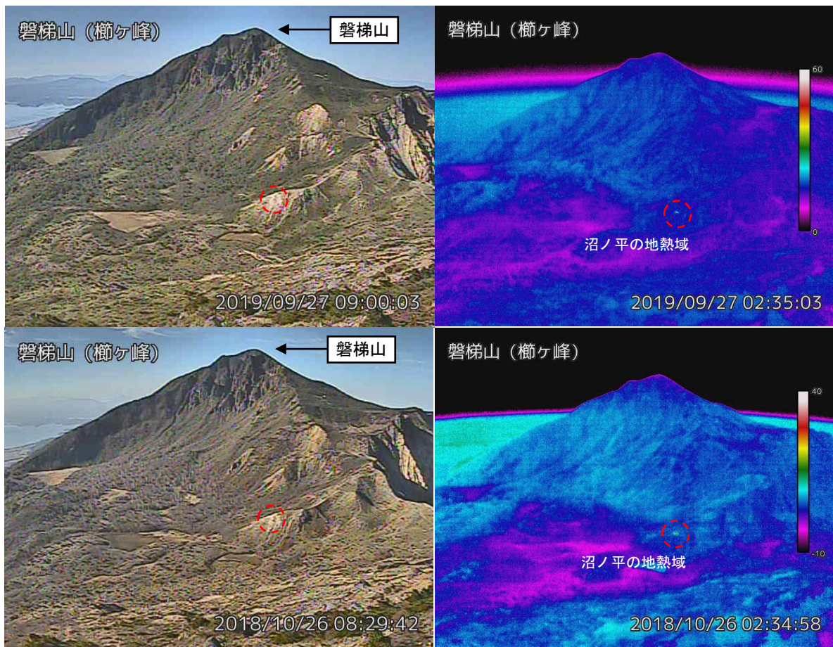
図2 磐梯山 沼ノ平周辺の状況と地表面温度分布（櫛ヶ峰監視カメラによる）
