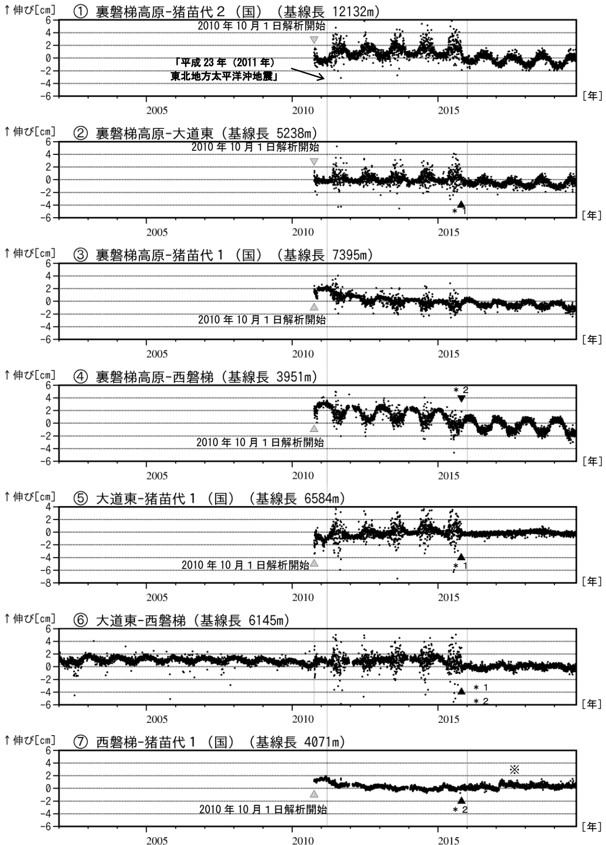
図4 磐梯山 GNSS 基線長変化図（2002年1月～2019年9月）
