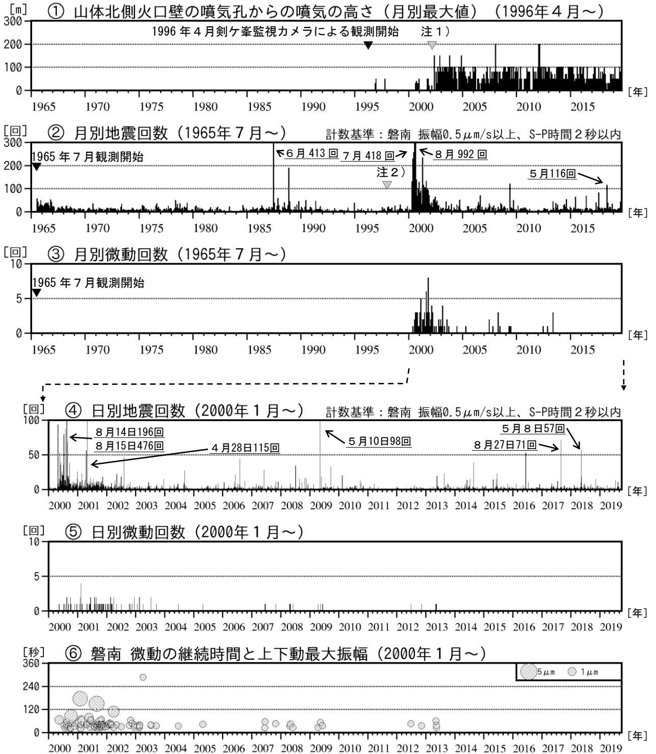
図3 磐梯山 火山活動経過図（1965年7月～2019年9月）
