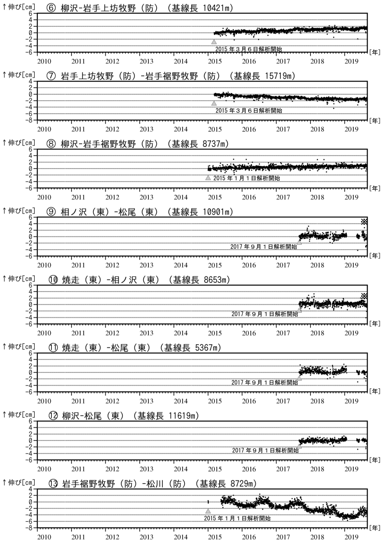
図6 岩手山 GNSS 基線長変化図（2015年1月～2019年8月）
