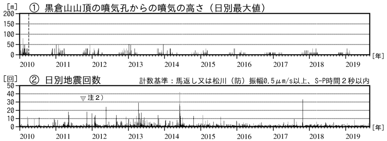
図4 岩手山 噴気の高さ及び日別地震回数（2010年1月～2019年8月）
