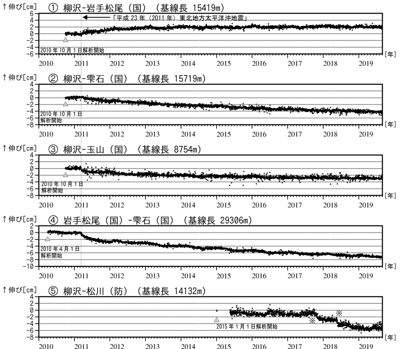
図5 岩手山 GNSS 基線長変化図（2010年4月～2019年8月）
