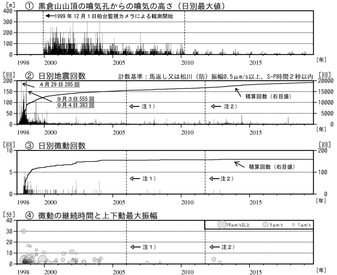
図3 岩手山 火山活動経過図（1998年1月～2019年8月）
