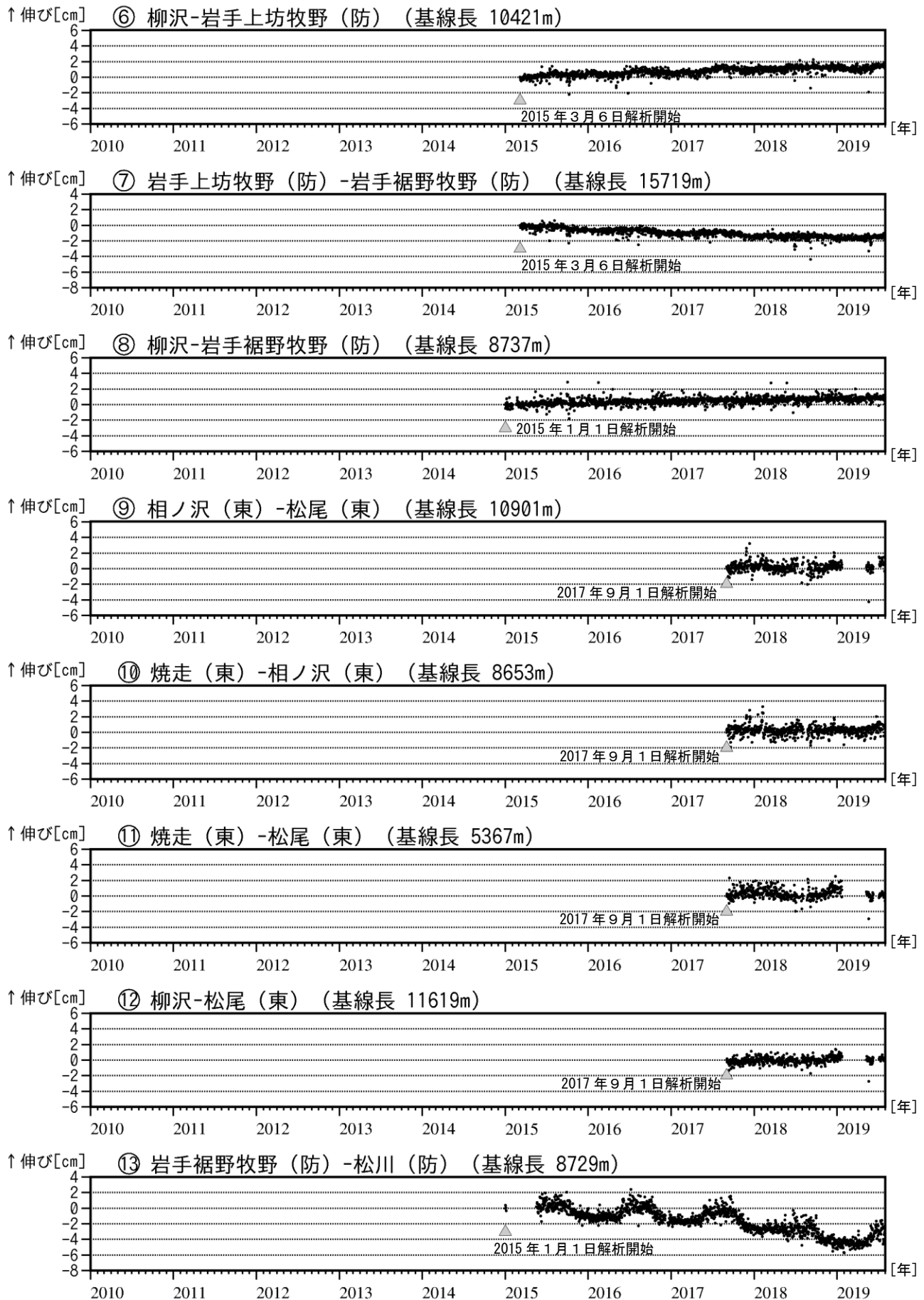
図 6 岩手山 GNSS 基線長変化図（2015 年 1 月～2019 年 7 月）
