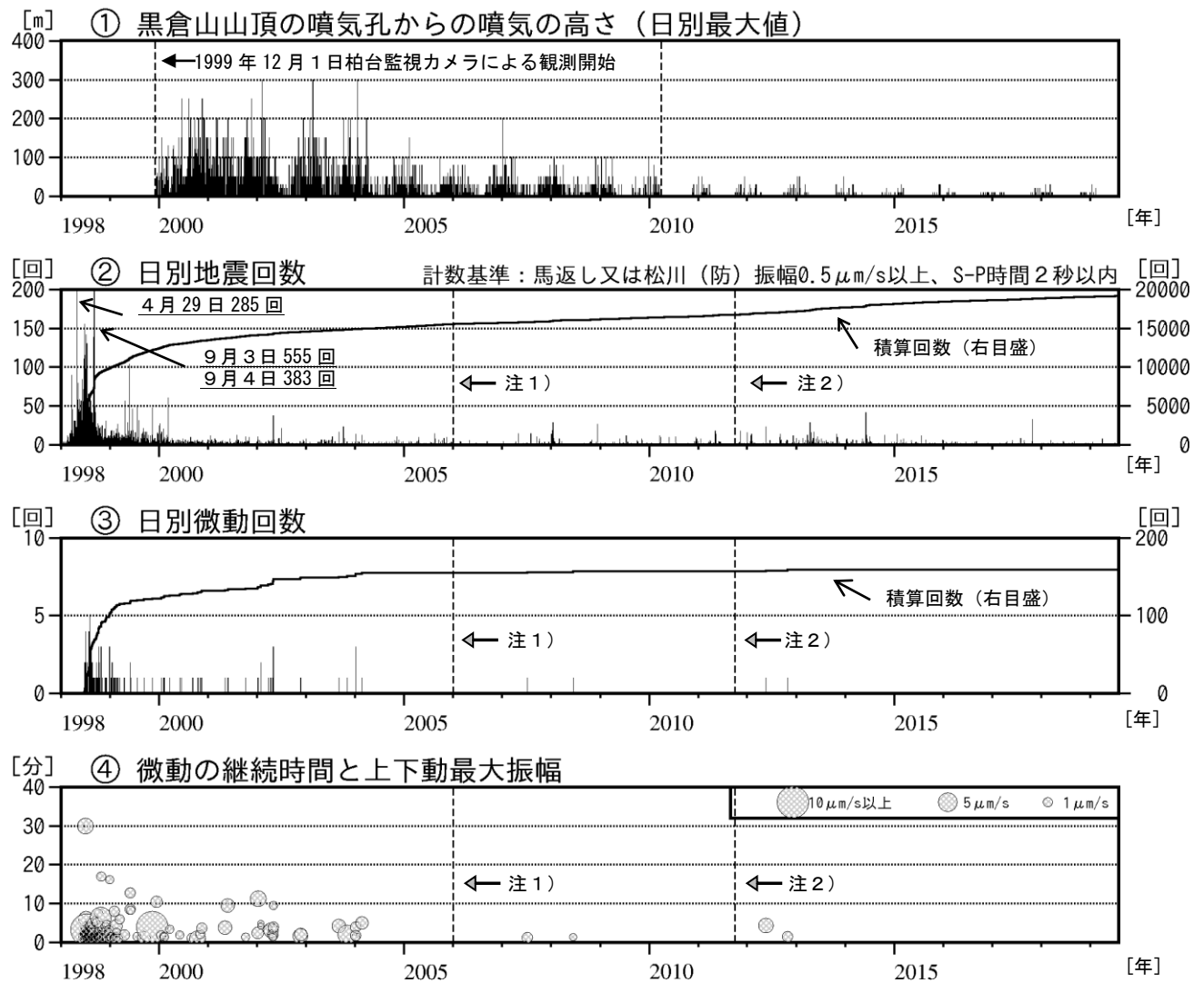
図 3 岩手山 火山活動経過図（1998 年 1 月～2019 年 7 月）
