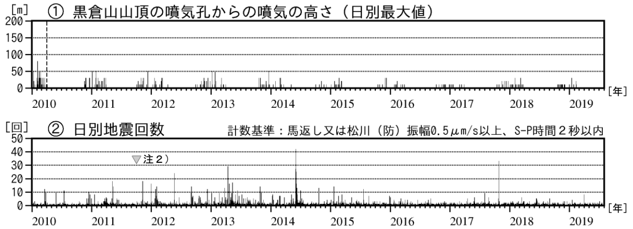
図4 岩手山 噴気の高さ及び日別地震回数（2010年1月～2019年7月）
