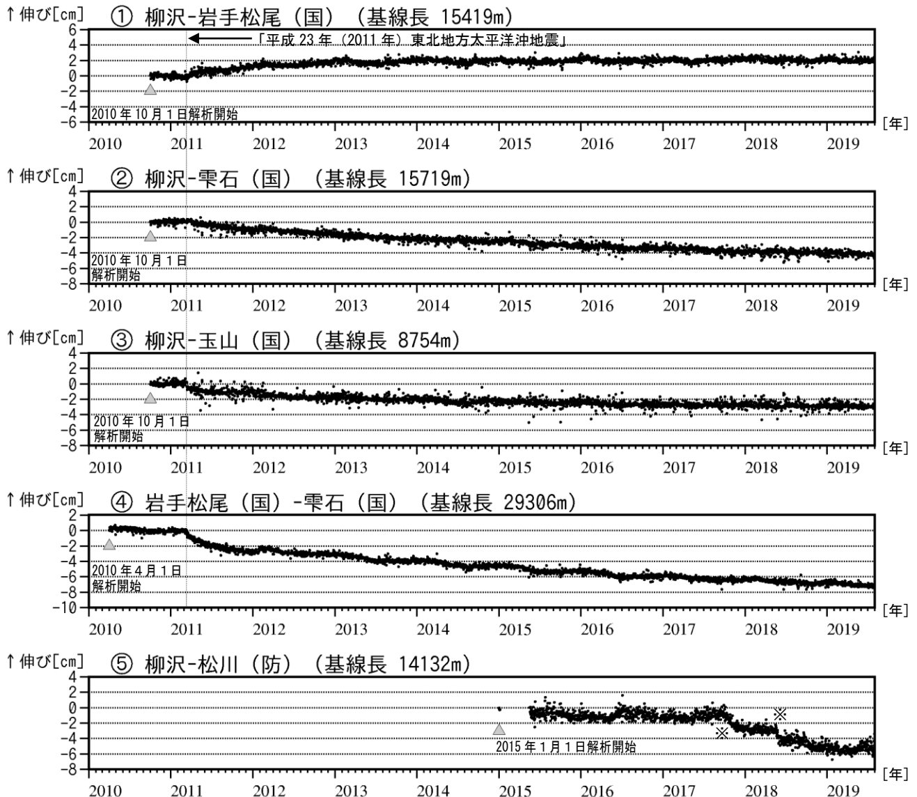
図5 岩手山 GNSS 基線長変化図（2010年4月～2019年7月）
