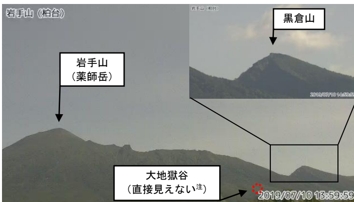
図1 岩手山 黒倉山の噴気の状況 （7月10日）
