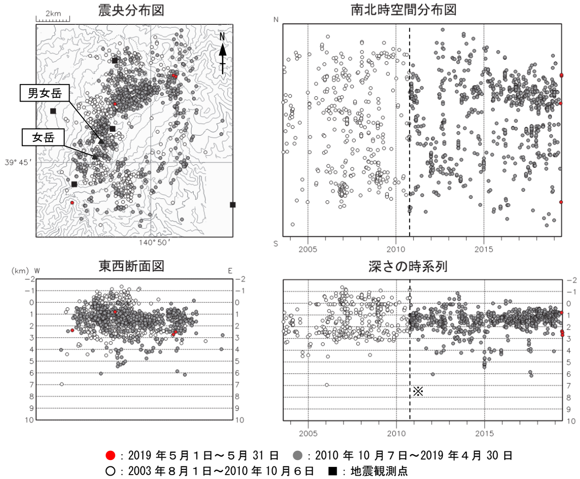
図7 秋田駒ヶ岳 地震活動（2003年8月～2019年5月）
