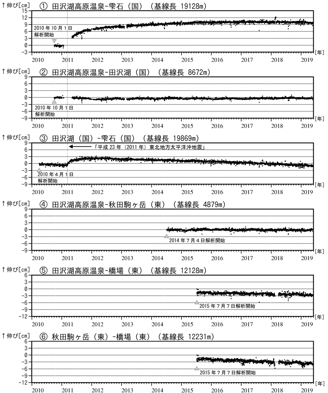
図8 秋田駒ヶ岳 GNSS 基線長変化図（2010年4月～2019年5月）
