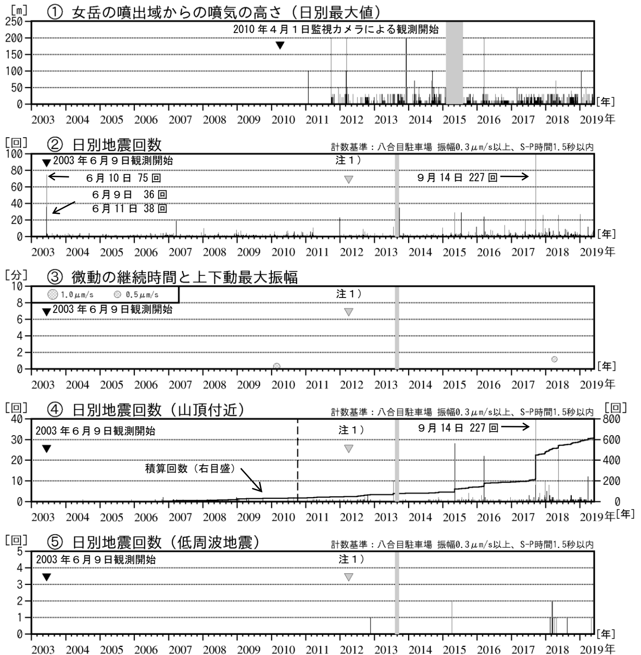
図6 秋田駒ヶ岳 火山活動経過図（2003年6月～2019年5月）
