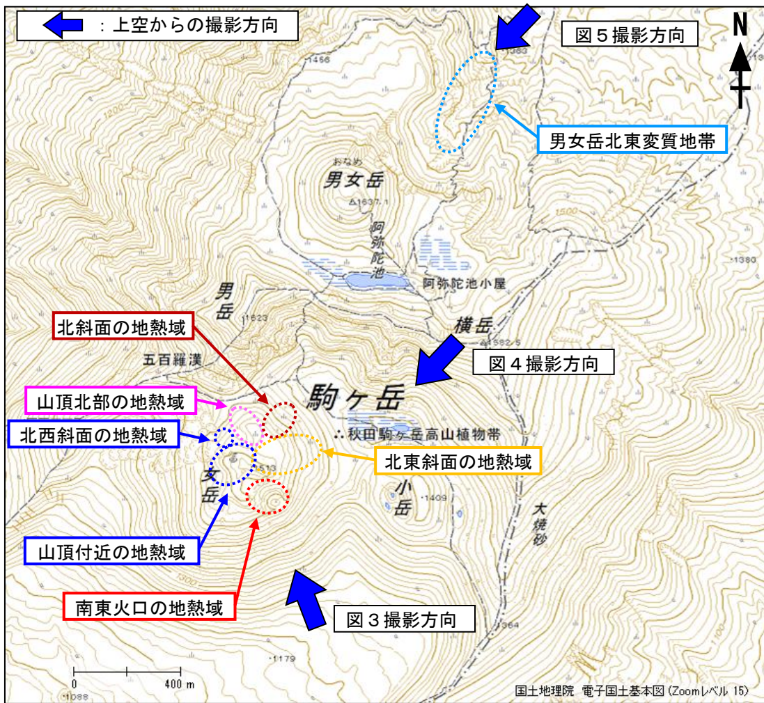
図2 秋田駒ヶ岳 女岳の地熱域の分布及び上空からの写真の撮影方向
