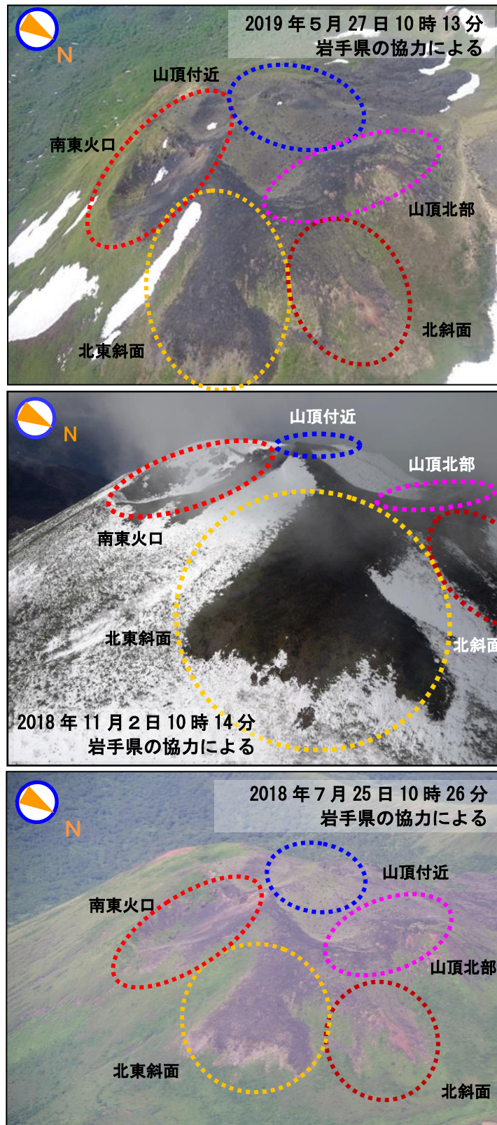
図4 秋田駒ヶ岳 上空から撮影した女岳南東火口、北東斜面、北斜面、山頂北部及び山頂付近の状況
