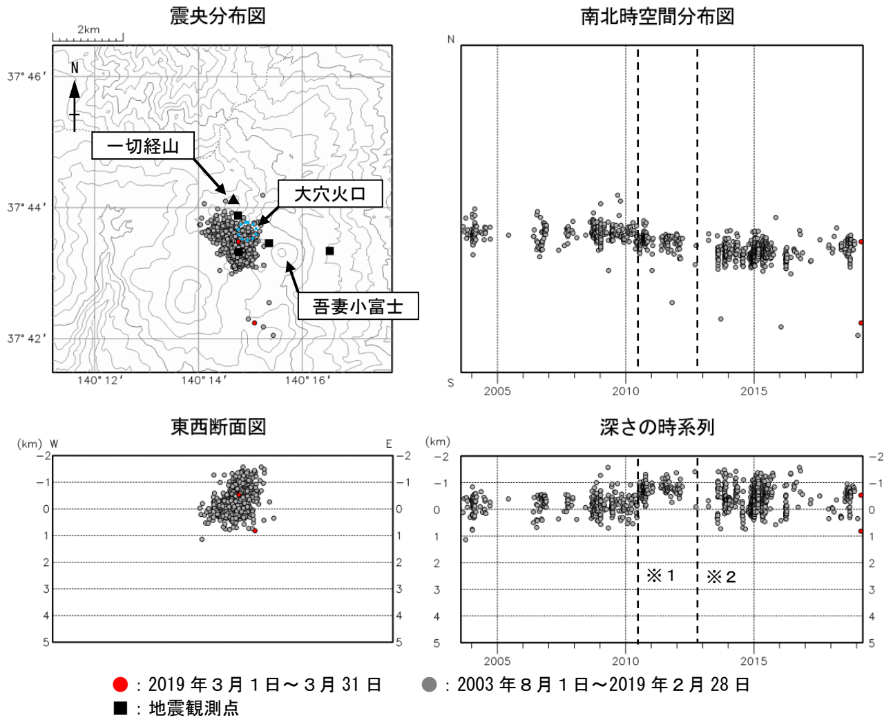
図 4 吾妻山 地震活動（2003 年 8 月～2019 年 3 月）
