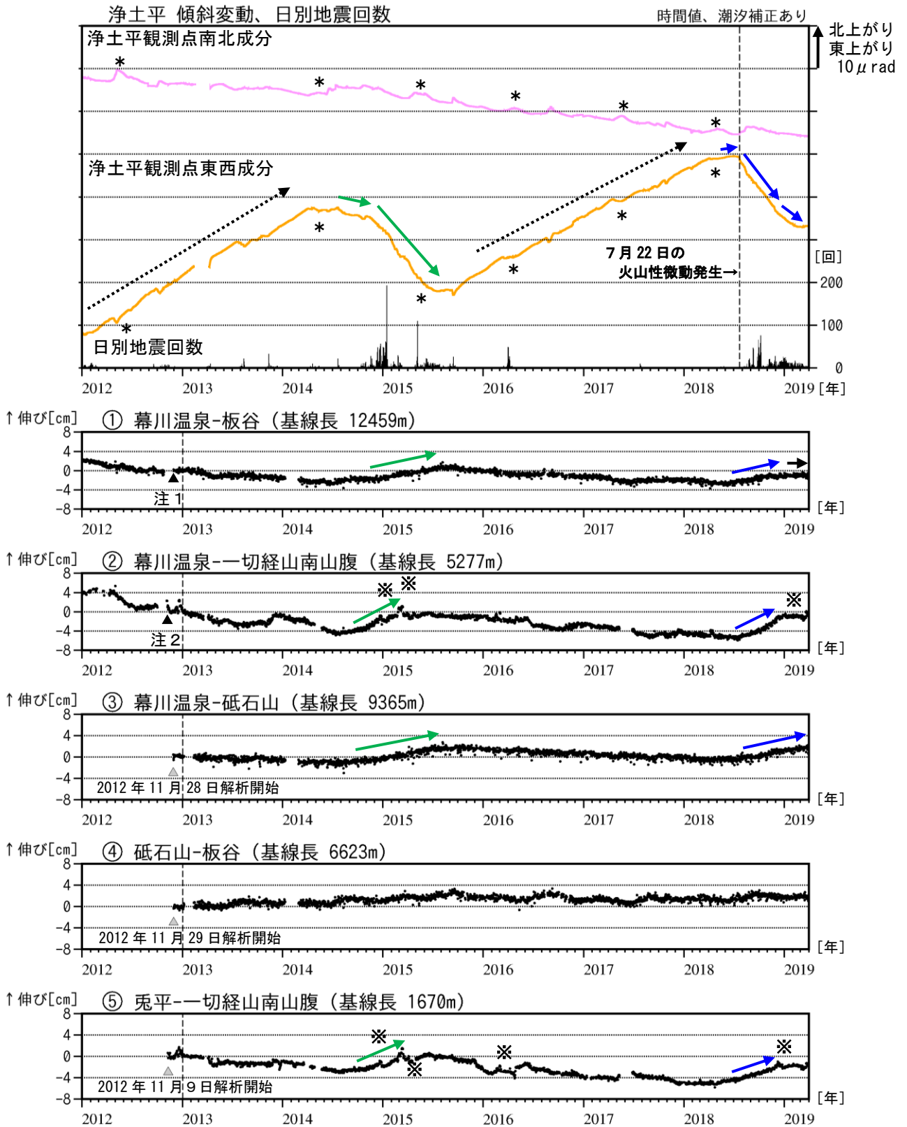
図5 吾妻山 傾斜変動及びGNSS基線長変化図（2012年1月～2019年3月）
