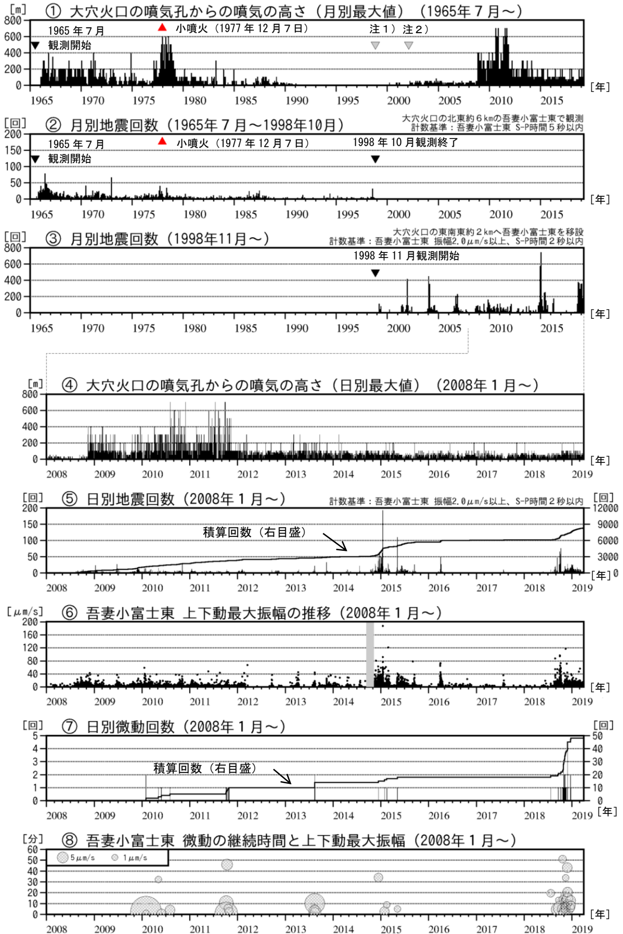
図3 吾妻山 火山活動経過図 (1965年7月～2019年3月)
