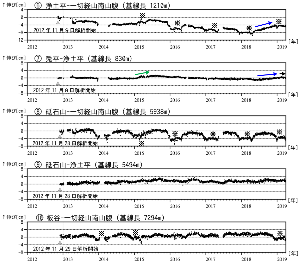
図6 吾妻山 GNSS 基線長変化図 (2012 年 1 月～2019 年 3 月)
