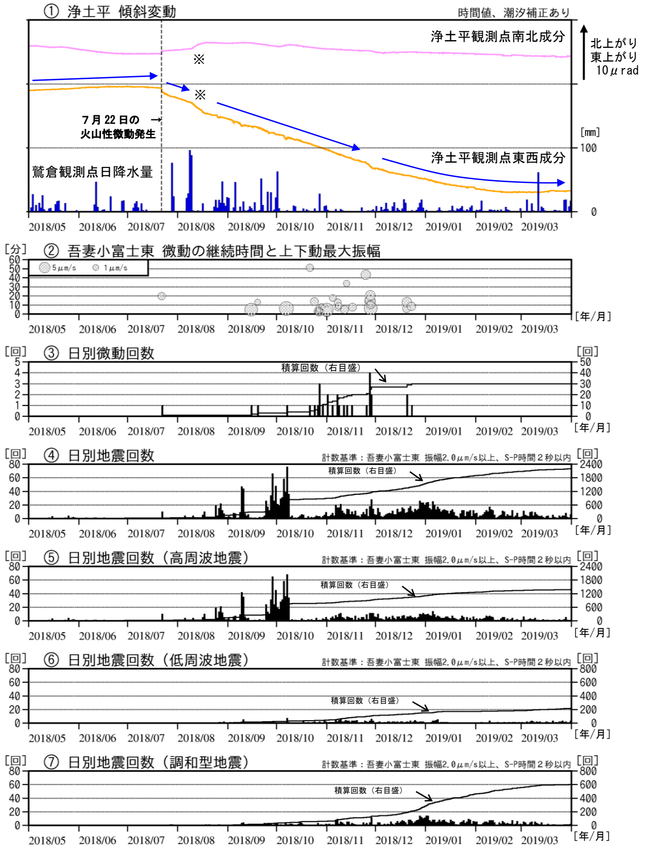
図2 吾妻山 浄土平観測点における傾斜変動、火山性微動の発生状況及び日別地震回数 (2018年5月~2019年3月)
