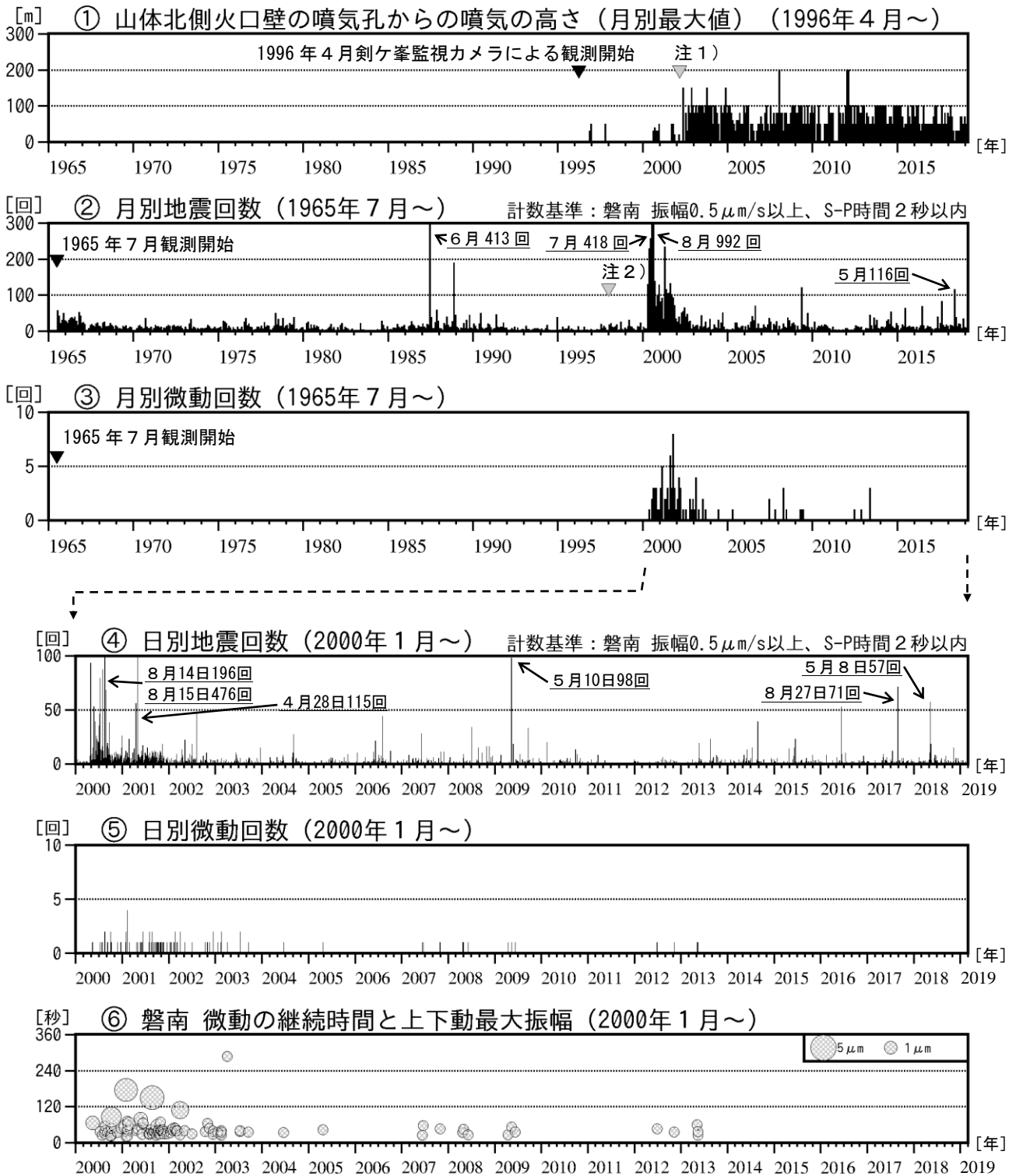
図7 磐梯山 火山活動経過図（1965年7月～2019年2月）
