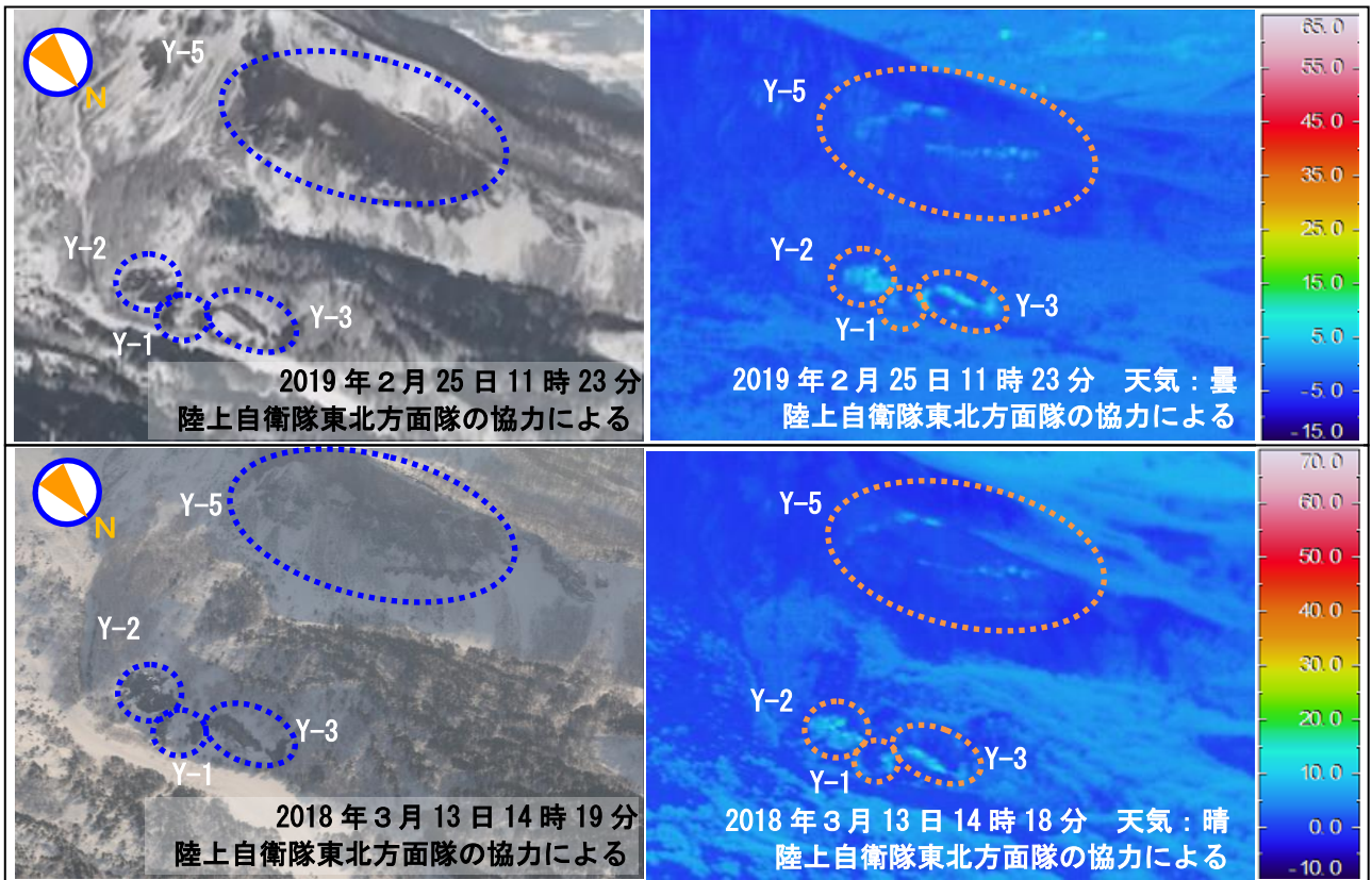
図5 磐梯山 上空から撮影した火口壁噴気地帯（Y-1、2、3、5）の状況と地表面温度分布 ・噴気及び地熱域の状況に特段の変化は認められませんでした。 ※地熱域以外の温度の高い部分は日射による影響と推定されます。
