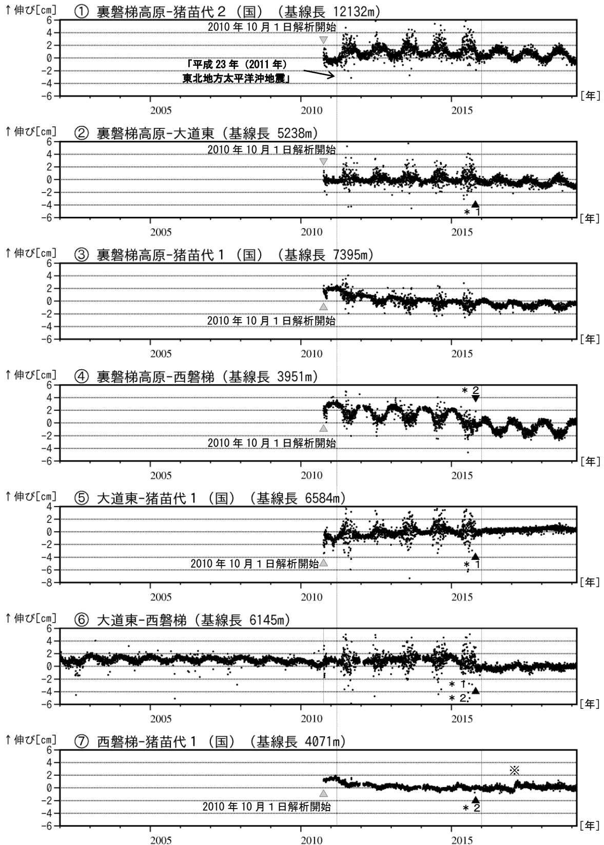
図 8 磐梯山 GNSS 基線長変化図 (2002 年 1 月～2019 年 2 月)
