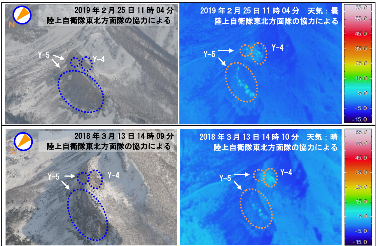
図6 磐梯山 上空から撮影した火口壁噴気地帯（Y-4、5）の状況と地表面温度分布 ・噴気は確認されず、地熱域（破線）の状況に特段の変化は認められませんでした。 ※地熱域以外の温度の高い部分は日射による影響と推定されます。
