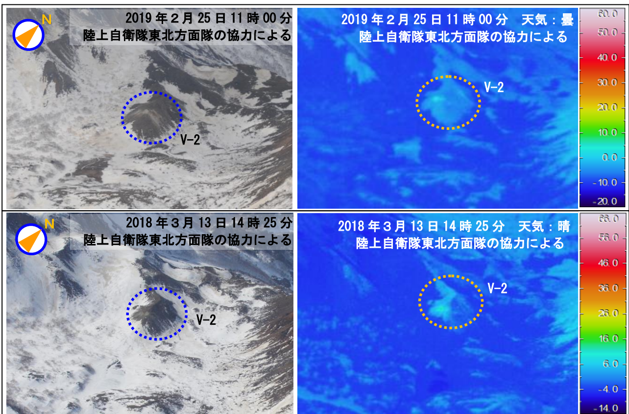
図 4 磐梯山 上空から撮影した沼ノ平噴気地帯 (V-2) の状況と地表面温度分布 ・噴気は確認されず、地熱域（破線）の状況に特段の変化は認められませんでした。 ※地熱域以外の温度の高い部分は日射による影響と推定されます。
