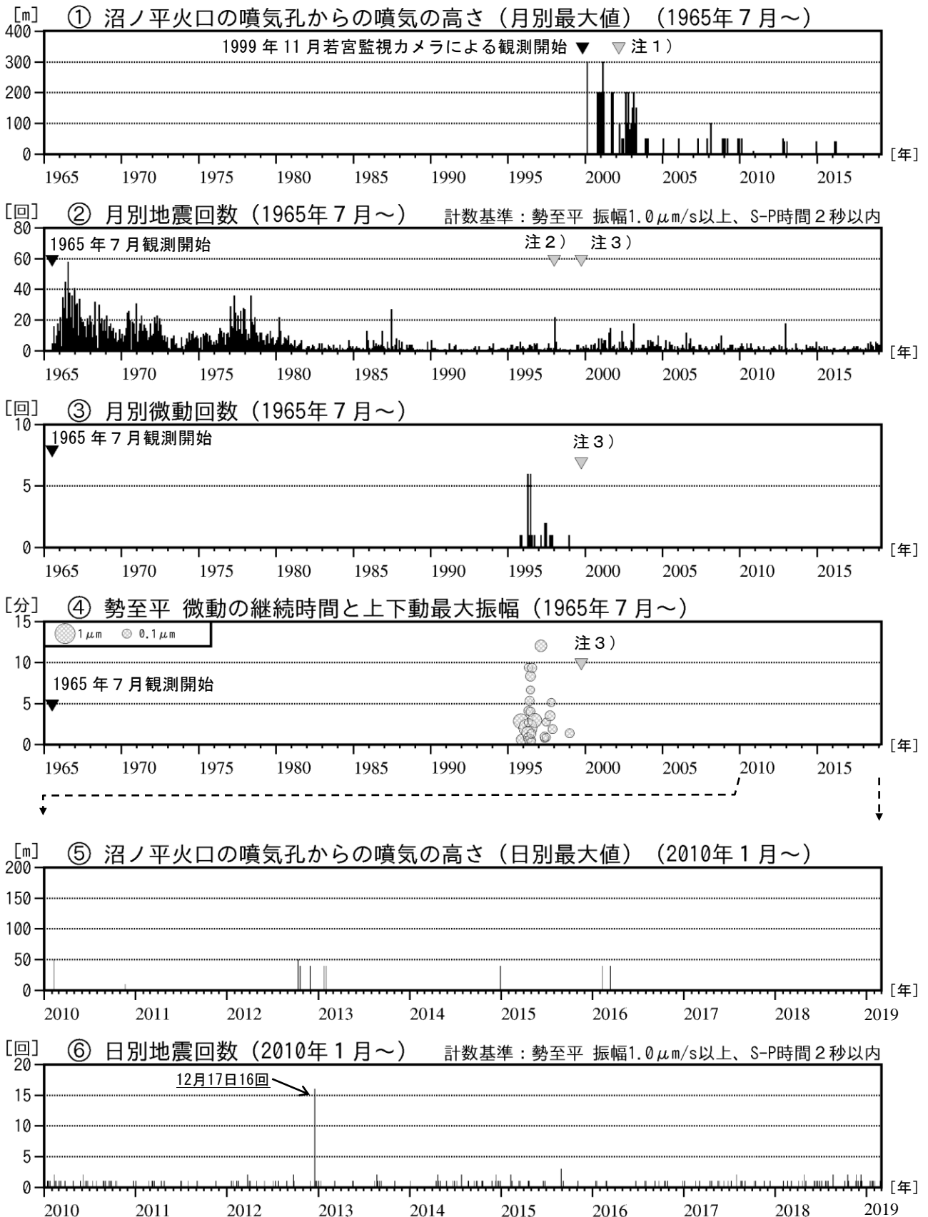
図4 安達太良山 火山活動経過図（1965年7月～2019年2月）
