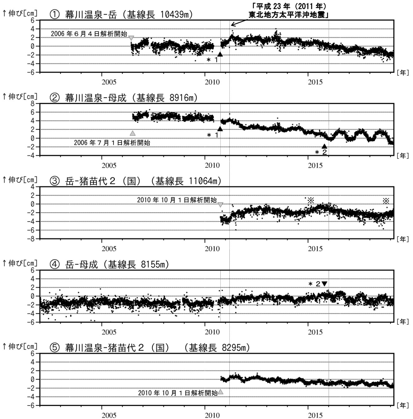
図5 安達太良山 GNSS 基線長変化図（2002年1月～2019年2月）
