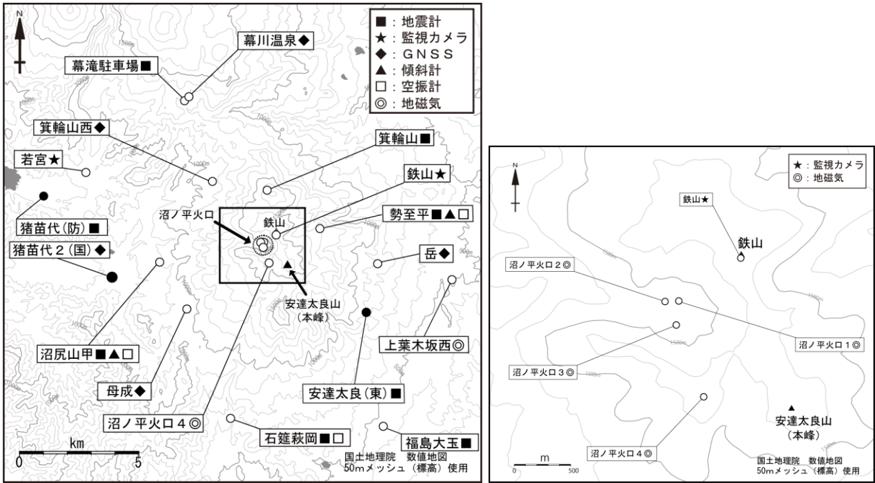
図6 安達太良山 観測点配置図
