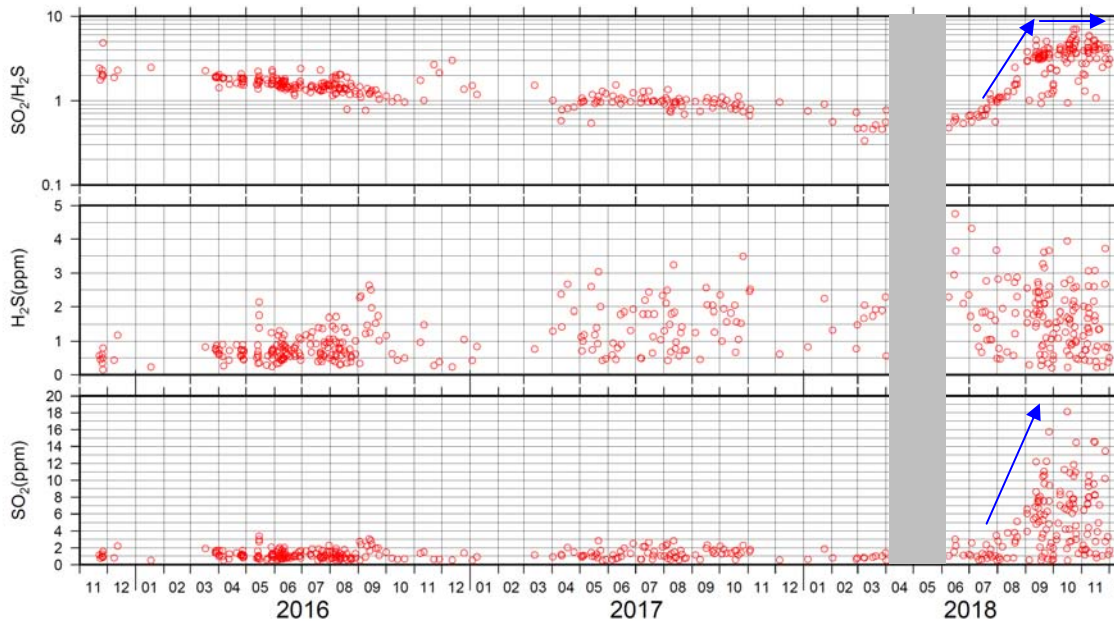
図9 吾妻山 火山ガス観測装置による観測（2015年11月～2018年11月）
