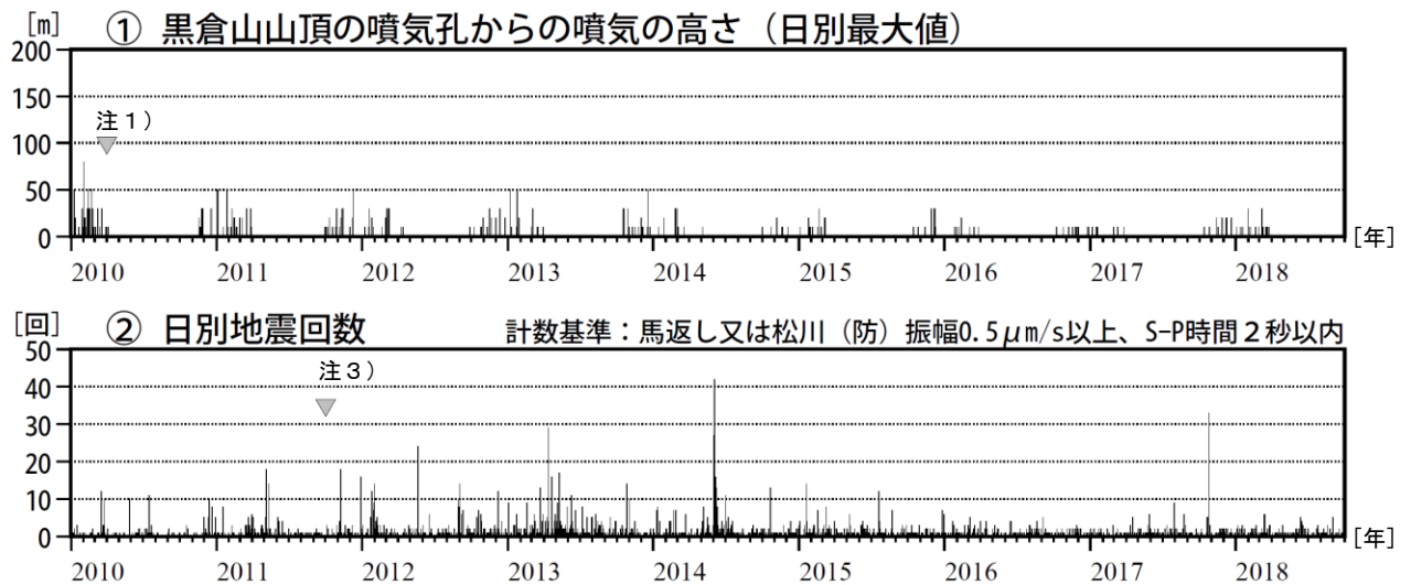
図4 岩手山 噴気の高さ及び日別地震回数（2010年1月～2018年9月）
