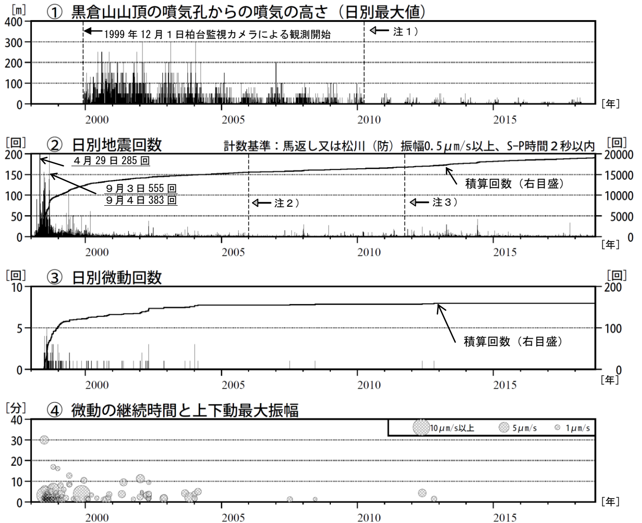
図 3 岩手山 火山活動経過図（1998 年 1 月～2018 年 9 月）
