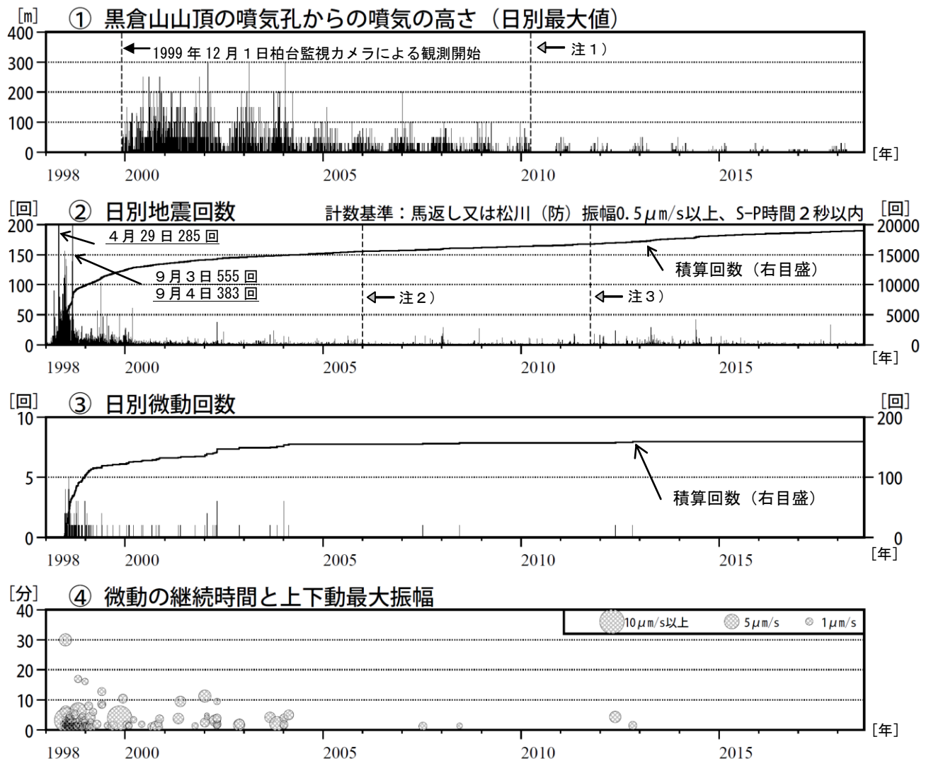
図 3 岩手山 火山活動経過図（1998 年 1 月～2018 年 8 月）
