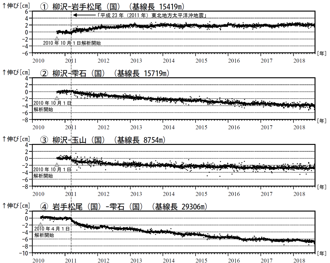
図 5 岩手山 GNSS 1) 基線長変化図（2010 年 4 月～2018 年 8 月）
