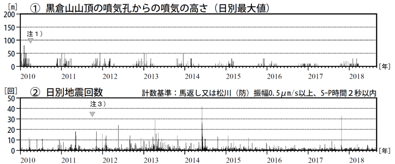
図 4 岩手山 噴気の高さ及び日別地震回数（2010 年 1 月～2018 年 8 月）
