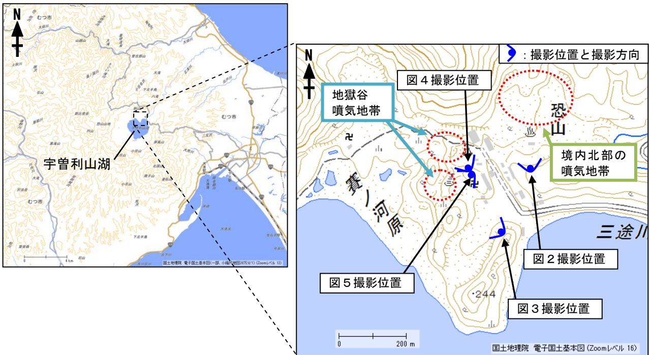
図1 恐山 宇曽利山湖北岸の写真と地表面温度分布 1) 撮影位置及び撮影方向
