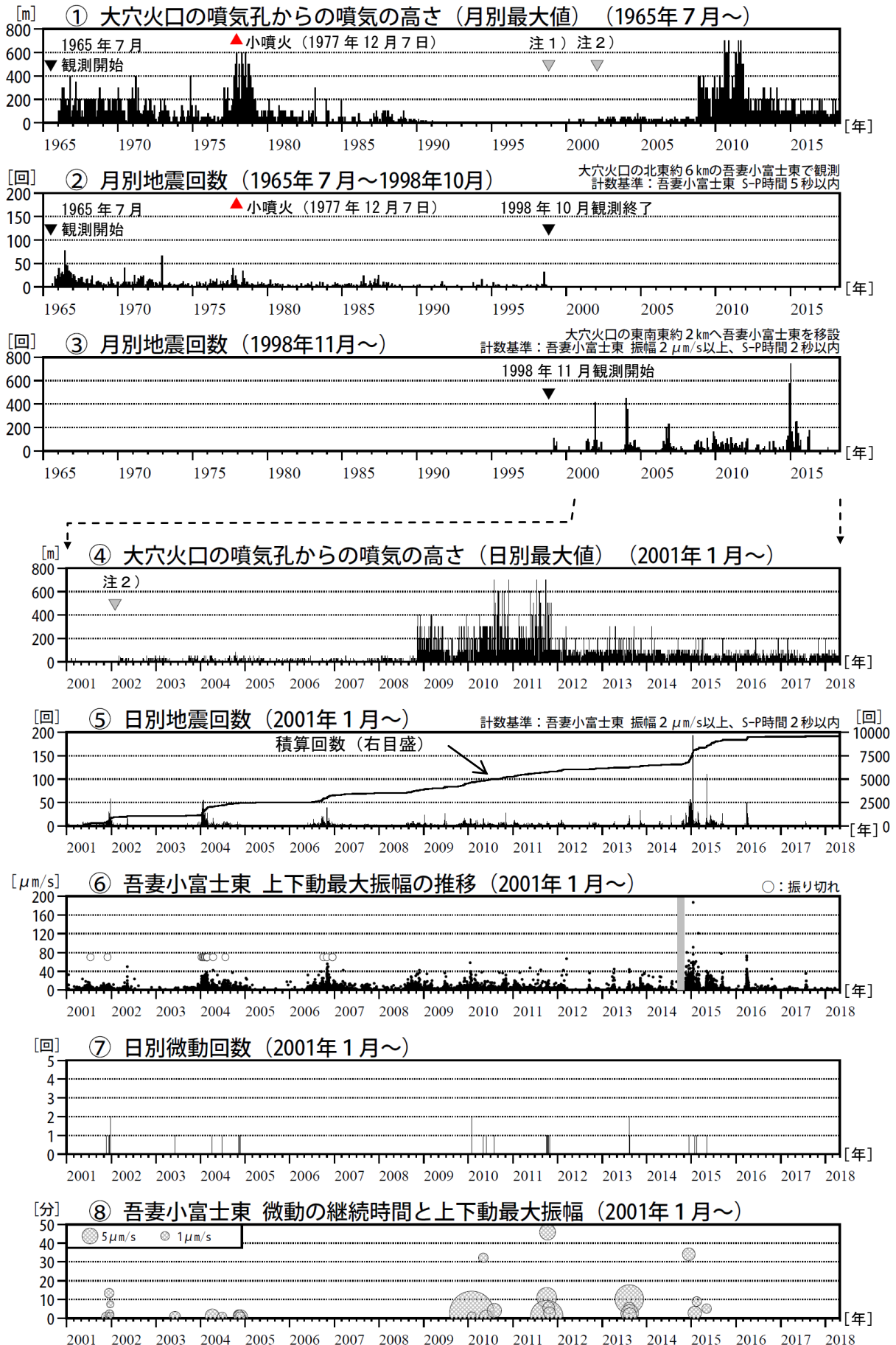
図2 吾妻山 火山活動経過図 (1965年7月～2018年4月)
