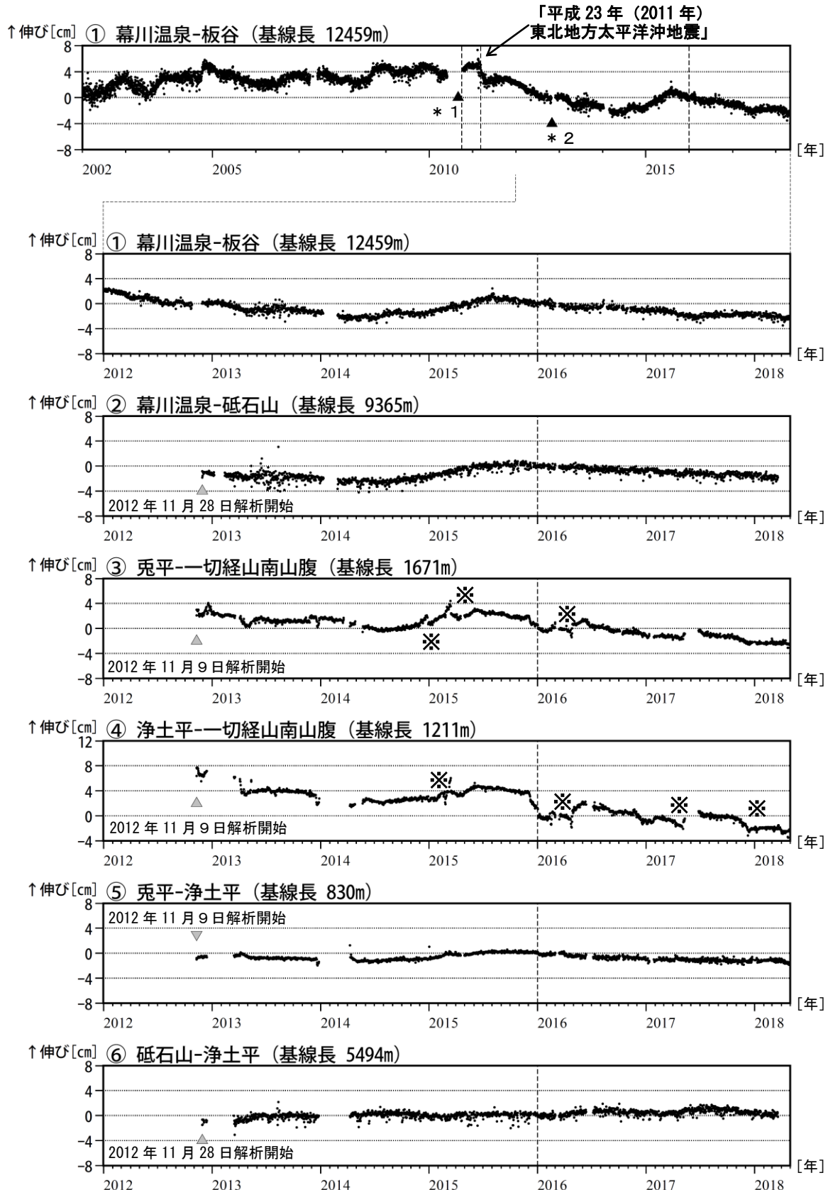
図3 吾妻山 GNSS 1) 基線長変化図 (2002年1月～2018年4月)
