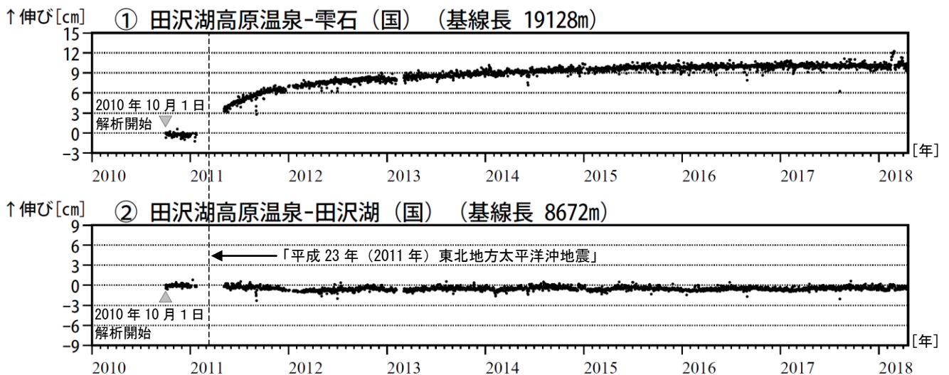
図7 秋田駒ヶ岳 GNSS 3) 基線長変化図 (2010年10月～2018年4月17日)
