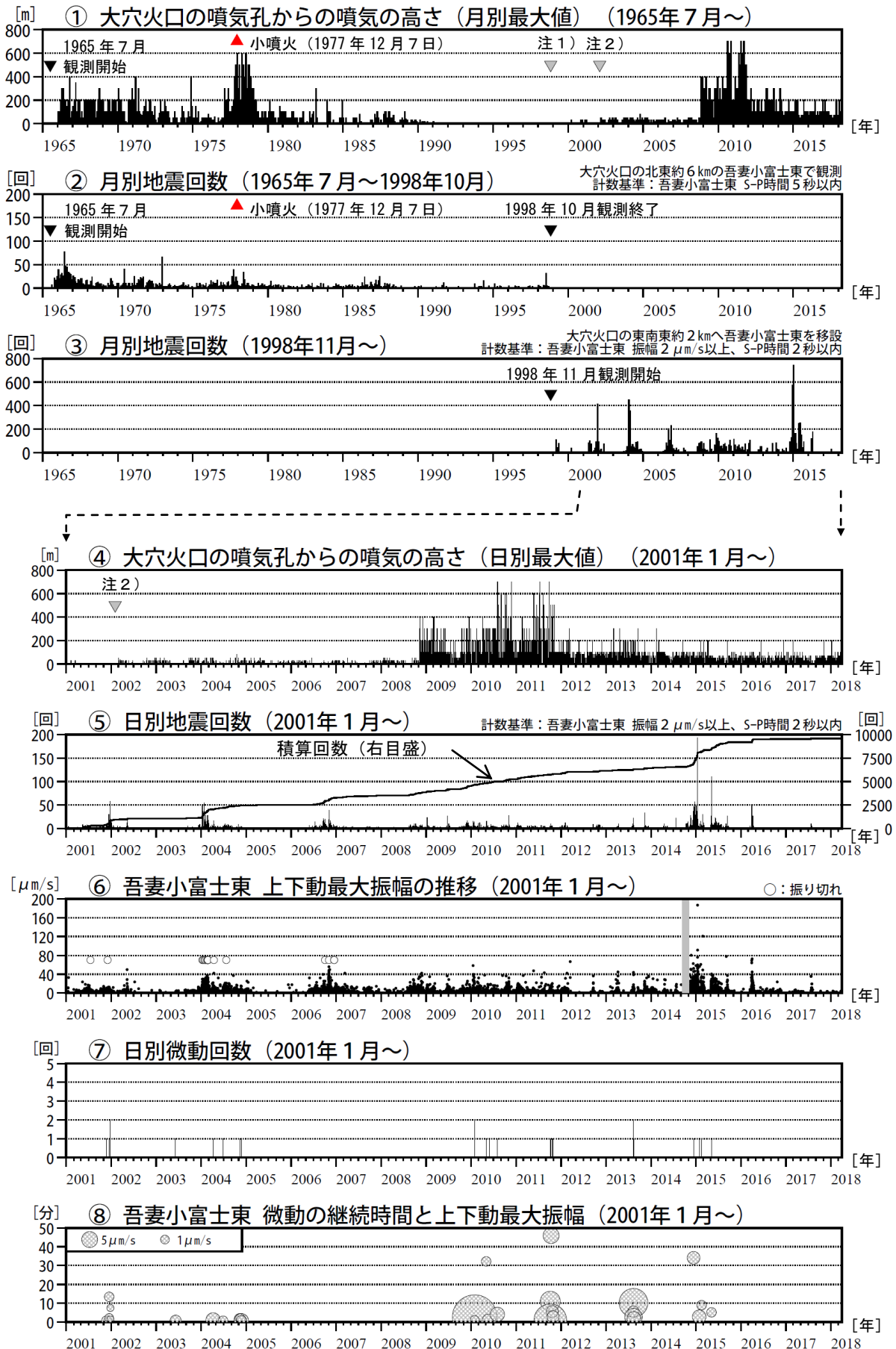
図5 吾妻山 火山活動経過図（1965年7月～2018年3月）
