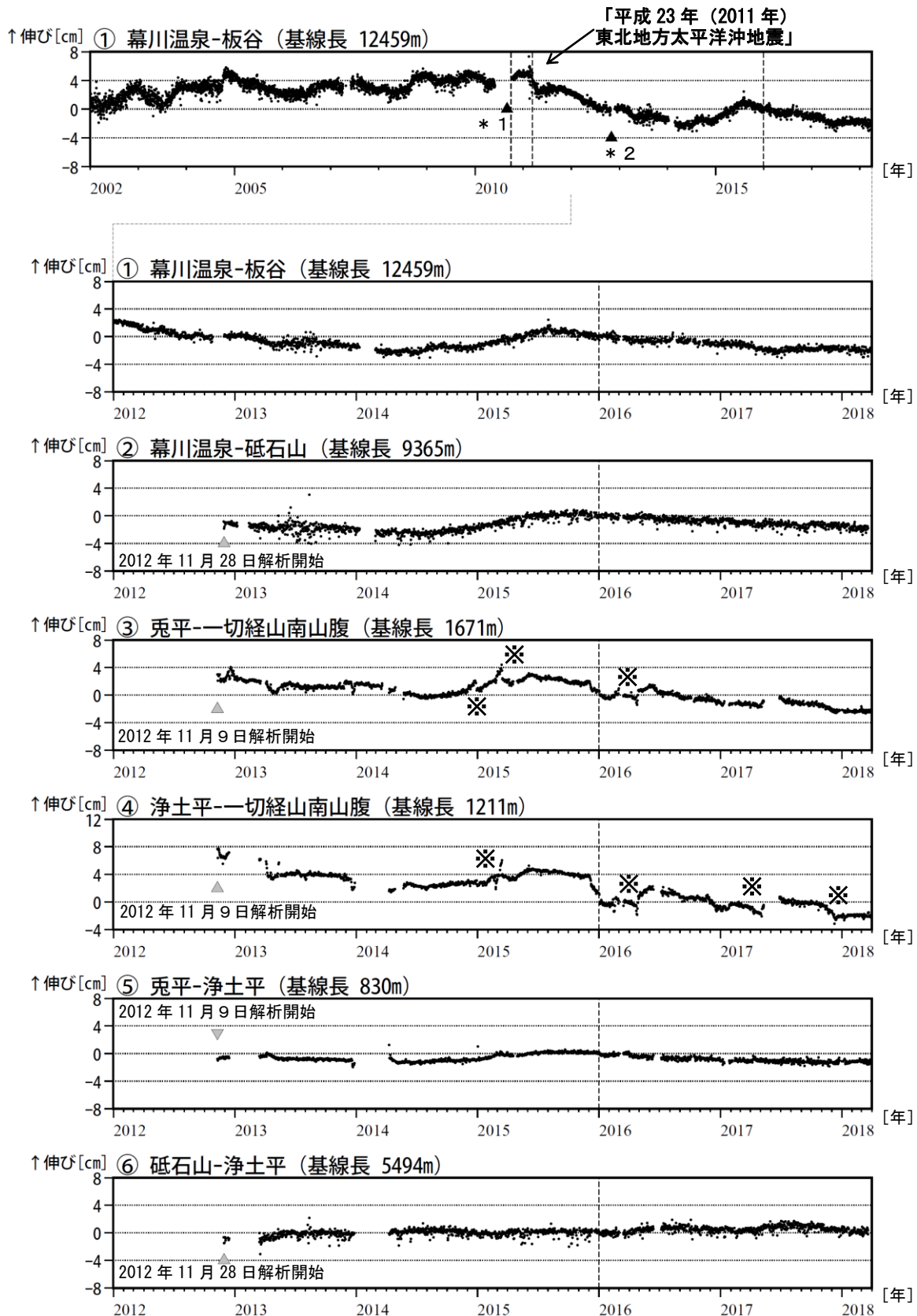
図 6 吾妻山 GNSS 2) 基線長変化図 (2002 年 1 月～2018 年 3 月)
