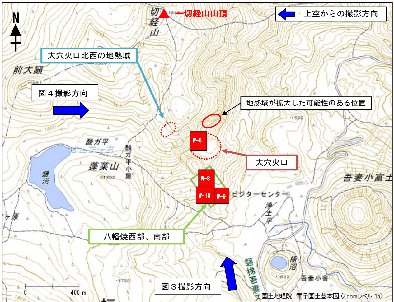
図 2 吾妻山 大穴火口付近の噴気と地熱域の分布及び写真と地表面温度分布 1) 撮影方向
