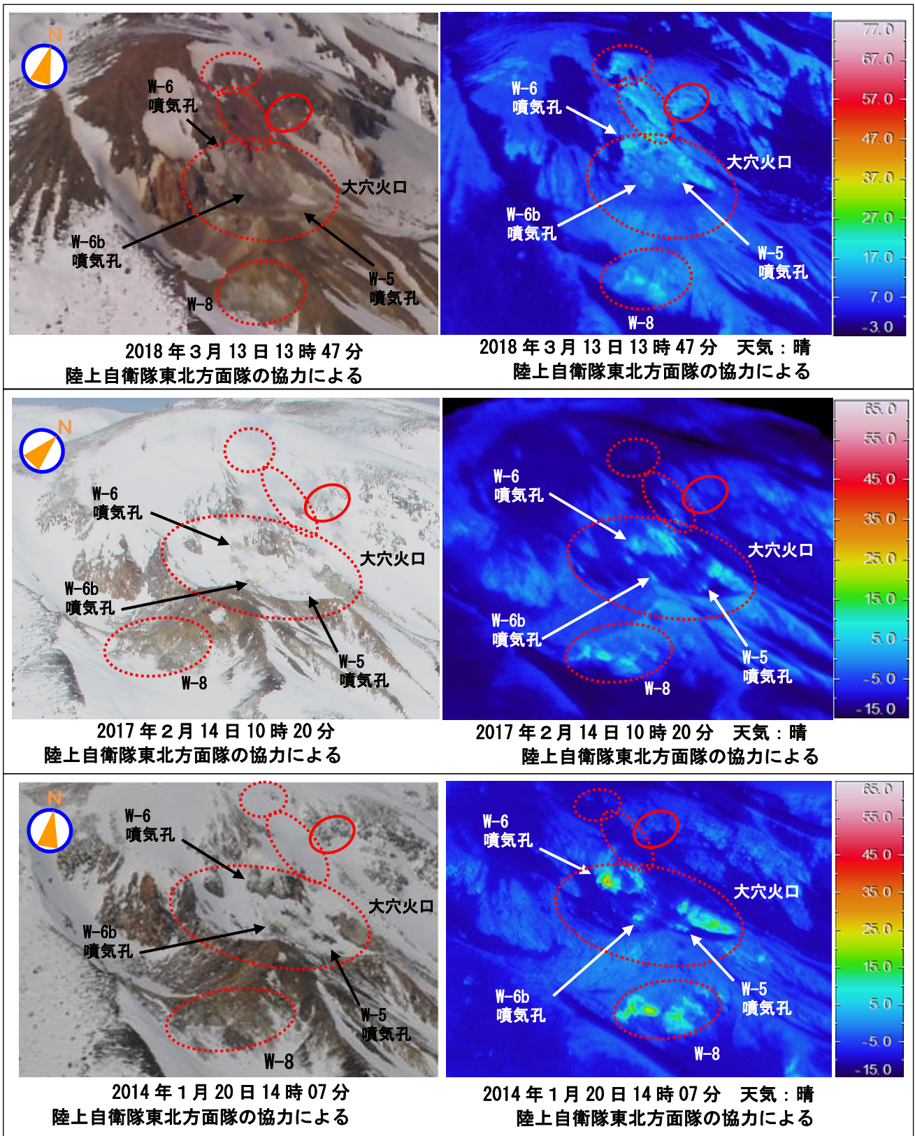
図3 吾妻山 上空から撮影した大穴火口及びその周辺の状況と地表面温度分布
