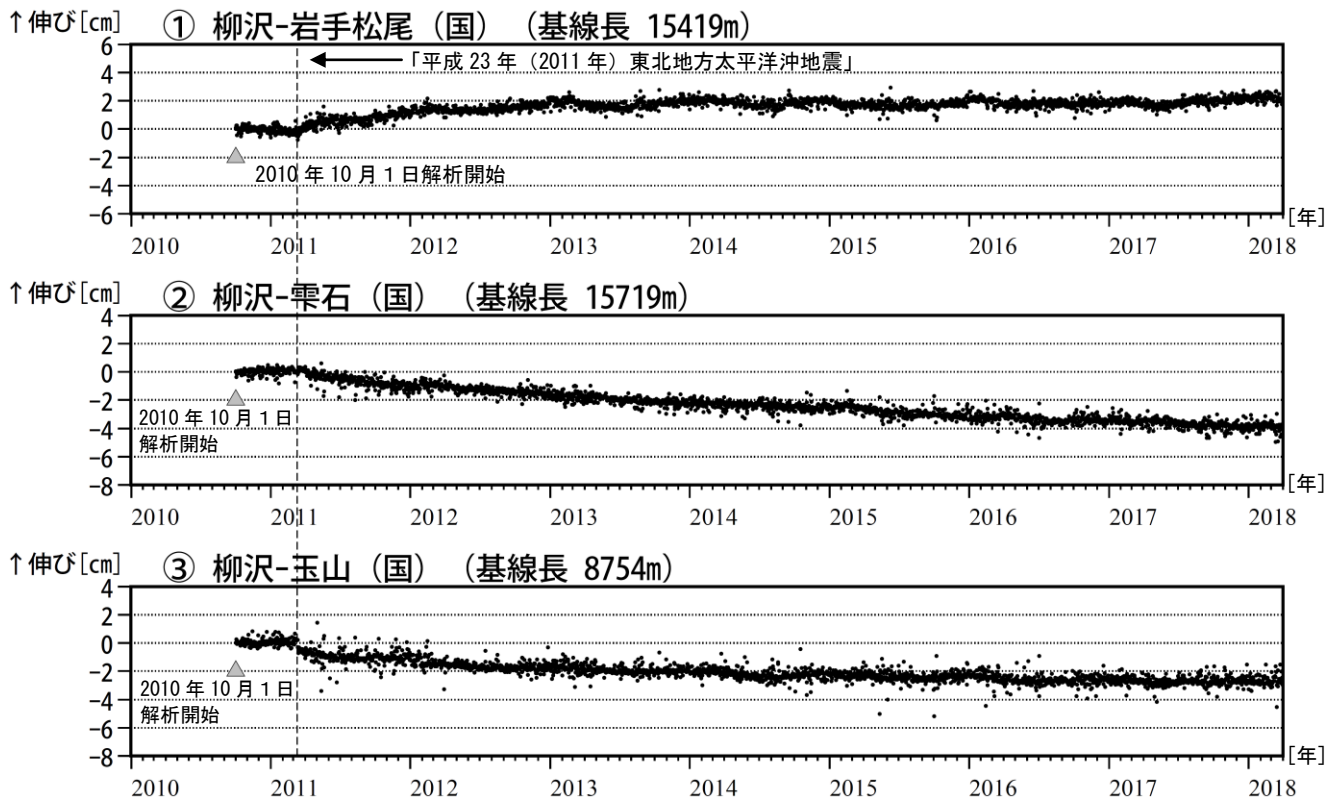
図 5 岩手山 GNSS 1) 基線長変化図（2010 年 10 月～2018 年 3 月）
