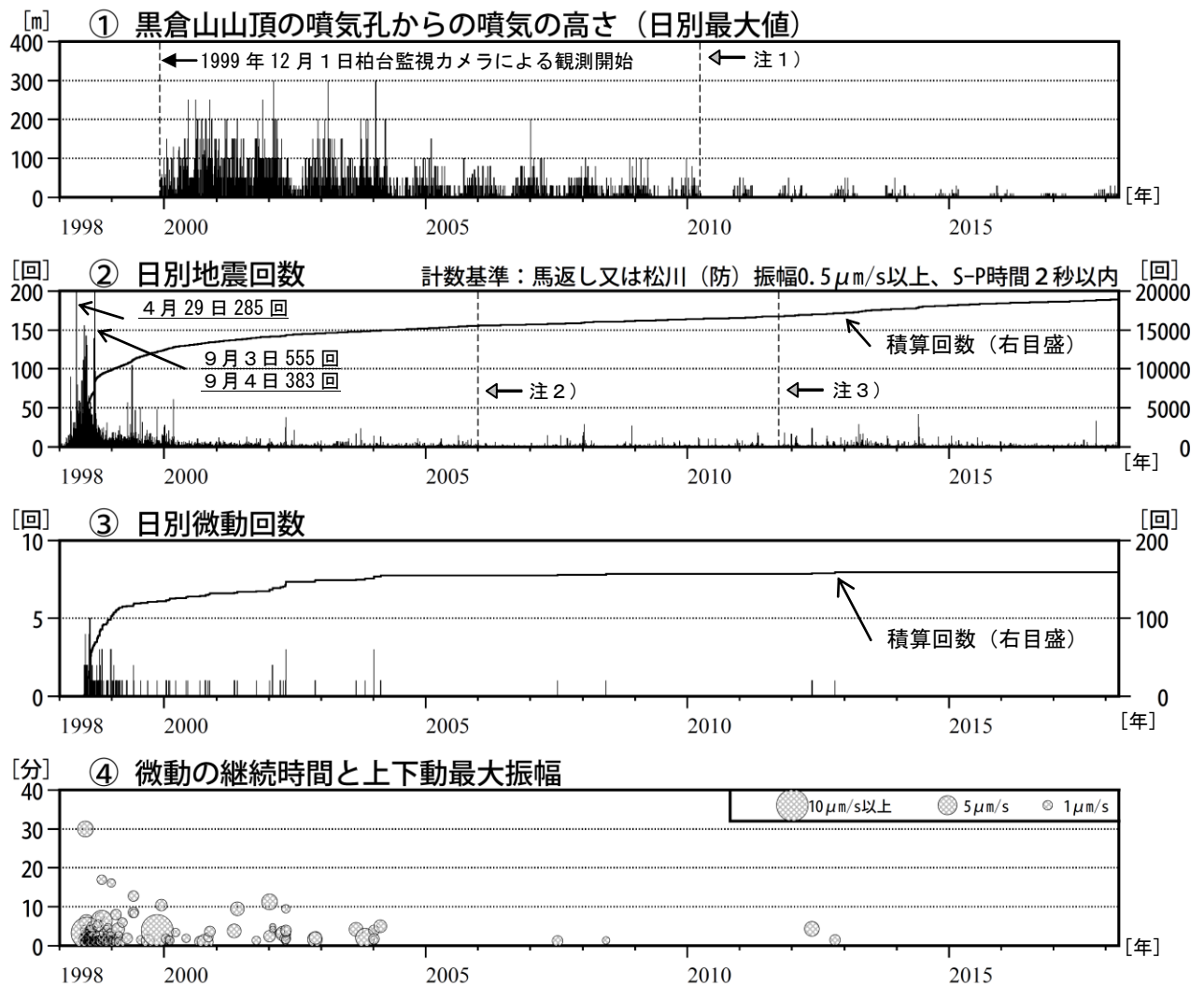
図 3 岩手山 火山活動経過図（1998 年 1 月～2018 年 3 月）
