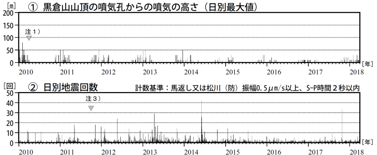
図 4 岩手山 噴気の高さ及び日別地震回数（2010 年 1 月～2018 年 3 月）
