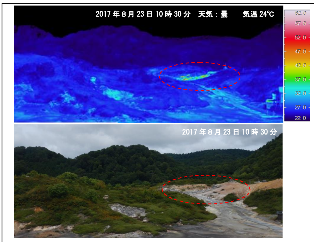
図3 恐山 南東から撮影した地獄谷噴気地帯の状況と地表面温度分布
