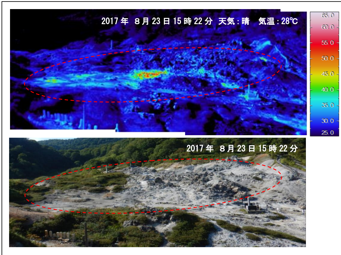
図 4 恐山 南東から撮影した地獄谷噴気地帯の状況と地表面温度分布
