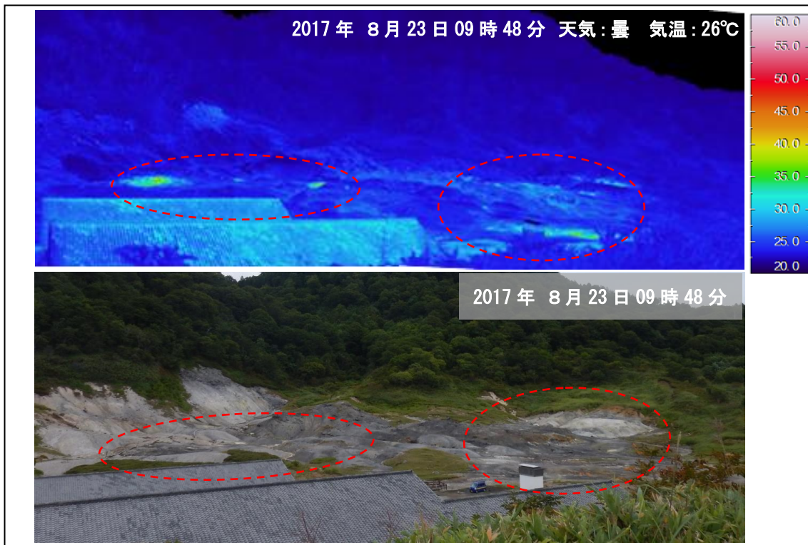
図2 恐山 南から撮影した花染の湯付近北側の状況と地表面温度分布
