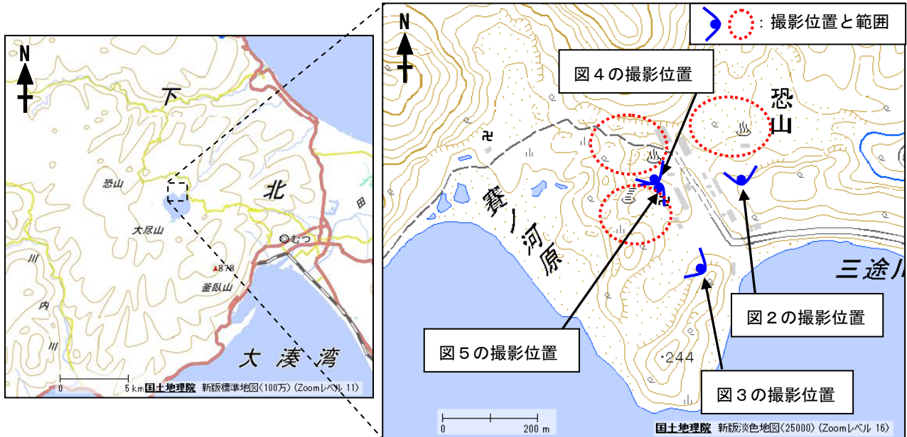
図 1 恐山 宇曾利山湖北岸の噴気地熱地帯周辺の写真と地表面温度分布 1) 撮影位置
