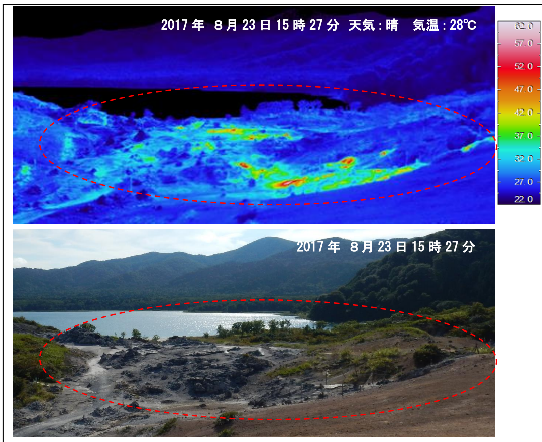
図 5 恐山 東北東から撮影した地獄谷噴気地帯の状況と地表面温度分布
