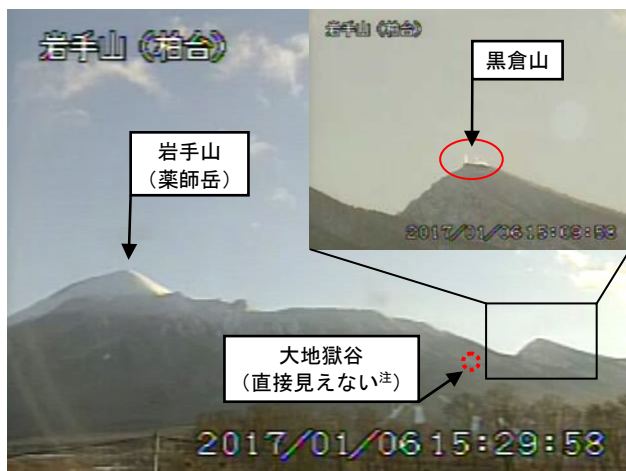
図 1 岩手山 黒倉山の噴気の状況 （1 月 6 日）
