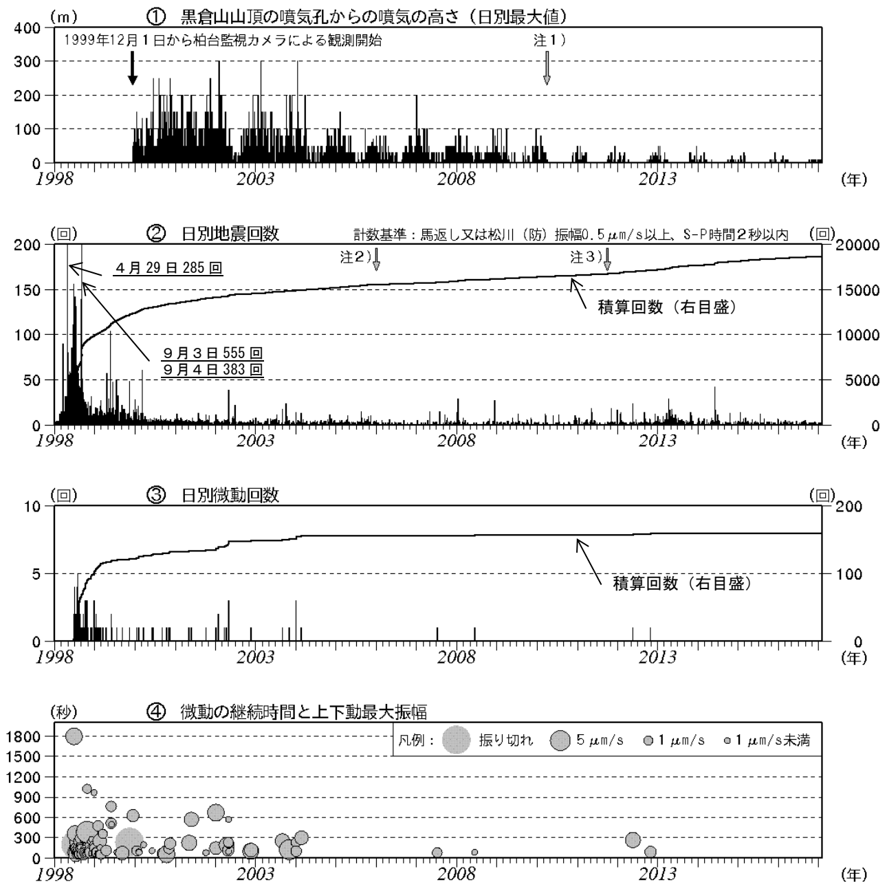
図3 岩手山 火山活動経過図（1998年1月～2017年1月）
