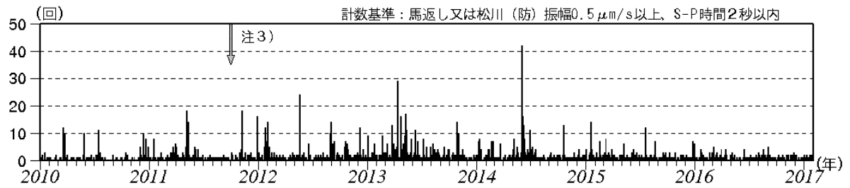
図4 岩手山 日別地震回数（2010年1月～2017年1月）
