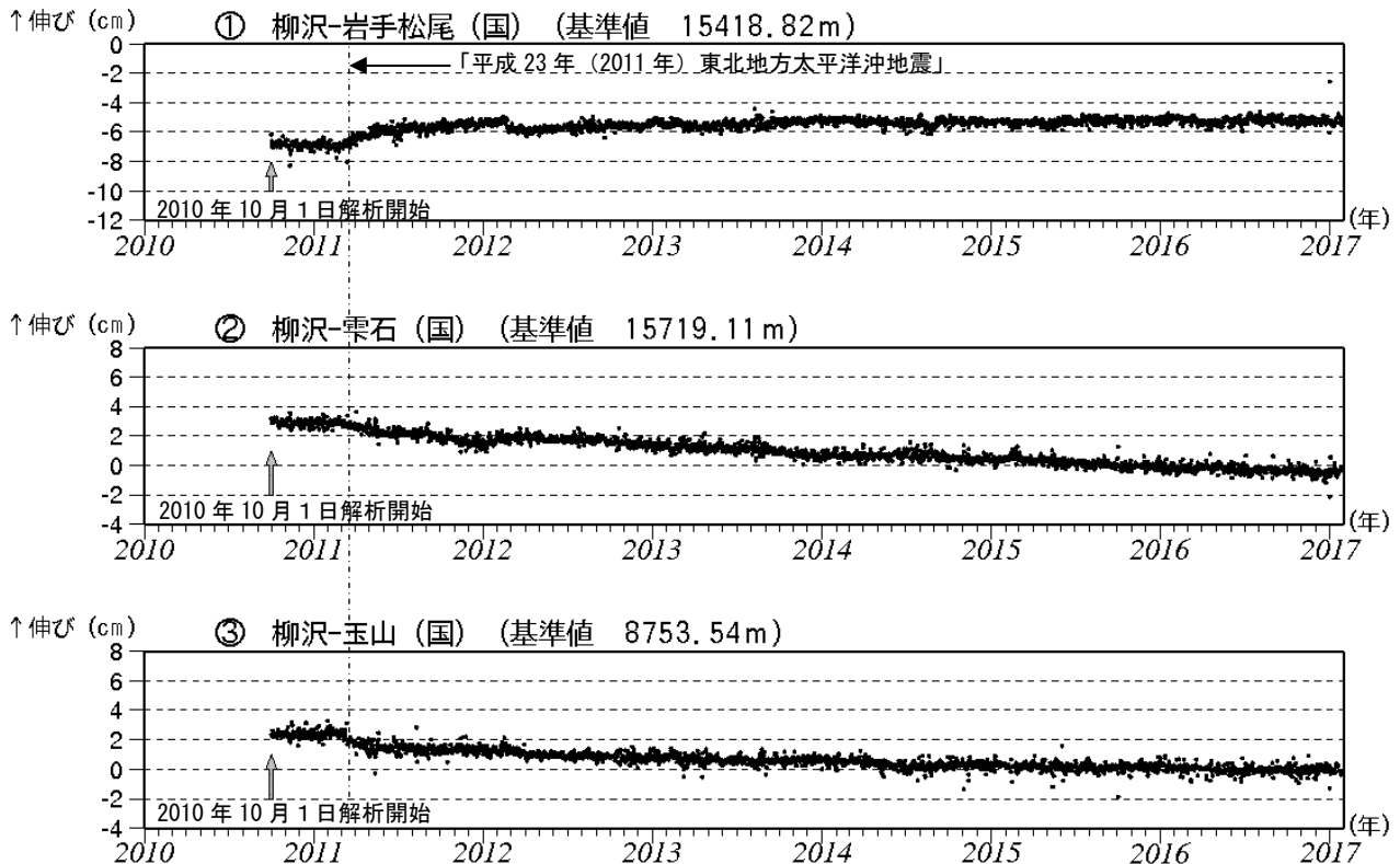
図5 岩手山 GNSS 1) 基線長変化図（2010年10月～2017年1月）
