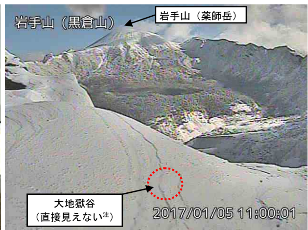
図 2 岩手山 黒倉山監視カメラからの状況 （1 月 5 日）
