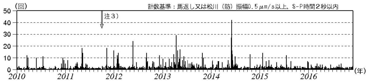
図3 岩手山 日別地震回数（2010年1月～2016年11月）
