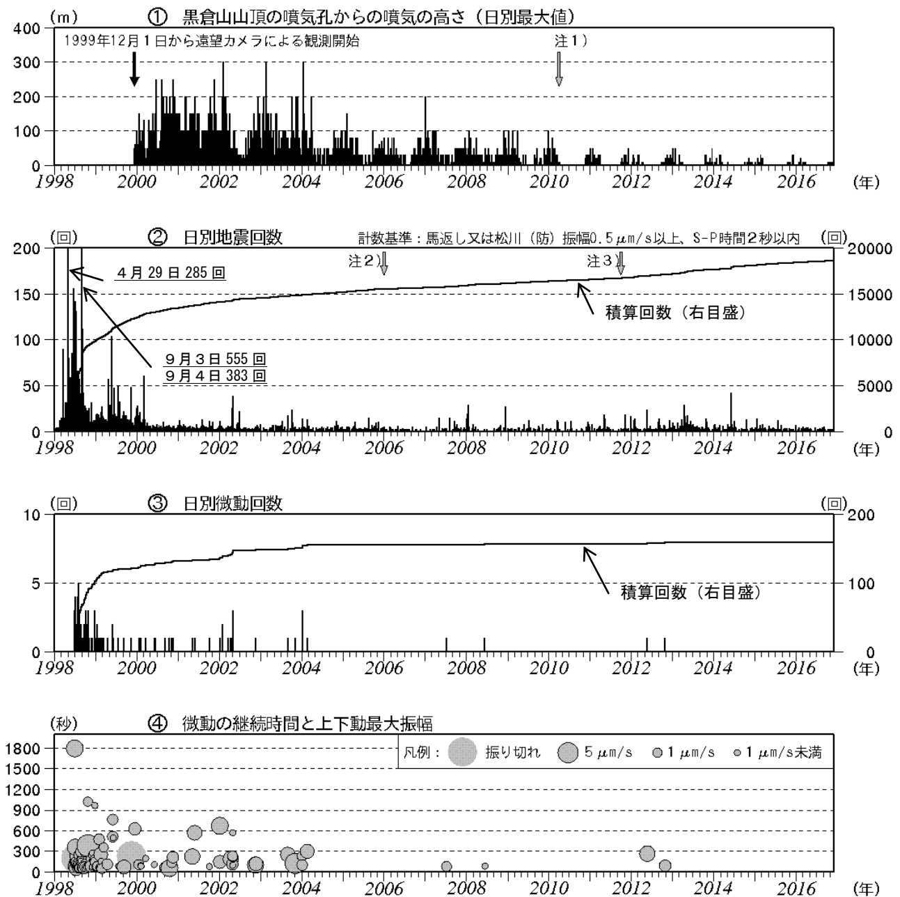
図2 岩手山 火山活動経過図（1998年1月～2016年11月）
