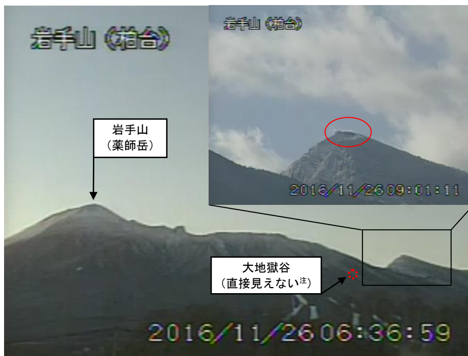
図 1 岩手山 黒倉山の噴気の状況（11 月 26 日）
