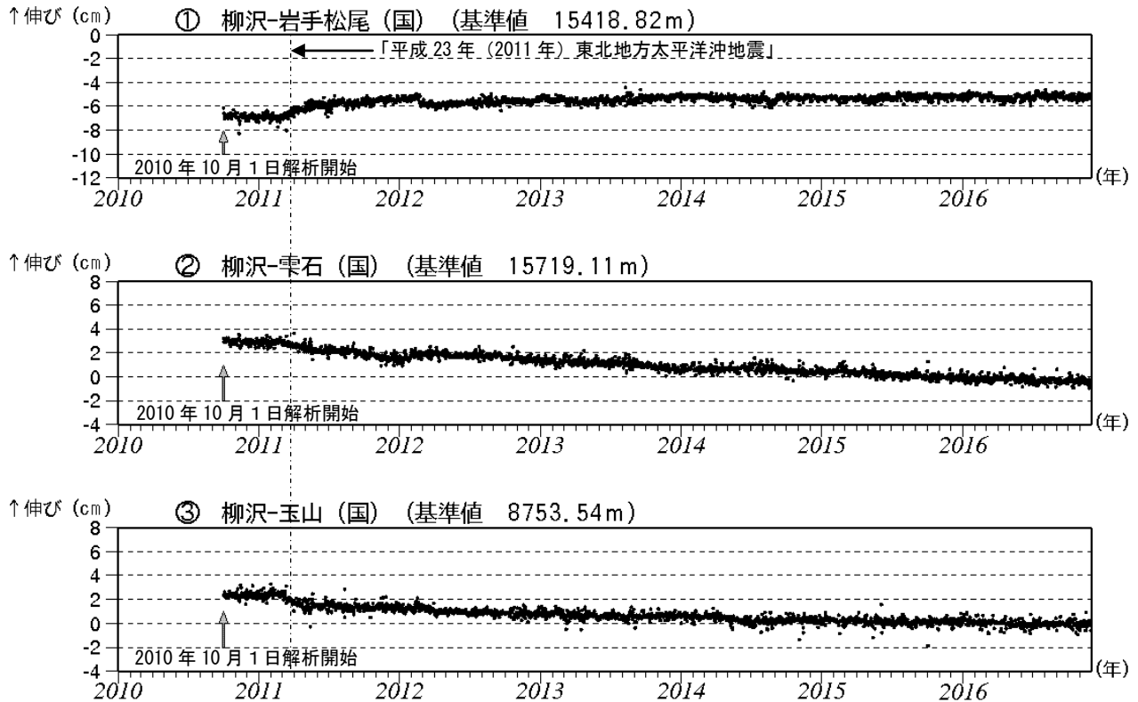
図4 岩手山 GNSS 1) 基線長変化図（2010年10月～2016年11月）
