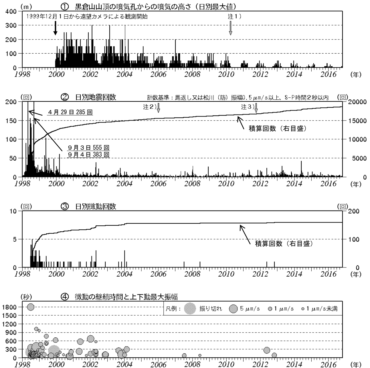
図2 岩手山 火山活動経過図（1998年1月～2016年10月）
