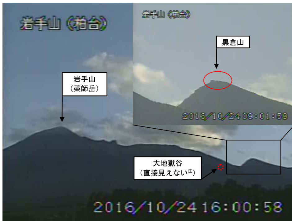
図 1 岩手山 黒倉山の噴気の状況（10 月 24 日）
