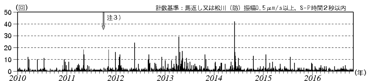
図3 岩手山 日別地震回数（2010年1月～2016年10月）
