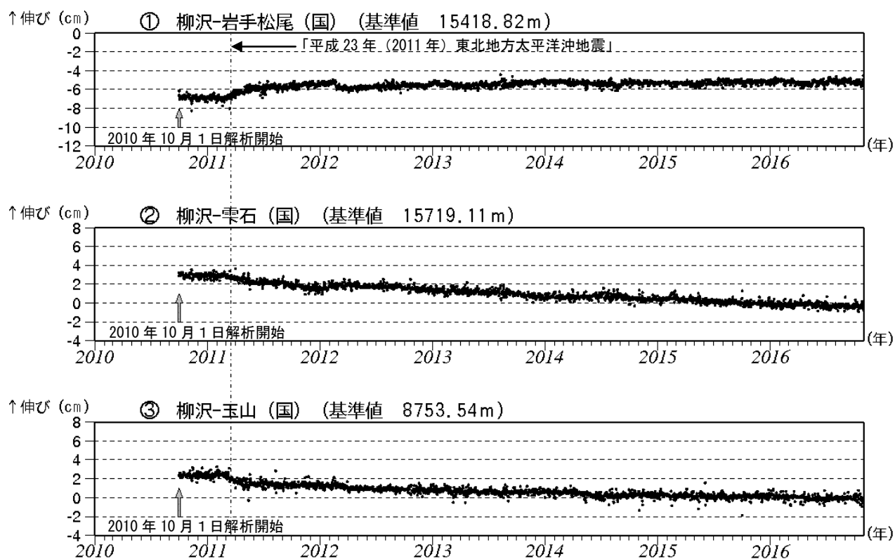
図4 岩手山 GNSS 1) 基線長変化図（2010年10月～2016年10月）
