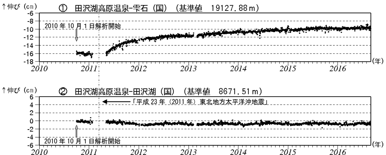
図6 秋田駒ヶ岳 GNSS 基線長変化図（2010年10月～2016年8月）
