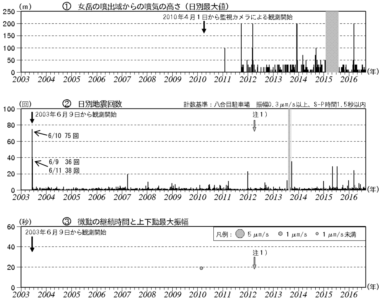
図5 秋田駒ヶ岳 火山活動経過図（2003年6月～2016年8月）
