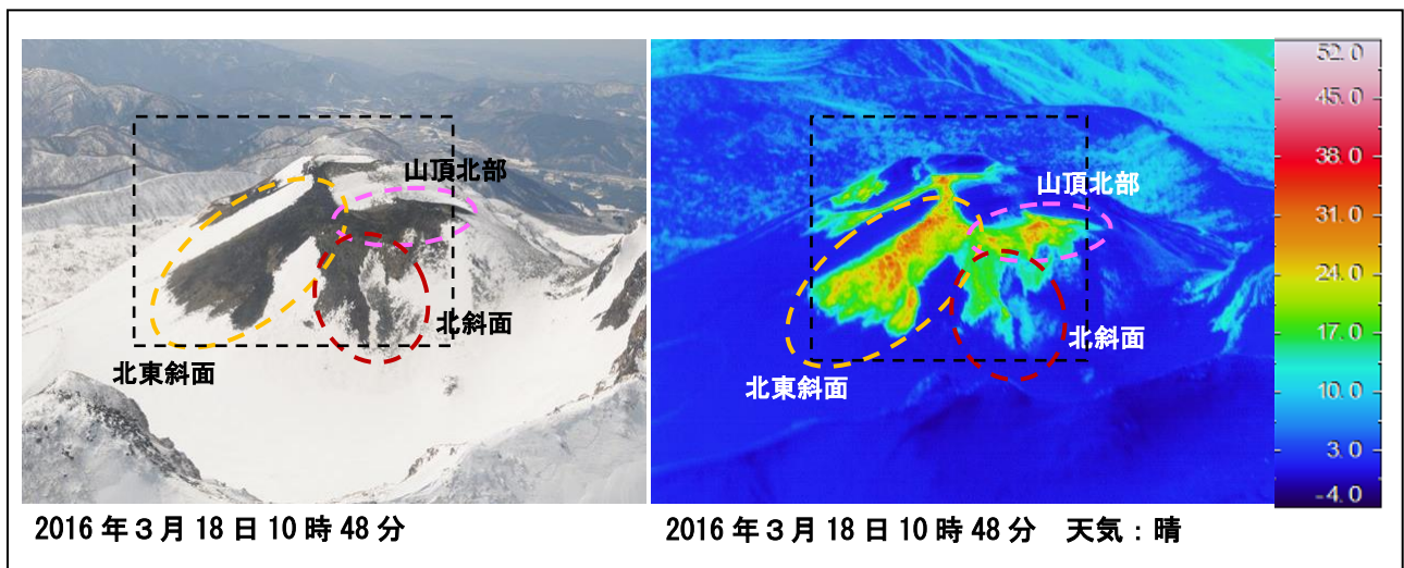
図4 秋田駒ヶ岳 上空からの北東斜面、北斜面、山頂北部の状況と地表面温度分布
