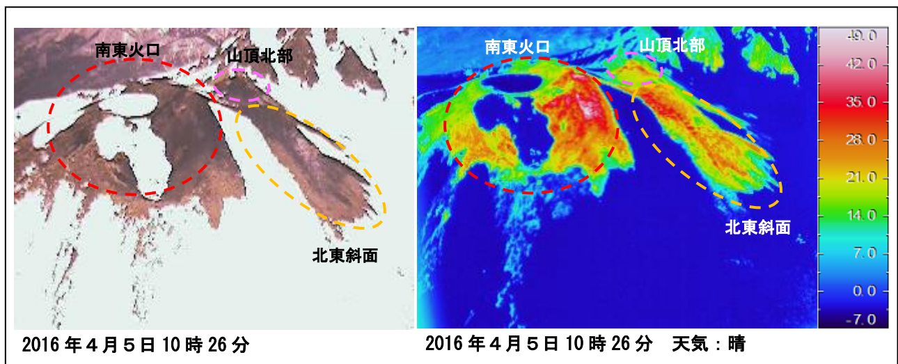
図3 秋田駒ヶ岳 上空からの南東火口の状況と地表面温度分布
