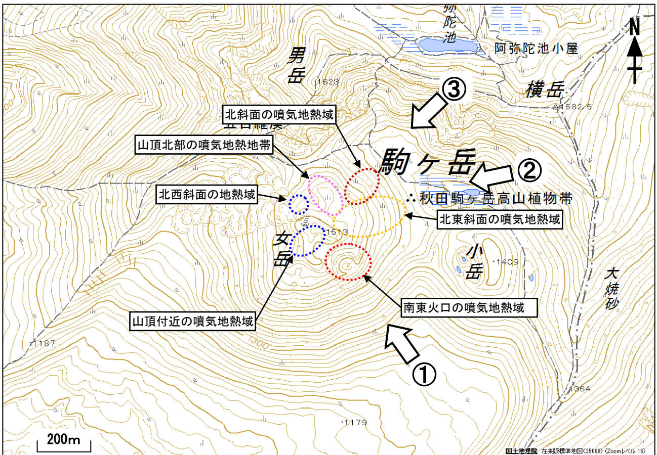
図 2 秋田駒ヶ岳 女岳の地熱域の分布図及び上空からの写真と地表面温度分布 1) 撮影方向
