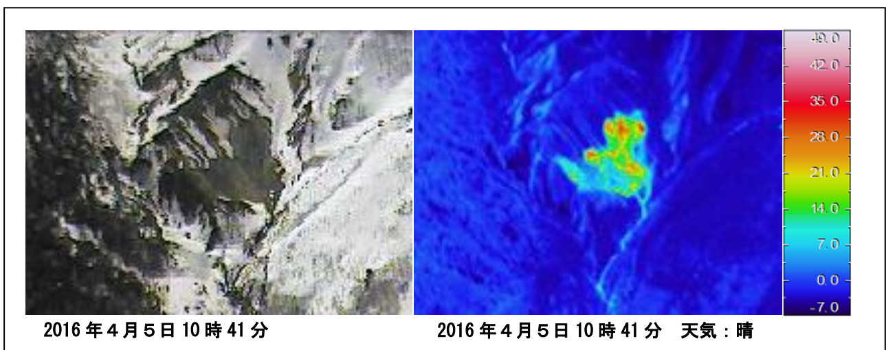
図4 岩手山 上空からの大地獄谷の状況と地表面温度分布 ・岩手県の協力により撮影しました。
