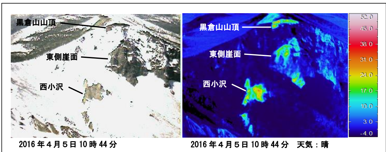
図3 岩手山 上空からの黒倉山山頂、黒倉山東側崖面及び西小沢の状況と地表面温度分布 ・岩手県の協力により撮影しました。
