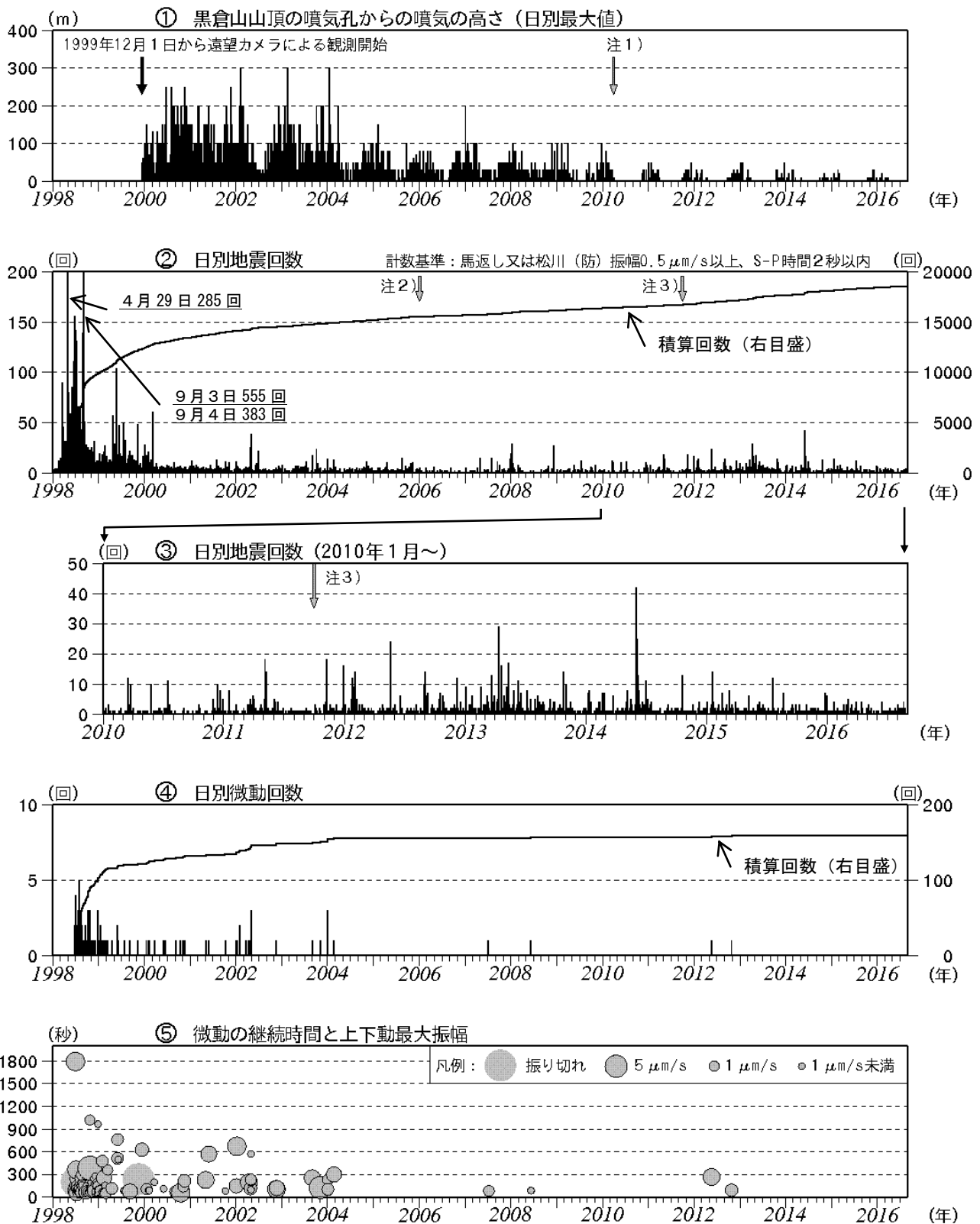
図5 岩手山 火山活動経過図（1998年1月～2016年8月）
