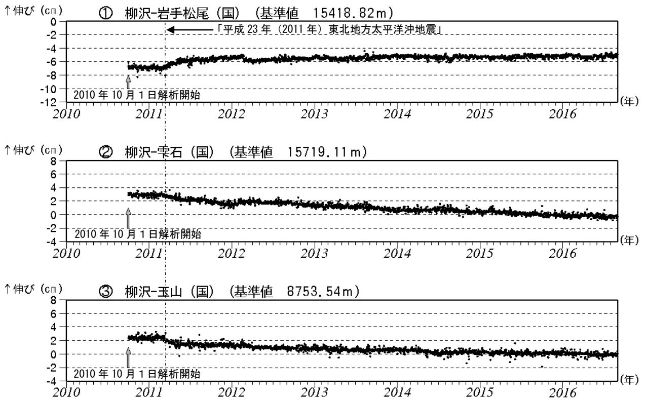
図6 岩手山 GNSS 2) 基線長変化図 (2010年10月～2016年8月)
