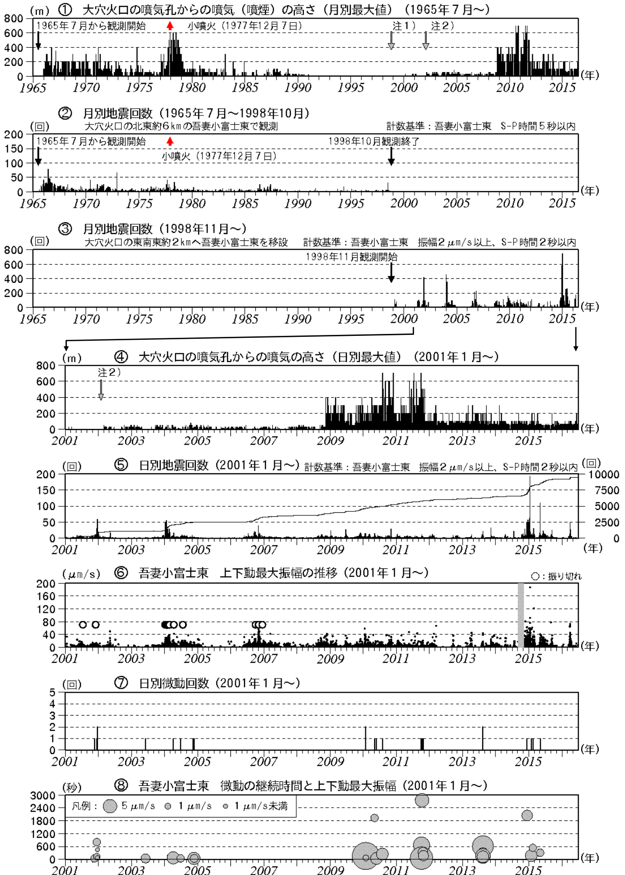
図3 吾妻山 火山活動経過図(1965年7月~2016年6月)
