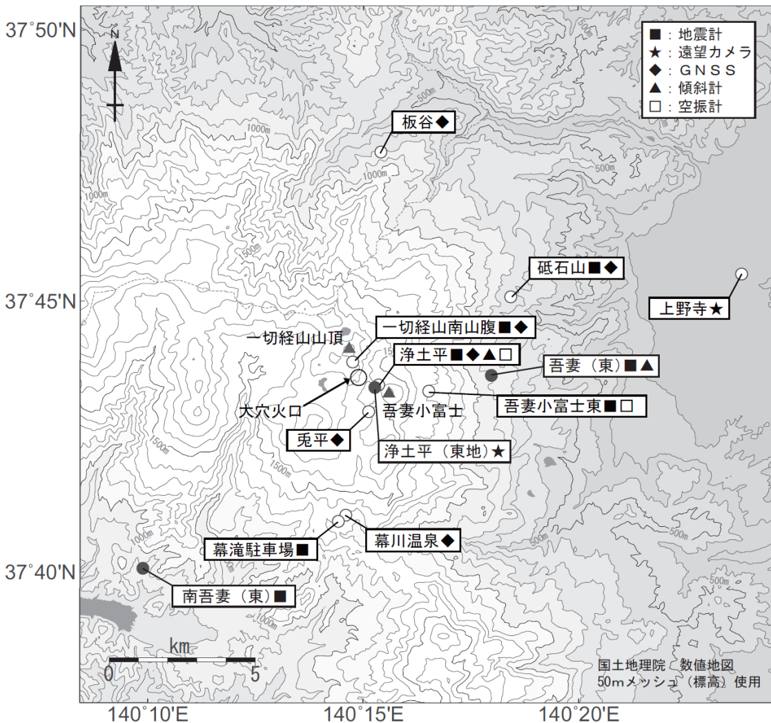
図2 吾妻山 観測点配置図
