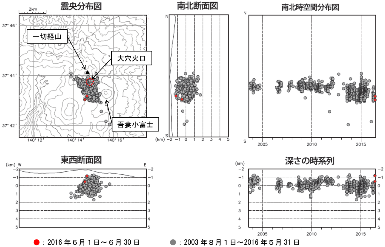
● : 2016 年 6 月 1 日～6 月 30 日 ● : 2003 年 8 月 1 日～2016 年 5 月 31 日 図 4 吾妻山 地震活動 (2003 年 8 月～2016 年 6 月) ・ 2012 年 12 月 1 日以降、観測点の移設更新の影響により、震源がやや南側に分布する傾向がみられます。
