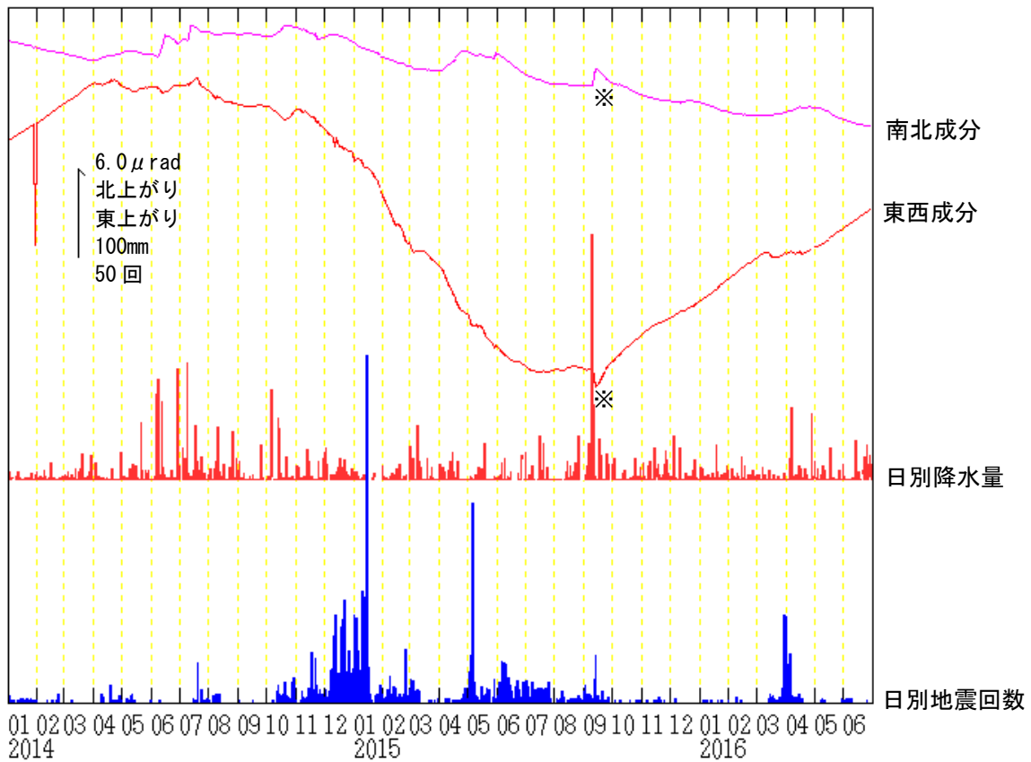
図 5 吾妻山 浄土平観測点での傾斜変動 (2014 年 1 月～2016 年 6 月、時間値、潮汐補正あり) ・ 1 \mu\text{rad} (マイクロラジアン) は、1 km 先が 1 mm 上下するような変化量です。 ・ 2015 年 6 月頃までみられていた西南西側 (火口方向側) 上がりの変動は、2015 年 7 月頃から停滞していましたが、2015 年 9 月頃から西側下がり傾向となっています。 ・ 日別降水量は鷺倉地域気象観測所で観測された値です。 ※ 「平成 27 年 9 月関東・東北豪雨」による変動です。
