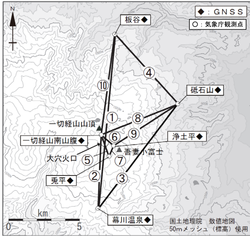
図6 吾妻山 GNSS 観測点配置図
