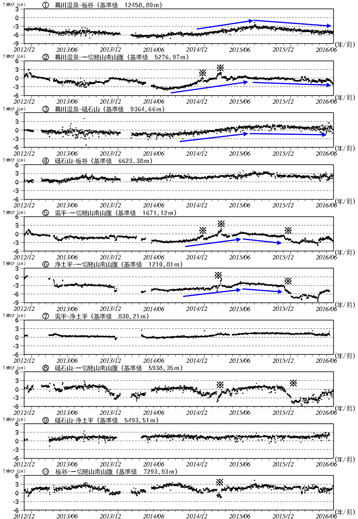
図 7-2 吾妻山 GNSS 基線長変化図 (2012 年 12 月～2016 年 6 月)
