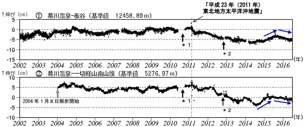
図7-1 吾妻山 GNSS 基線長変化図 (2002 年 1 月～2016 年 6 月)
