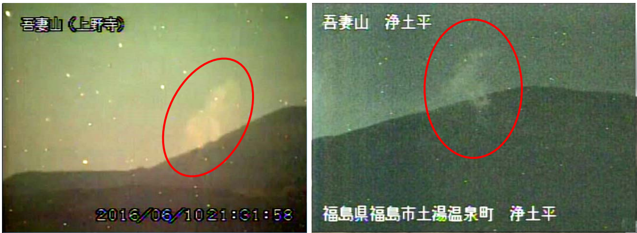
図1 吾妻山 大穴火口周辺の噴気の状況（6月10日）
