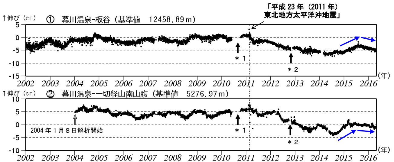
図8-1 吾妻山 GNSS 基線長変化図 (2002年1月～2016年4月)
