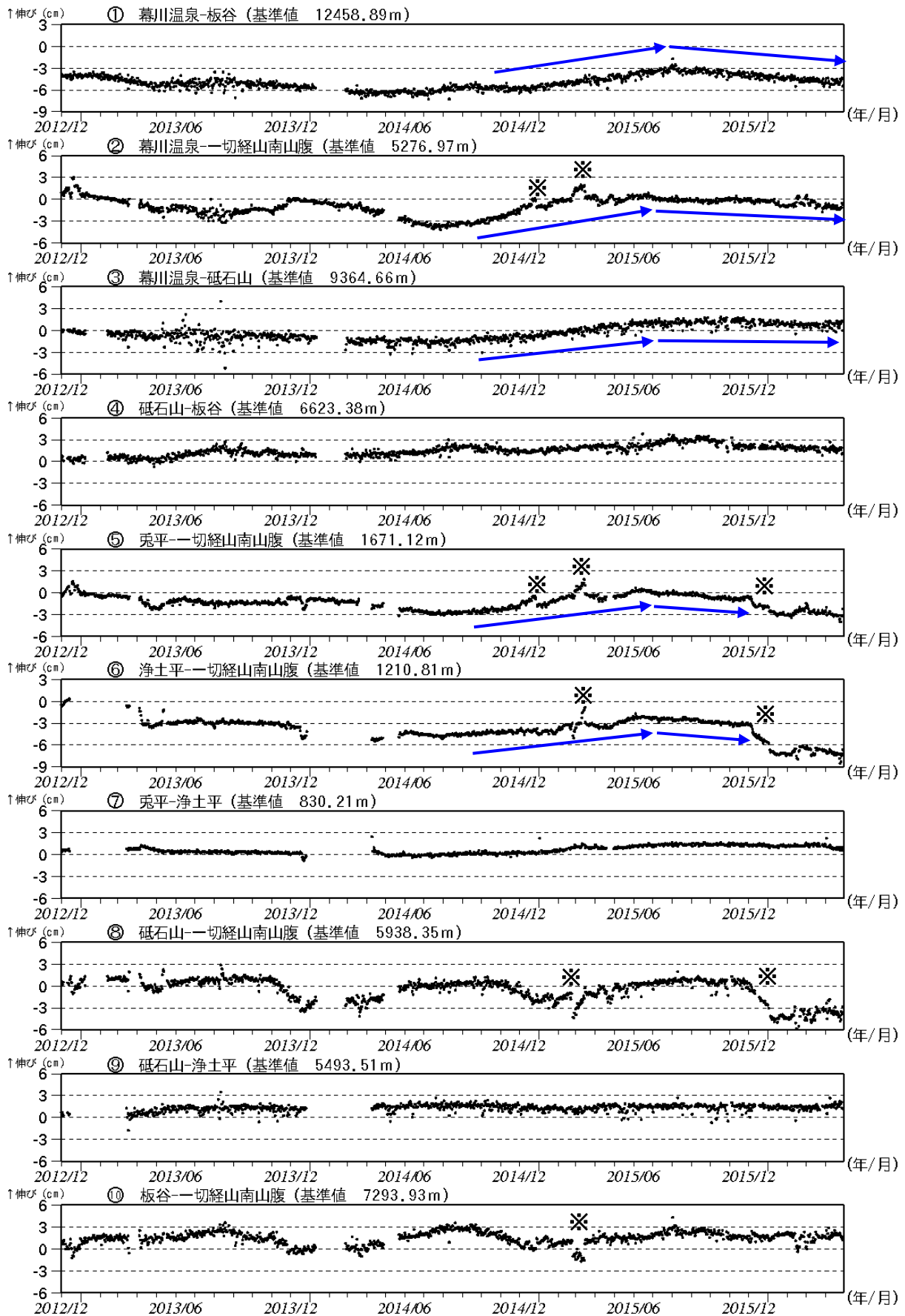
図 8-2 吾妻山 GNSS 基線長変化図 (2012 年 12 月～2016 年 4 月)
