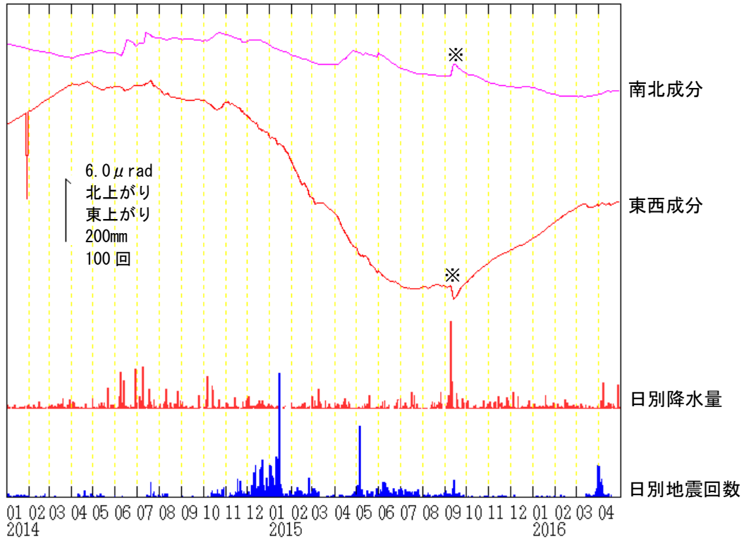
図 6 吾妻山 浄土平観測点での傾斜変動
