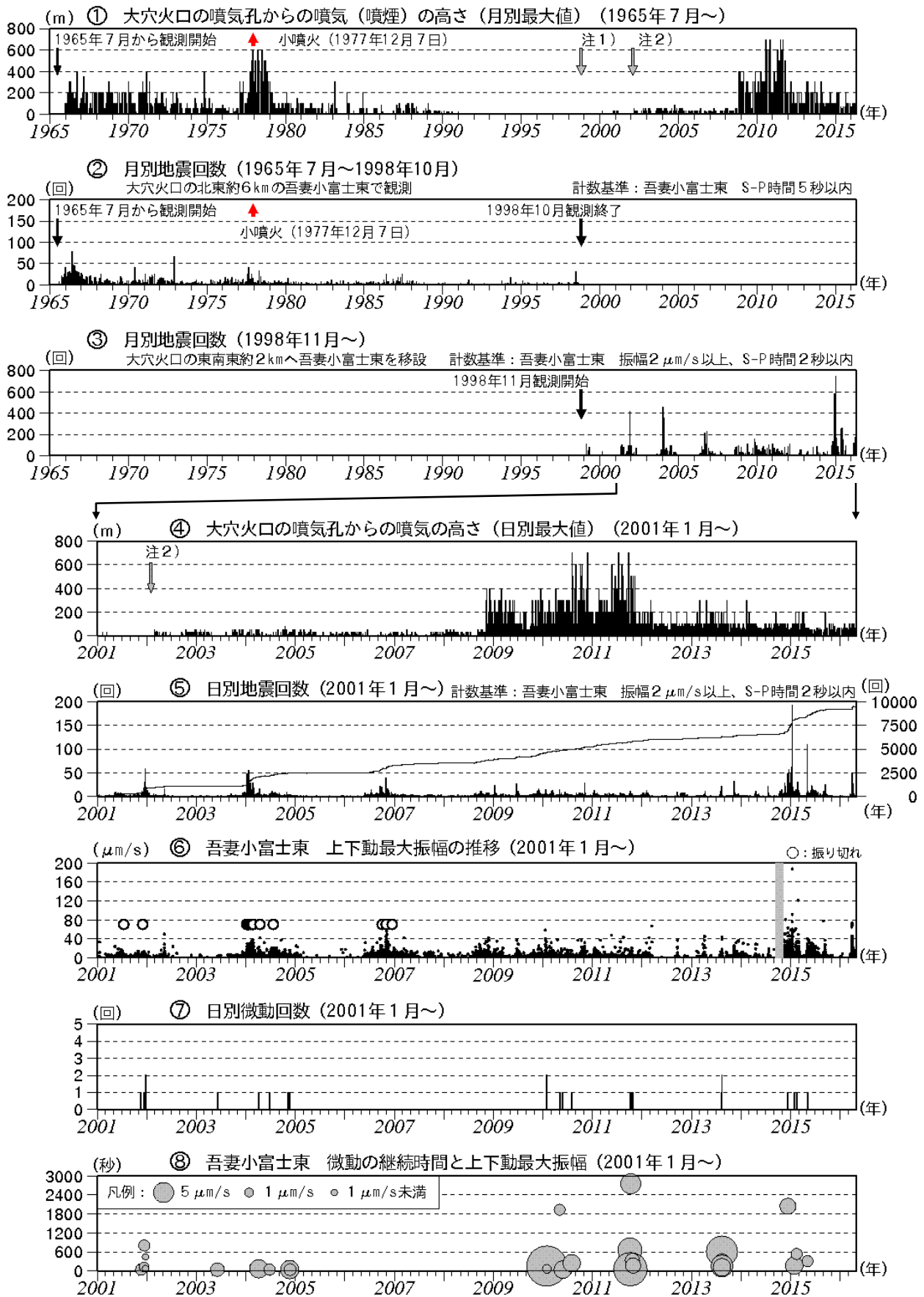
図4 吾妻山 火山活動経過図(1965年7月~2016年4月)
