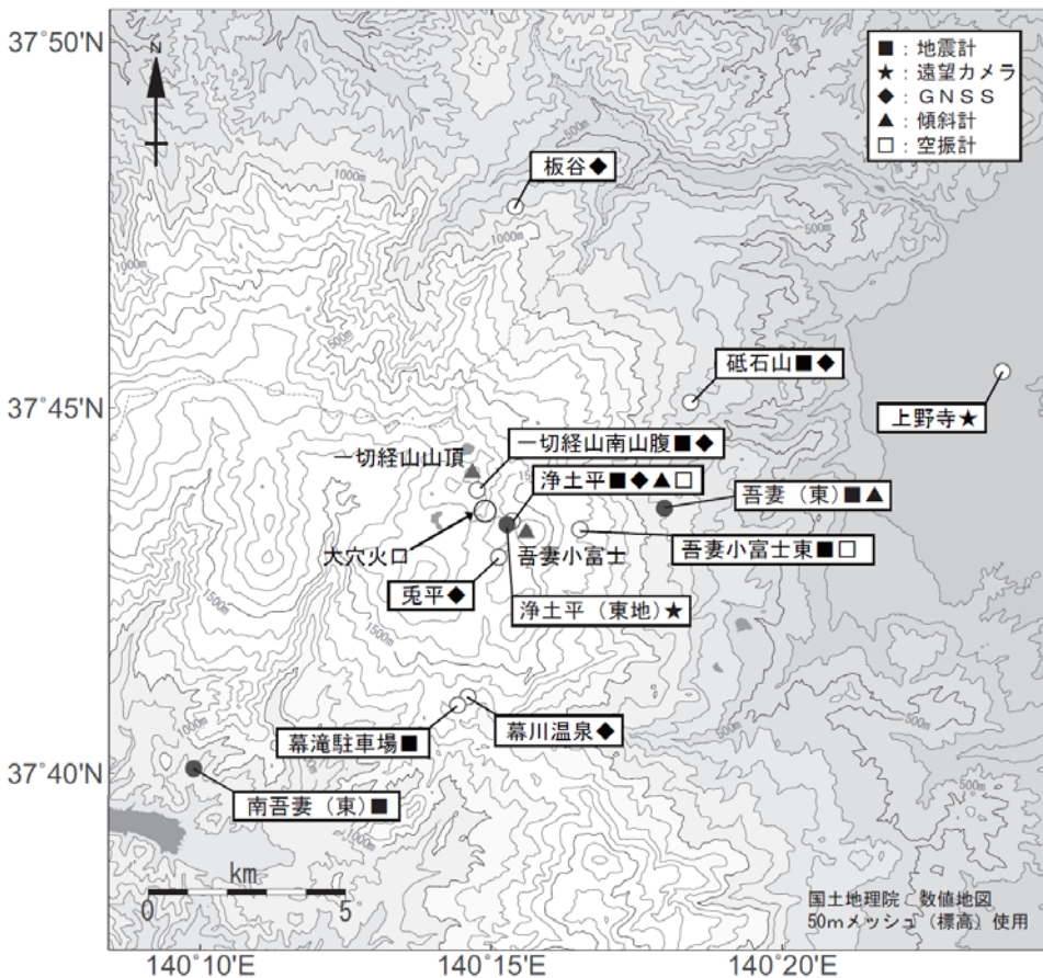
図2 吾妻山 観測点配置図
