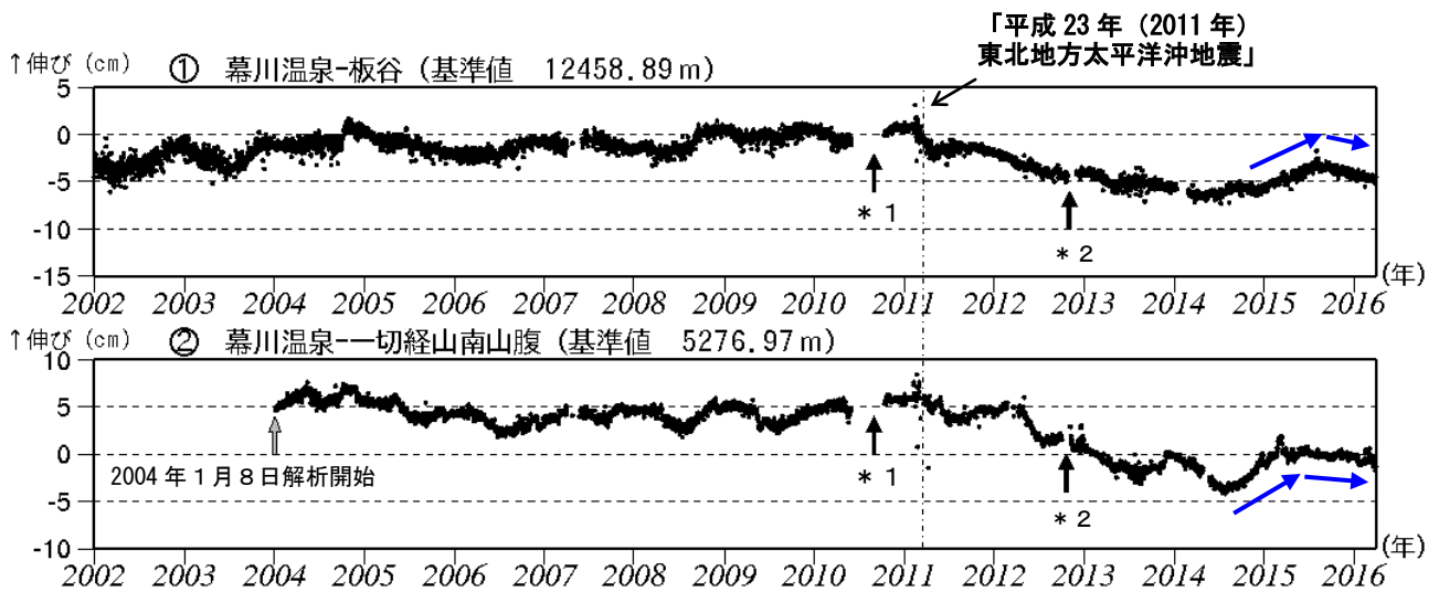
図10-1 吾妻山 GNSS 基線長変化図 (2002年1月～2016年3月)
