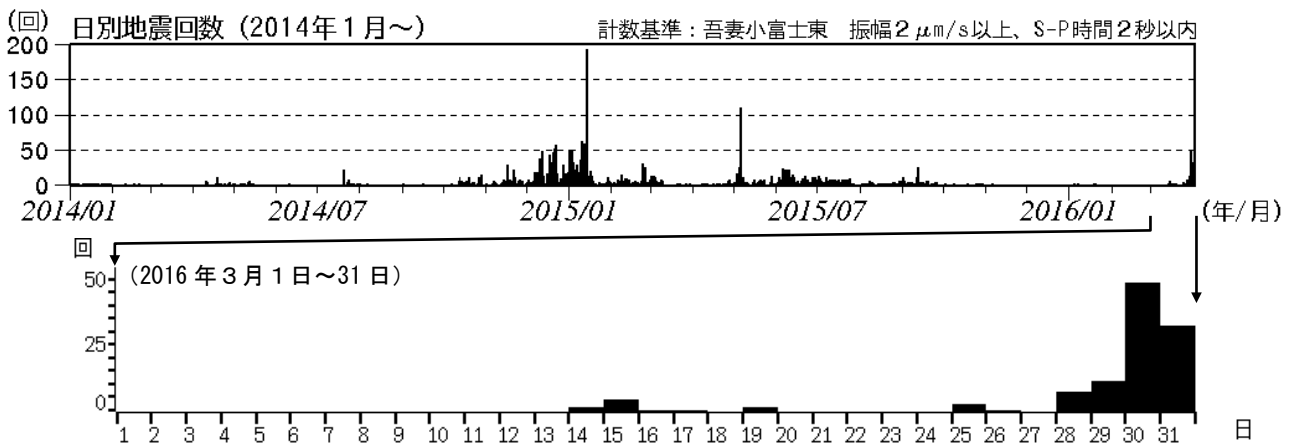
図5 吾妻山 日別地震回数 (2014年1月~2016年3月)
