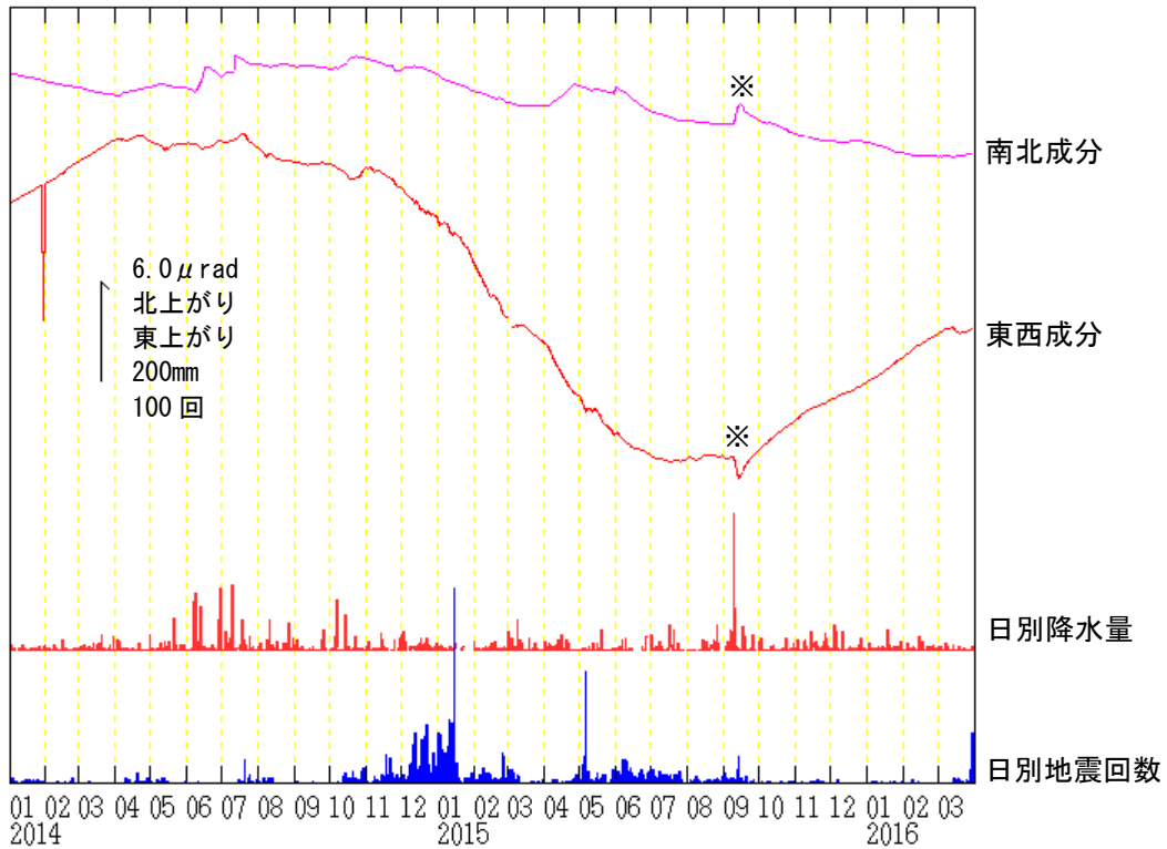
図 8 吾妻山 浄土平観測点での傾斜変動 （2014 年 1 月 1 日～2016 年 3 月 31 日、時間値、潮汐補正あり） ・ 1 \mu\text{rad} （マイクロラジアン）は、1 km 先が 1 mm 上下するような変化量です。 ・ 2014 年 7 月頃からみられている西南西側（火口方向側）上がりの傾向は、2015 年 7 月頃から停滞していましたが、9 月頃から西側下がりの傾向がみられています。 ・ 日別降水量は鷲倉地域気象観測所の値です。 ※ 「平成 27 年 9 月関東・東北豪雨」による変動です。
