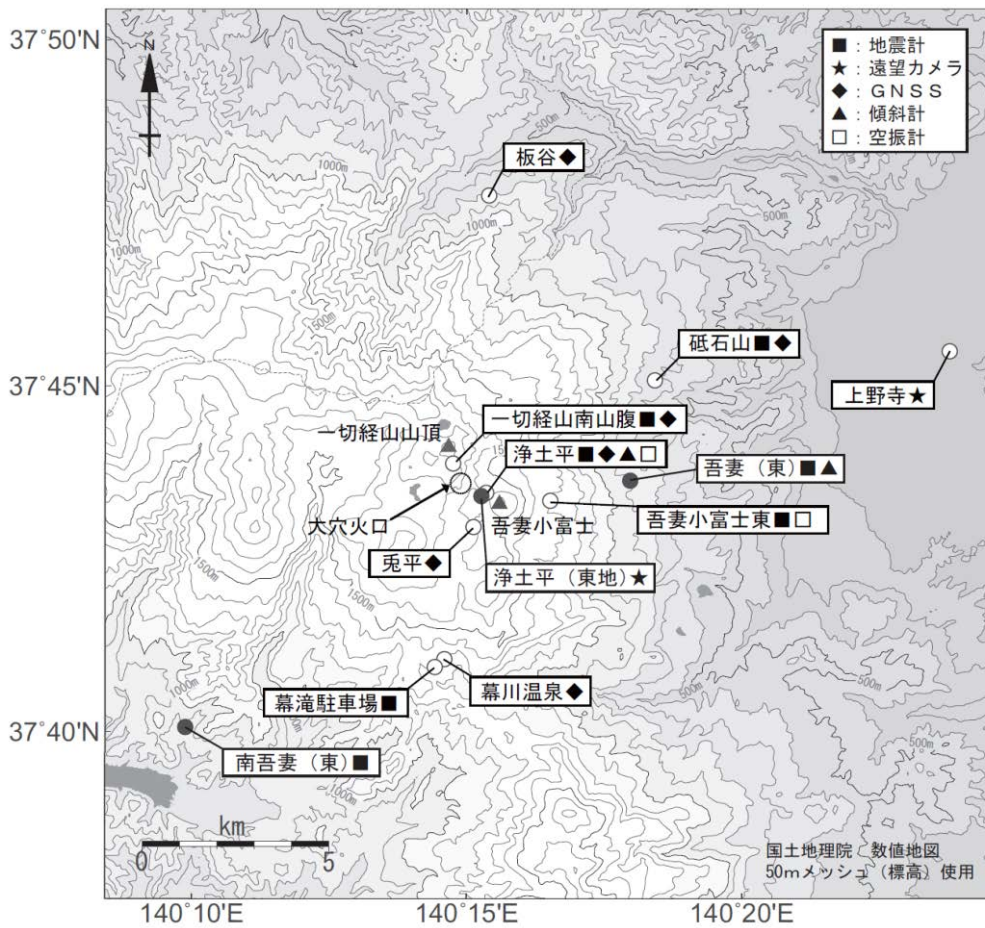
図4 吾妻山 観測点配置図
