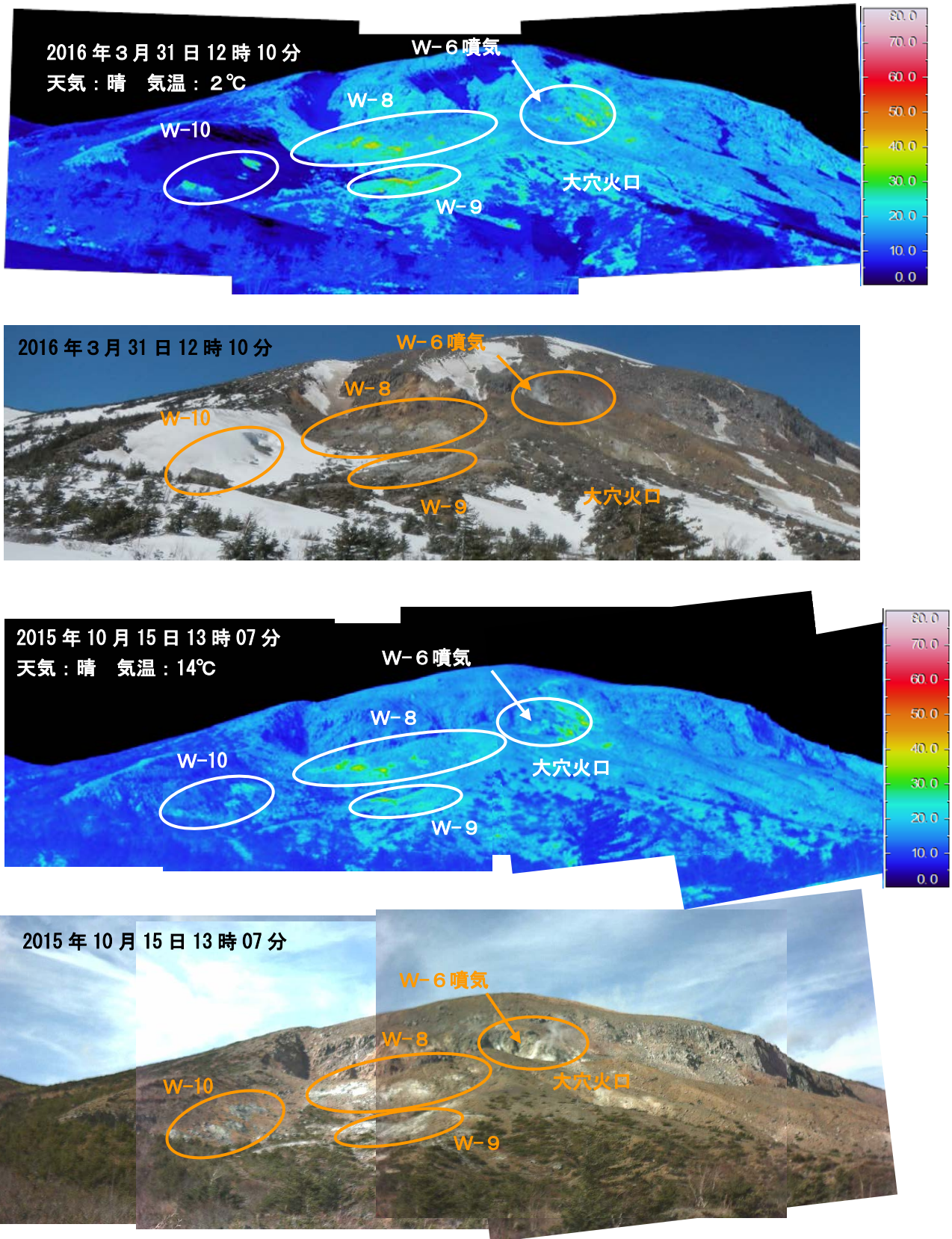
図3 吾妻山 大穴火口及び八幡焼の状況と地表面温度分布
