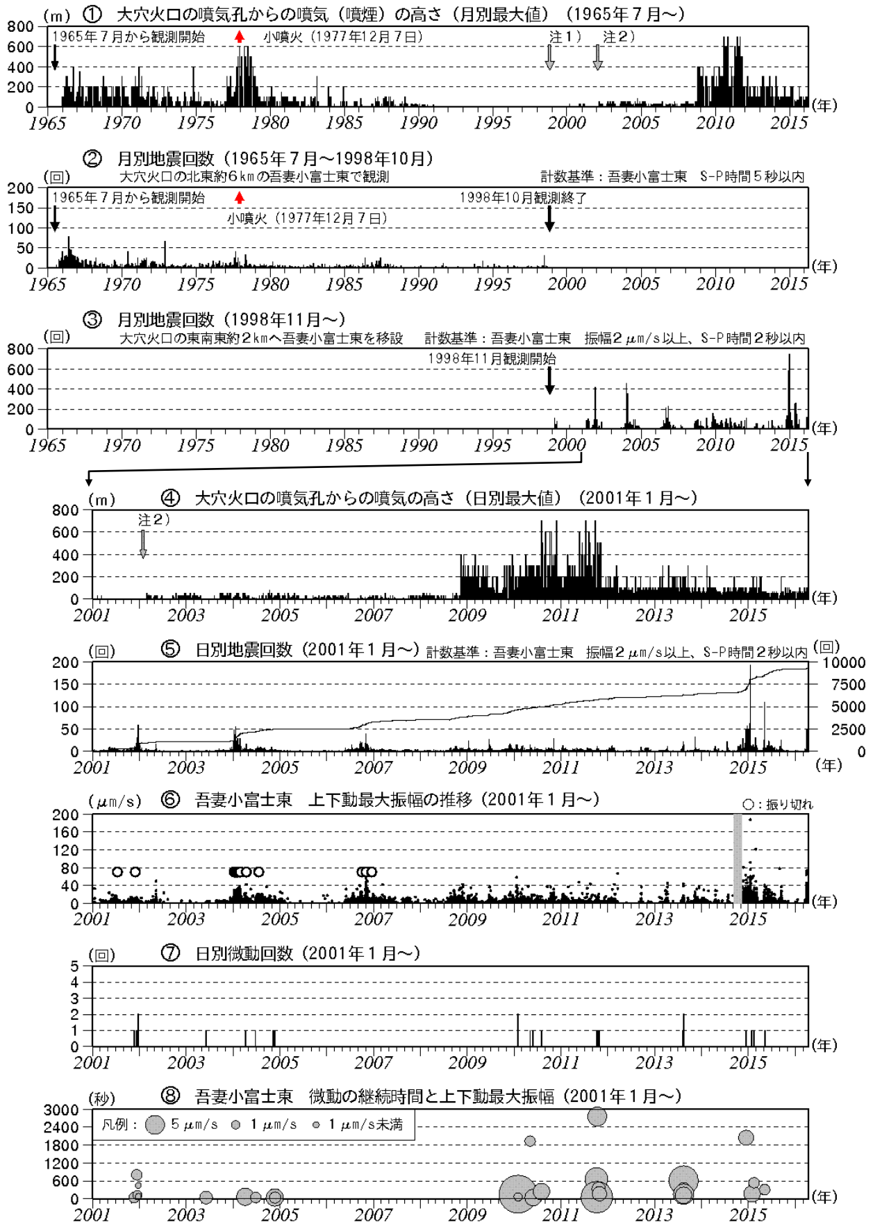
図6 吾妻山 火山活動経過図(1965年7月~2016年3月)
