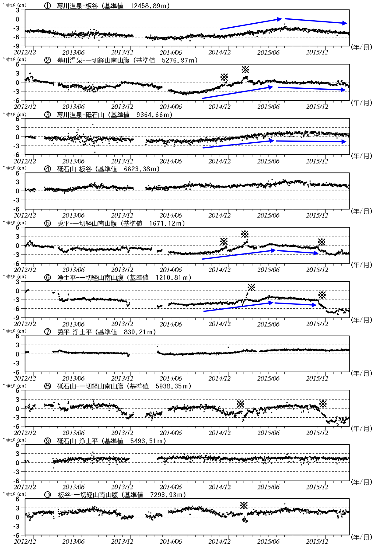
図 10-2 吾妻山 GNSS 基線長変化図 (2012 年 12 月～2016 年 3 月)
