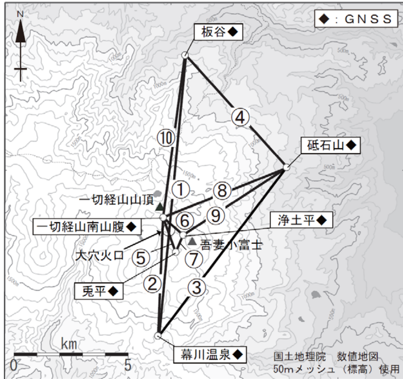
図7 吾妻山 GNSS 観測点配置図 小さな白丸 (○) は気象庁の観測点位置を示しています。
