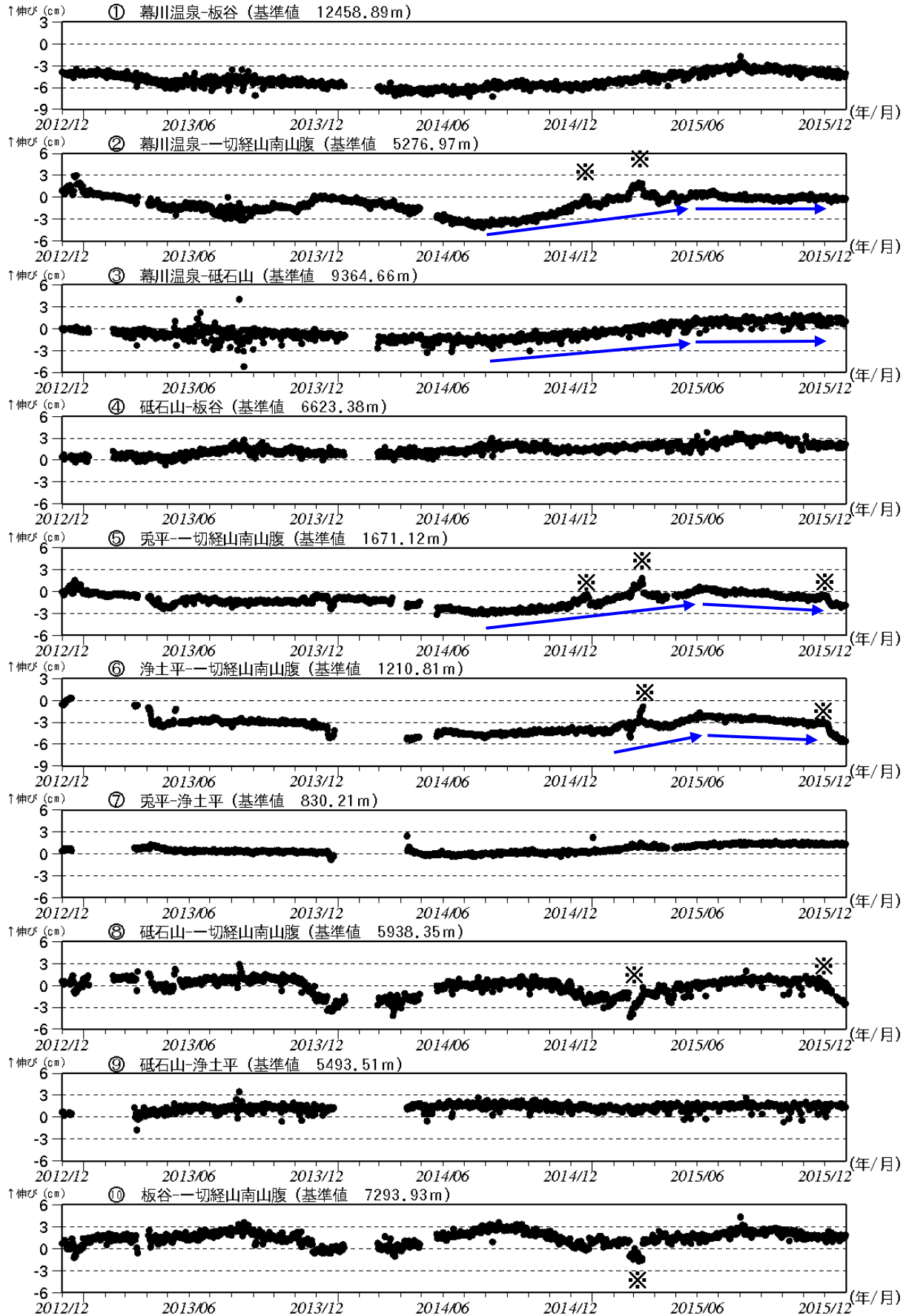
図8-② 吾妻山 GNSS 基線長変化図 (2012 年 12 月～2015 年 12 月)
