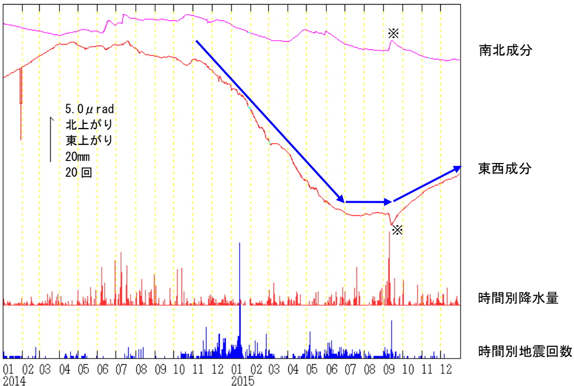
図 6 吾妻山 浄土平観測点での傾斜変動
