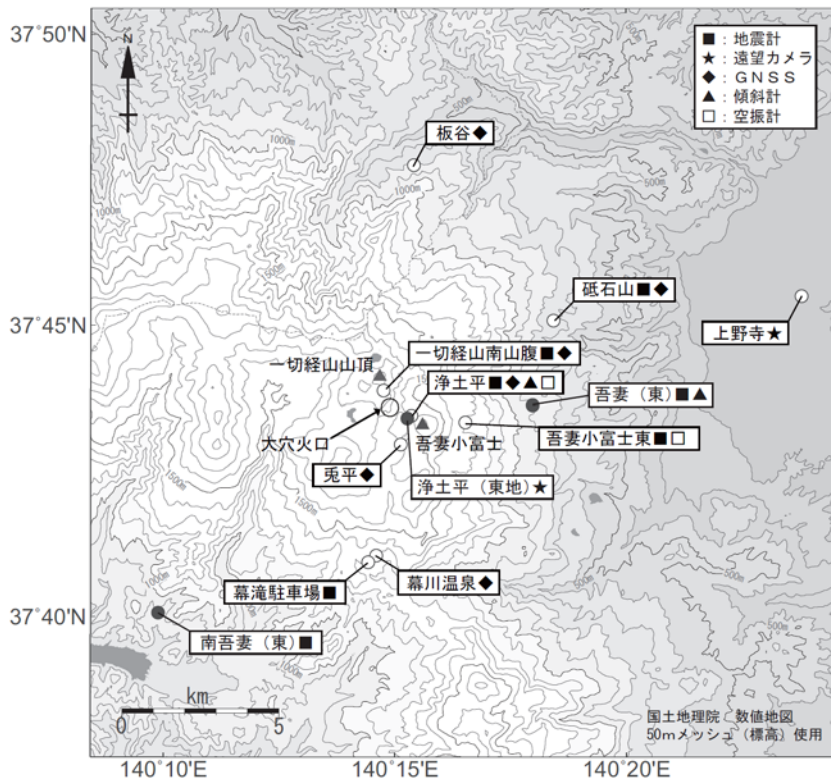
図3 吾妻山 観測点配置図
