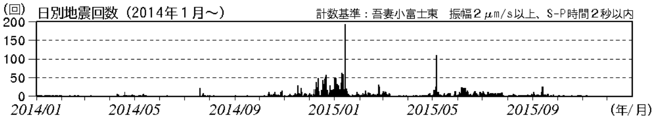
図2 吾妻山 日別地震回数（2014年1月～2015年12月）
