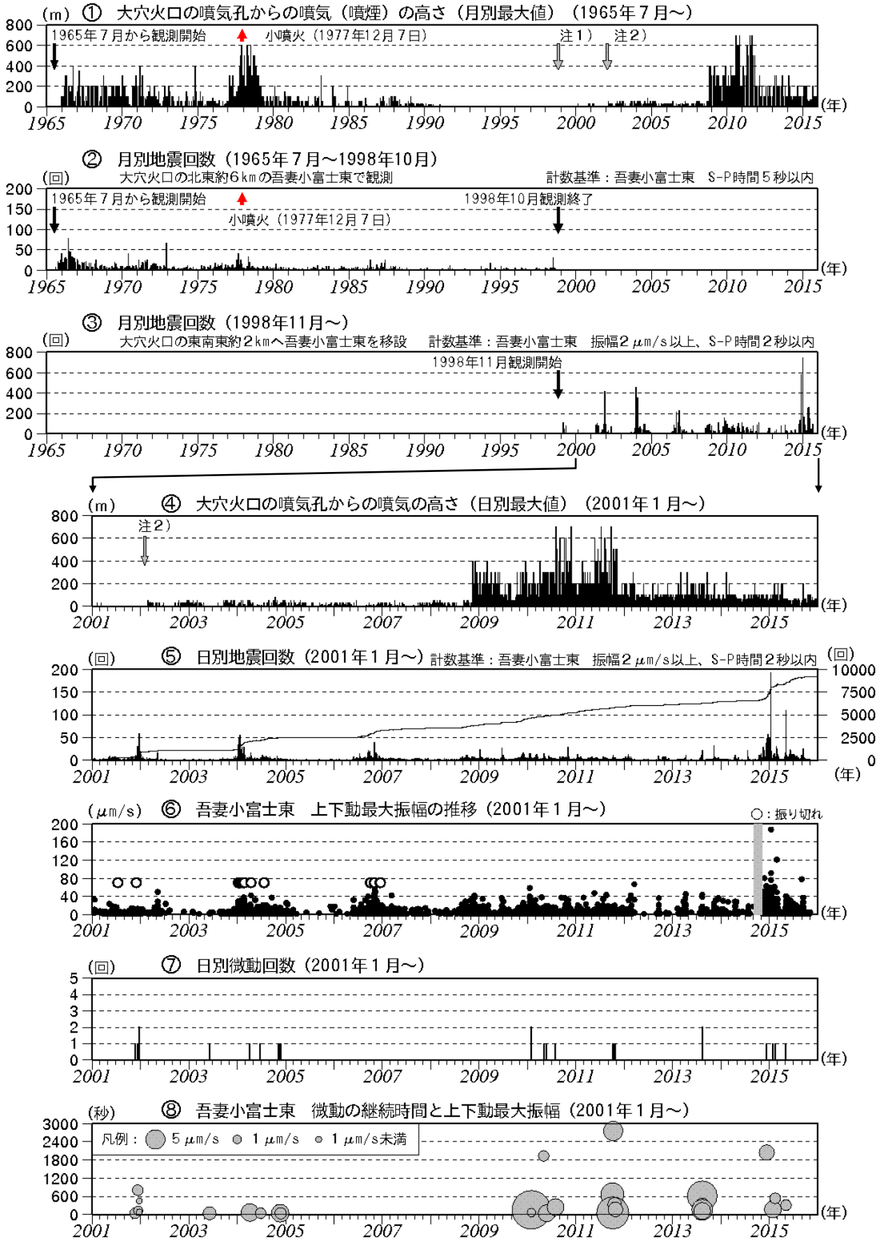
図4 吾妻山 火山活動経過図（1965年7月～2015年12月）
