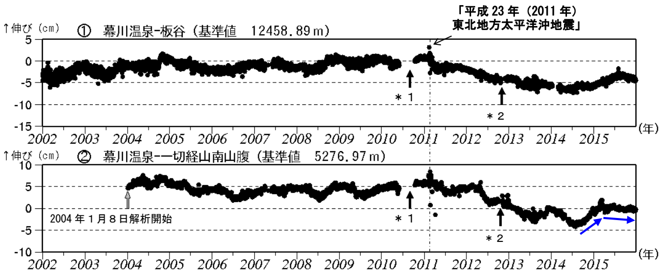
図8-① 吾妻山 GNSS 基線長変化図 (2002 年 1 月～2015 年 12 月)
