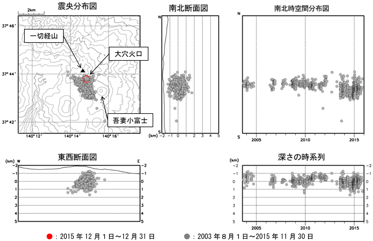
● : 2015 年 12 月 1 日～12 月 31 日 ● : 2003 年 8 月 1 日～2015 年 11 月 30 日
