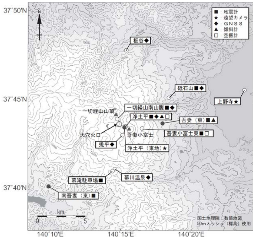
図 2 吾妻山 観測点配置図
