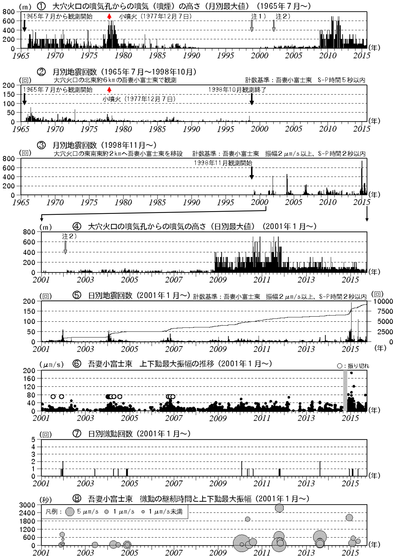
図4 吾妻山 火山活動経過図(1965年7月~2015年9月)
