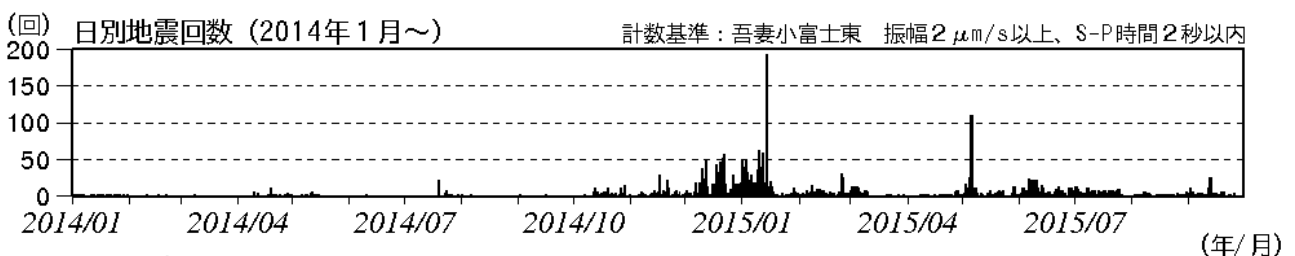
図 3 吾妻山 日別地震回数（2014年1月～2015年9月）
