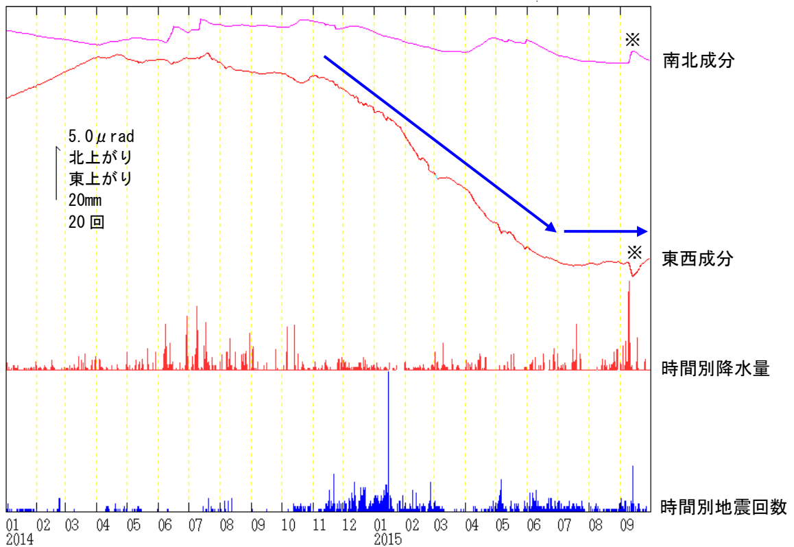
図 6 吾妻山 浄土平観測点での傾斜変動 (2014 年 1 月 1 日～2015 年 9 月 30 日、時間値、潮汐補正あり) ・ 1 \mu\text{rad} (マイクロラジアン) は、 1 \text{ km} 先が 1 \text{ mm} 上下するような変化量です。 ・ 青矢印は傾斜計の変化傾向を示します。 ・ 2014 年 11 月頃からみられている西側上がりの傾向は、2015 年 7 月頃から停滞しています。 ・ 時間別降水量は鷲倉地域気象観測所の値です。 ※平成 27 年 9 月関東・東北豪雨による変動です。
