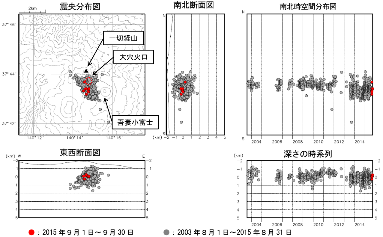
● : 2015 年 9 月 1 日～9 月 30 日 ● : 2003 年 8 月 1 日～2015 年 8 月 31 日 図 5 吾妻山 地震活動 (2003 年 8 月～2015 年 9 月) ・ 2010 年 2 月 24 日～6 月 29 日の震源は、吾妻小富士東の地震計のテレメータ装置の時刻校正に不具合があったため、機器の内部温度で時刻補正值を求め、吾妻小富士東の検測値を補正しました。 ・ 2012 年 12 月 1 日以降、観測点の移設更新の影響により、震源がやや南側に分布する傾向がみられます。
