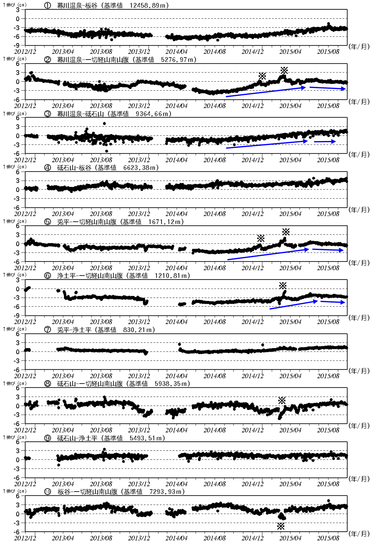
図8-② 吾妻山 GNSS 基線長変化図 (2012年12月～2015年9月)
