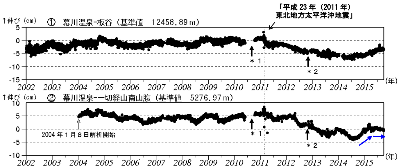
図8-① 吾妻山 GNSS 基線長変化図 (2002 年 1 月～2015 年 9 月)
