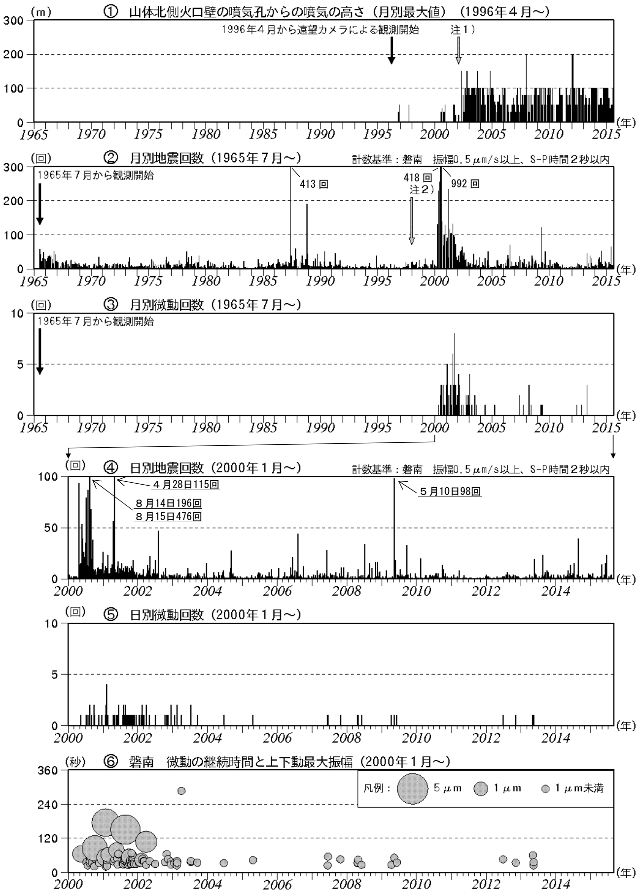
図2 磐梯山 火山活動経過図（1965年7月～2015年8月）
