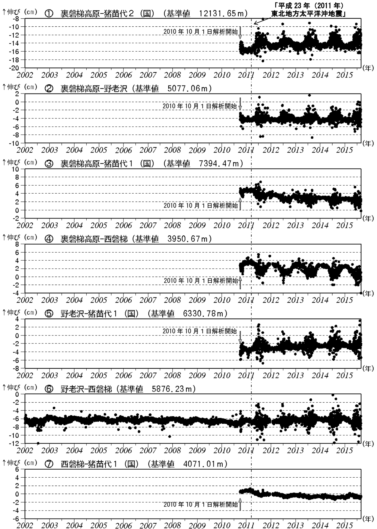
図3 磐梯山 GNSS 1) 基線長変化図 (2002年1月～2015年8月)
