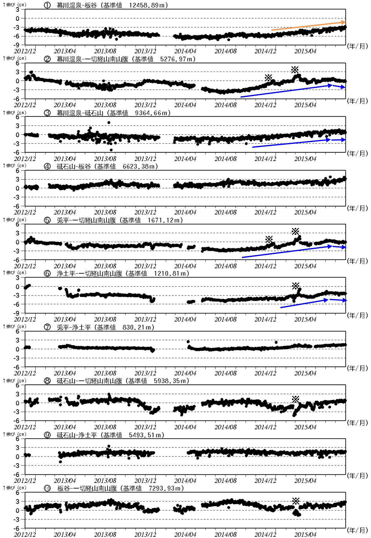
図 8-② 吾妻山 GNSS 基線長変化図 (2012 年 12 月～2015 年 7 月)
