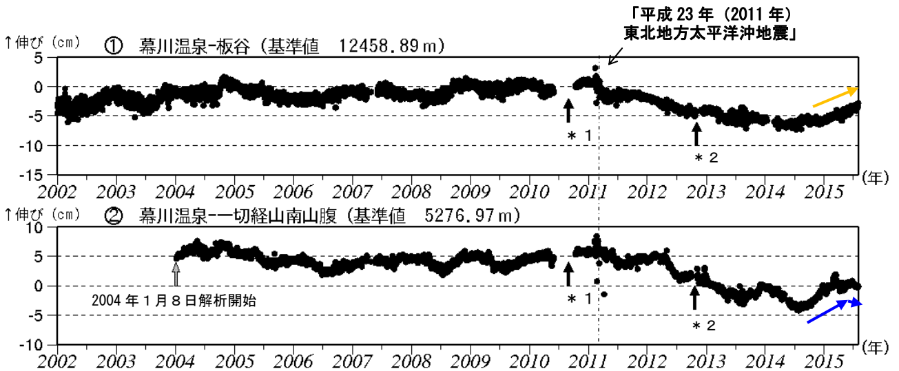
図8-① 吾妻山 GNSS 基線長変化図 (2002 年 1 月～2015 年 7 月)
