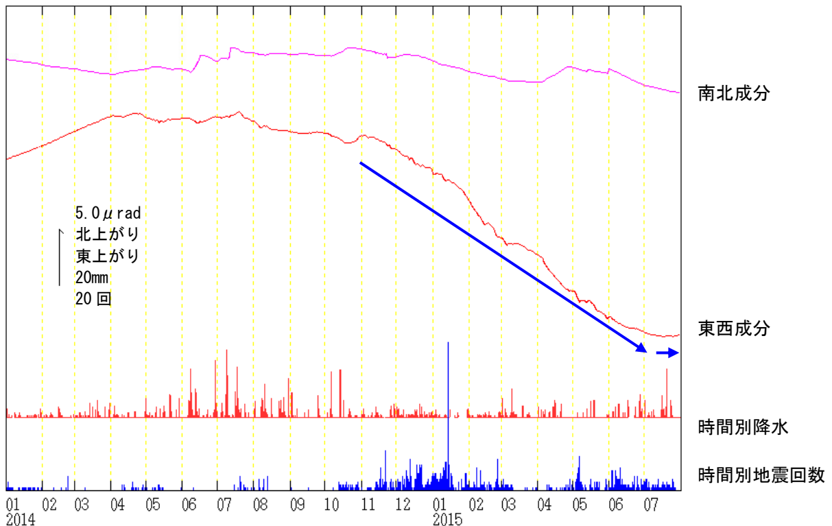
図 6 吾妻山 浄土平観測点での傾斜変動
