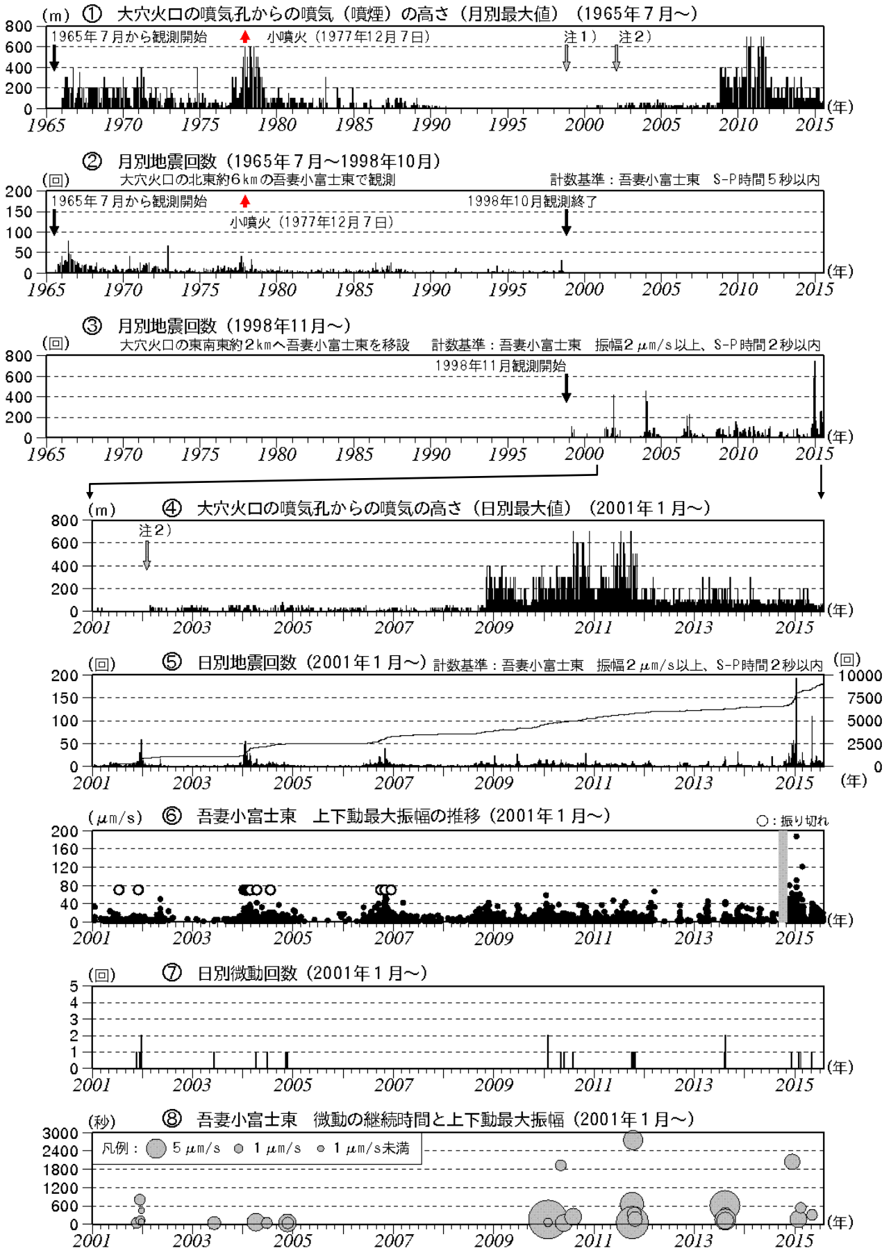
図4 吾妻山 火山活動経過図 (1965年7月～2015年7月)
