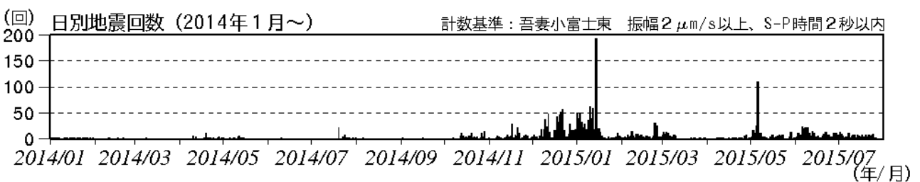
図 3 吾妻山 日別地震回数（2014年1月～2015年7月）
