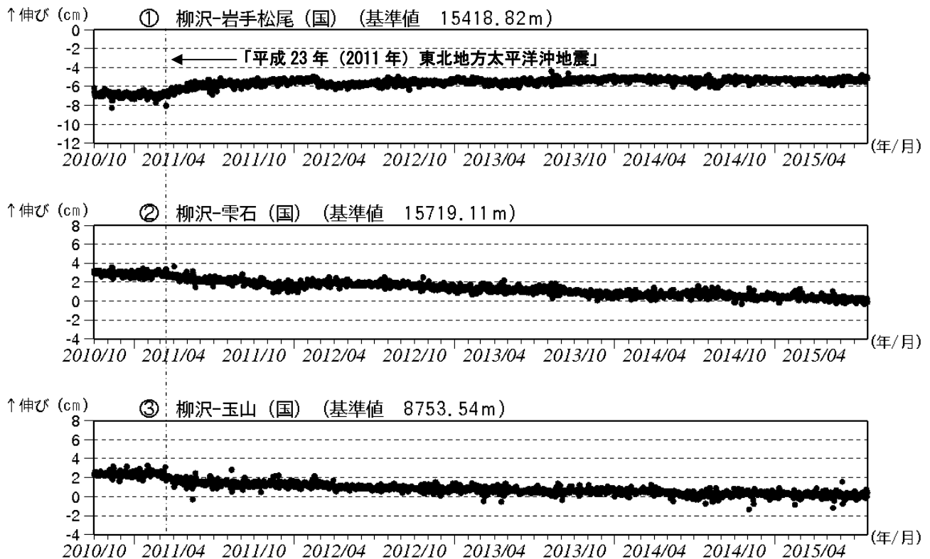
図 3 岩手山 GNSS 1) 基線長変化図 (2010 年 10 月～2015 年 7 月)
