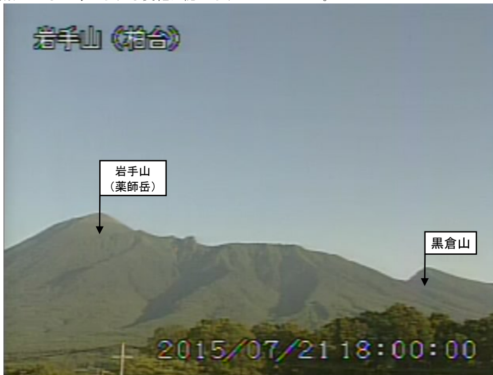
図 1 岩手山 黒倉山の噴気の状況（7月21日）
