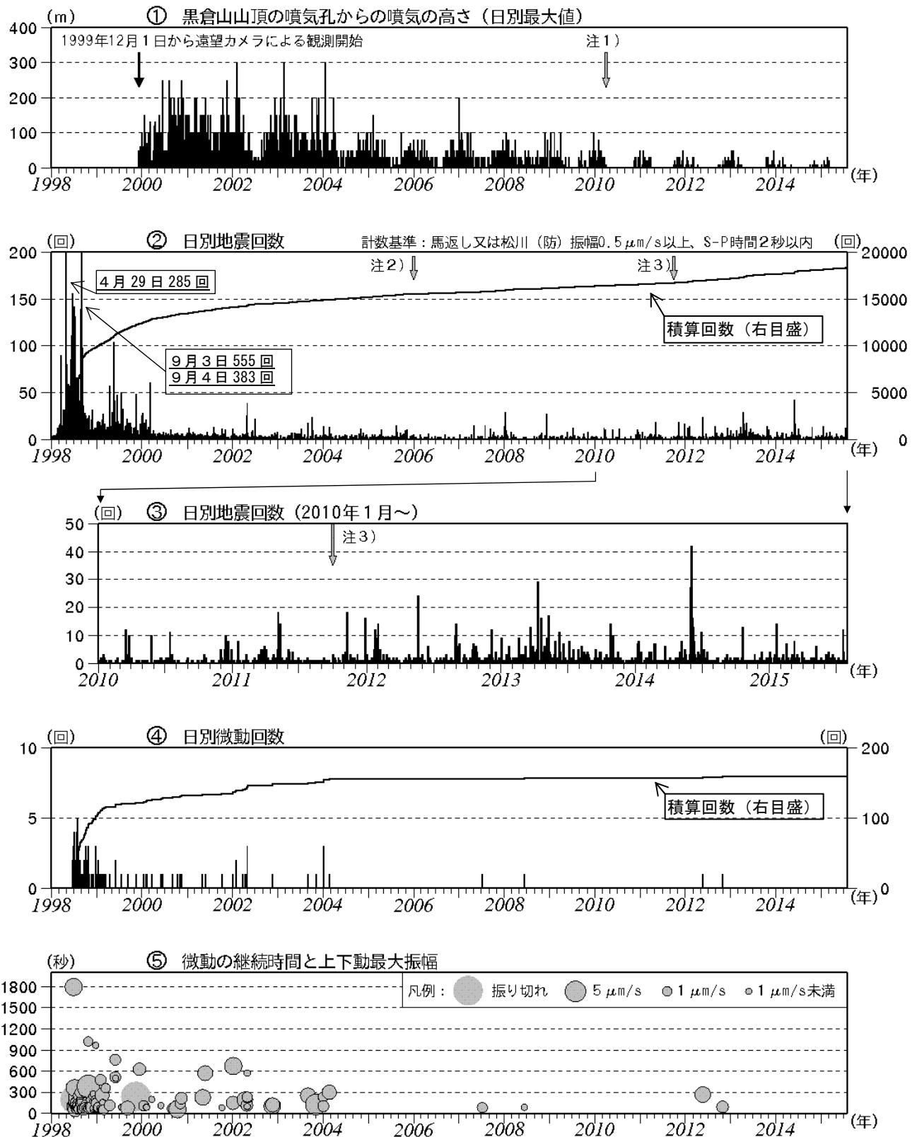
図2 岩手山 火山活動経過図（1998年1月～2015年7月）
