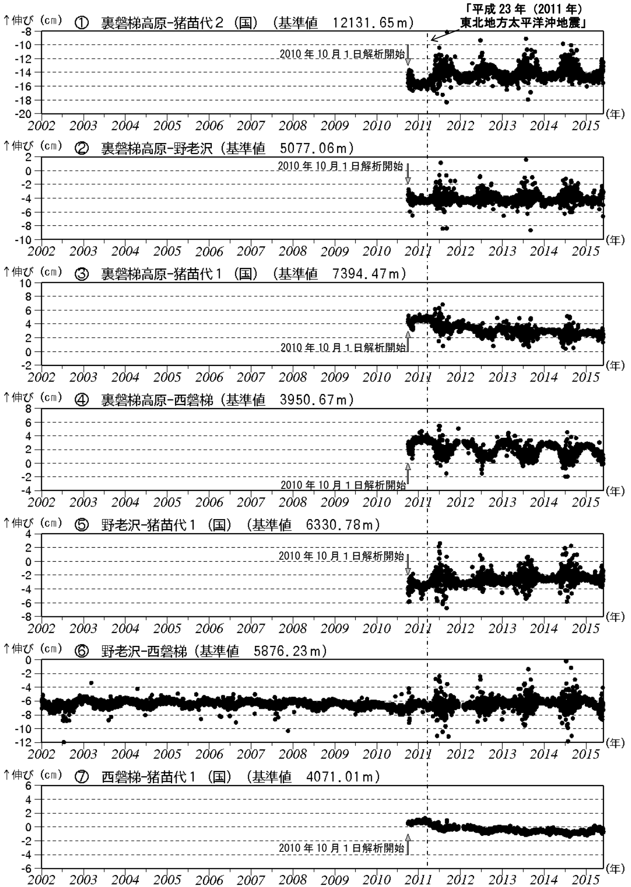
図3 磐梯山 GNSS 1) 基線長変化図 (2002 年 1 月～2015 年 5 月)
