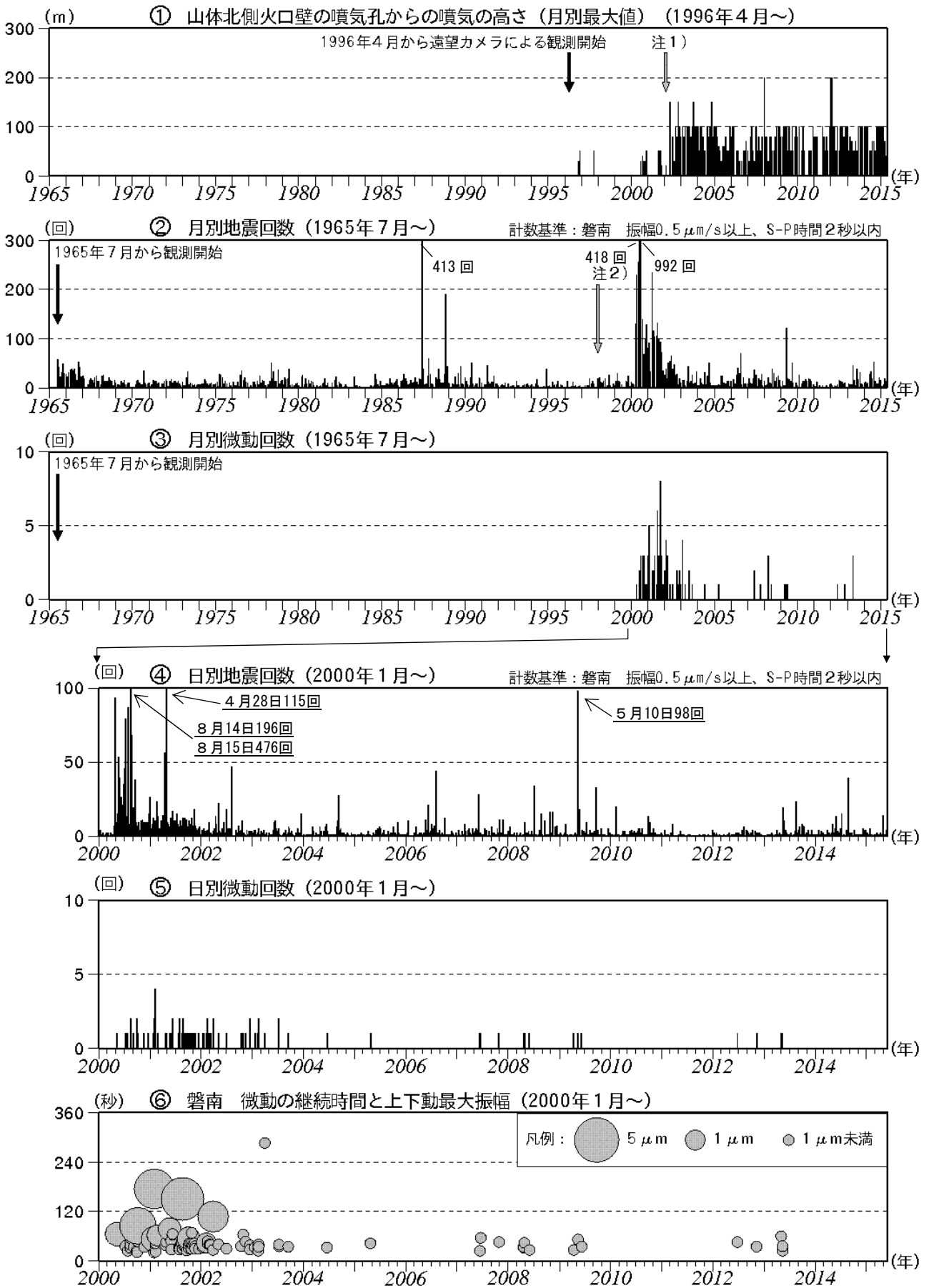
図2 磐梯山 火山活動経過図（1965年7月～2015年5月）
