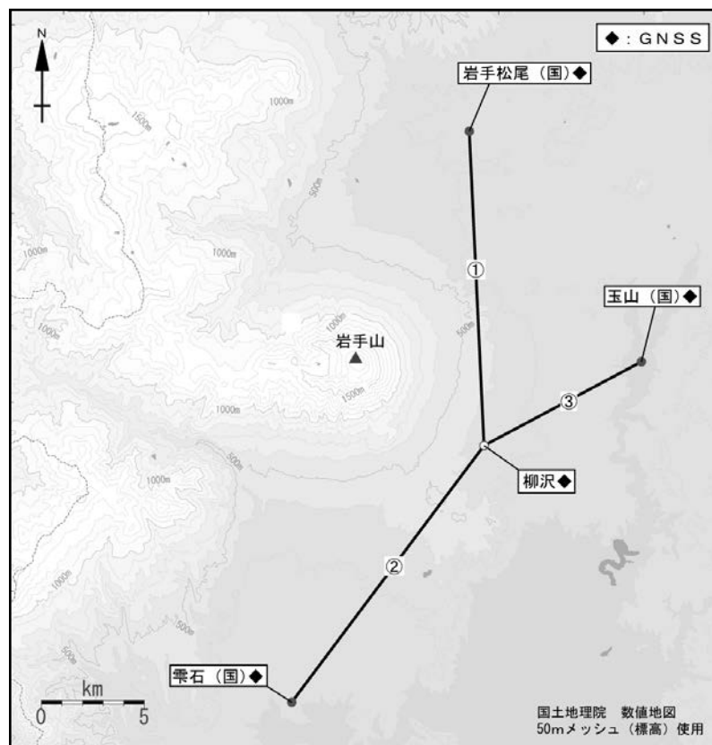
図 5 岩手山 GNSS 1) 観測点配置図
