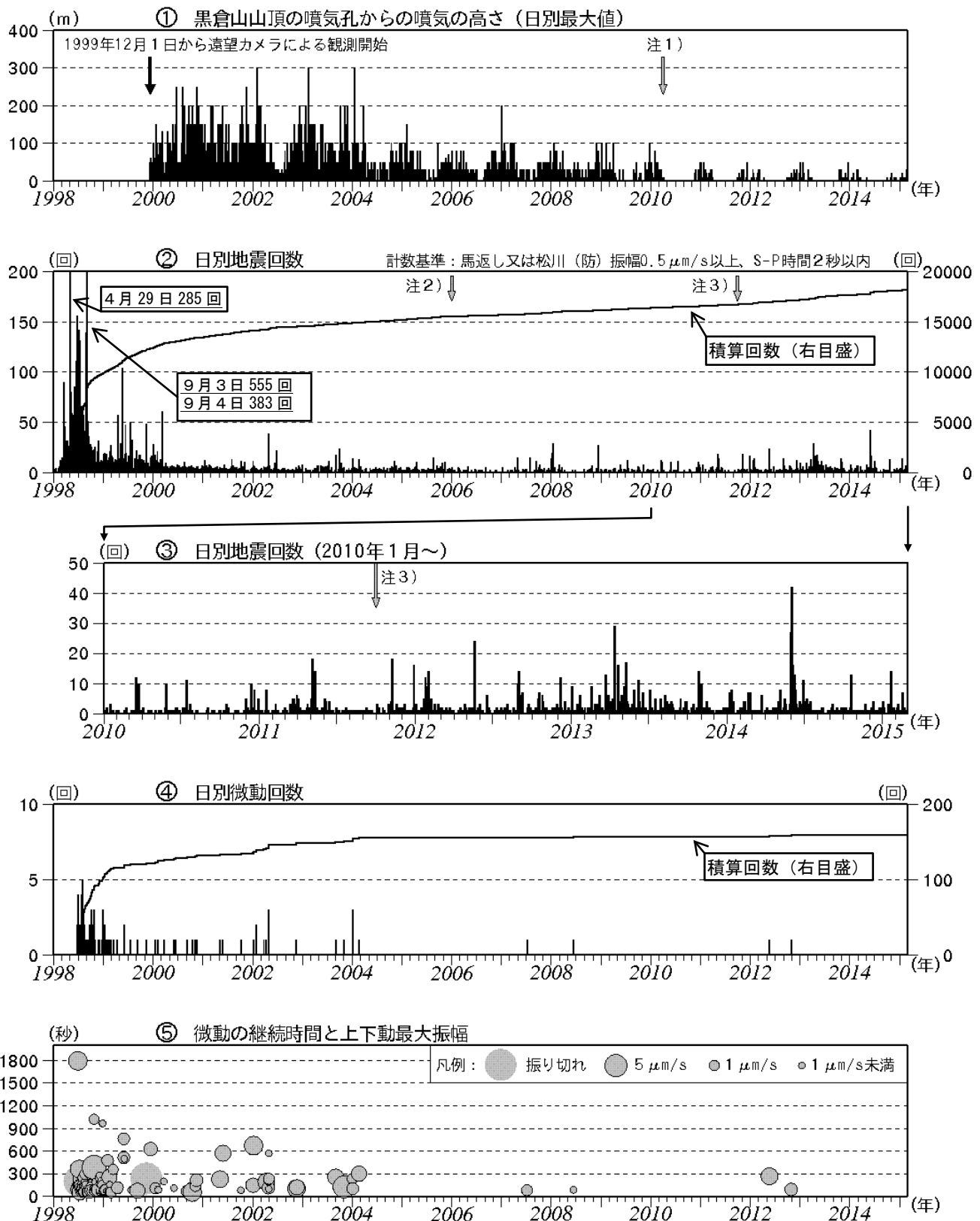
図2 岩手山 火山活動経過図（1998年1月～2015年2月）
