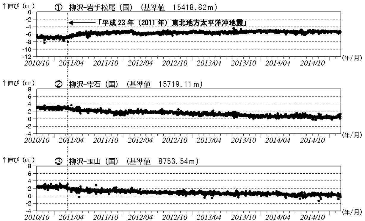
図3 岩手山 GNSS 基線長変化図 (2010 年 10 月～2015 年 2 月)
