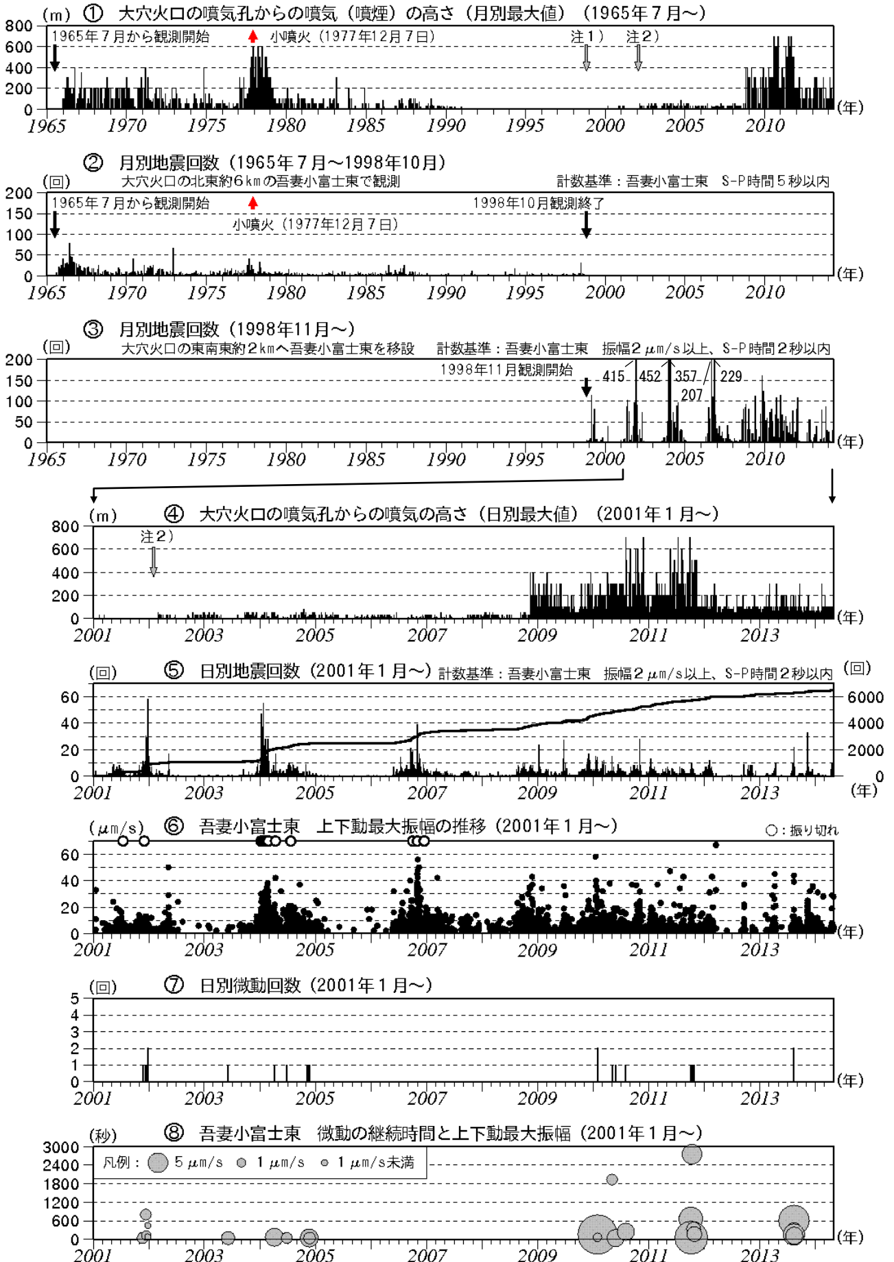
図2 吾妻山 火山活動経過図 (1965年7月~2014年4月)
