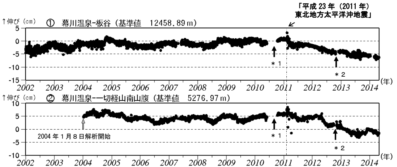
図4 吾妻山 GNSS 基線長変化図 (2002 年 1 月～2014 年 4 月)
