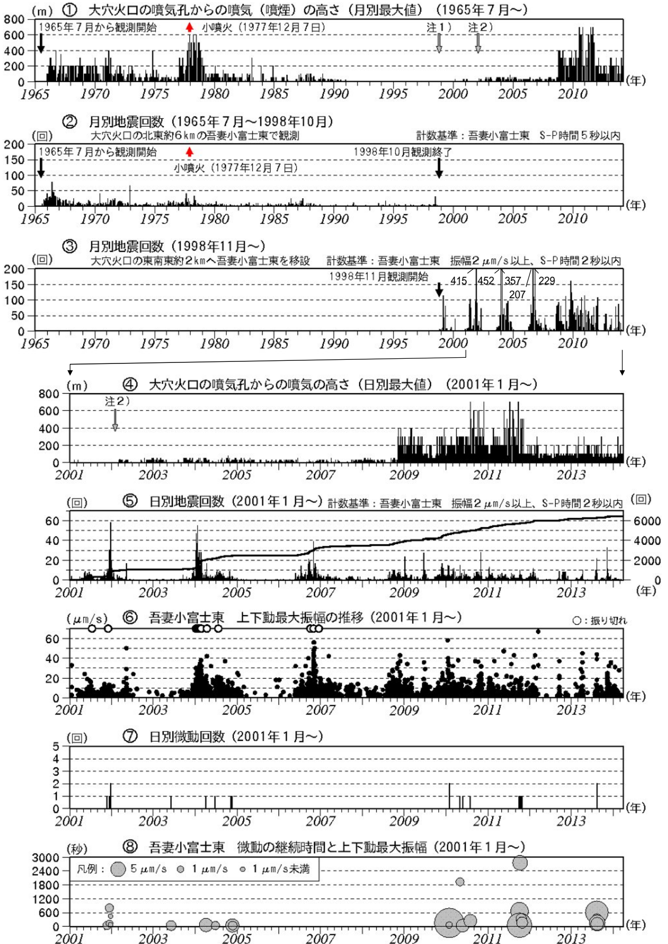
図2 吾妻山 火山活動経過図（1965年7月～2014年3月）
