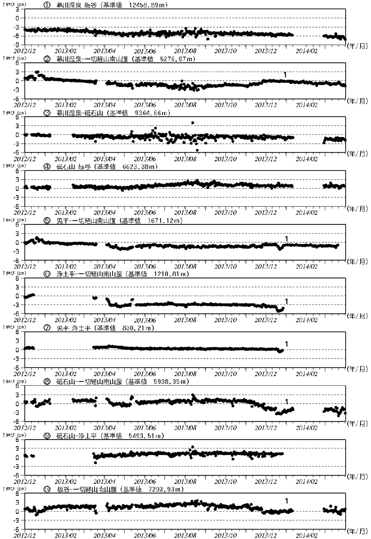
図5 吾妻山 GNSS 基線長変化図(2012年12月~2014年3月)
