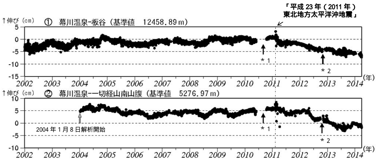
図4 吾妻山 GNSS 基線長変化図 (2002 年 1 月 ~ 2014 年 3 月)
