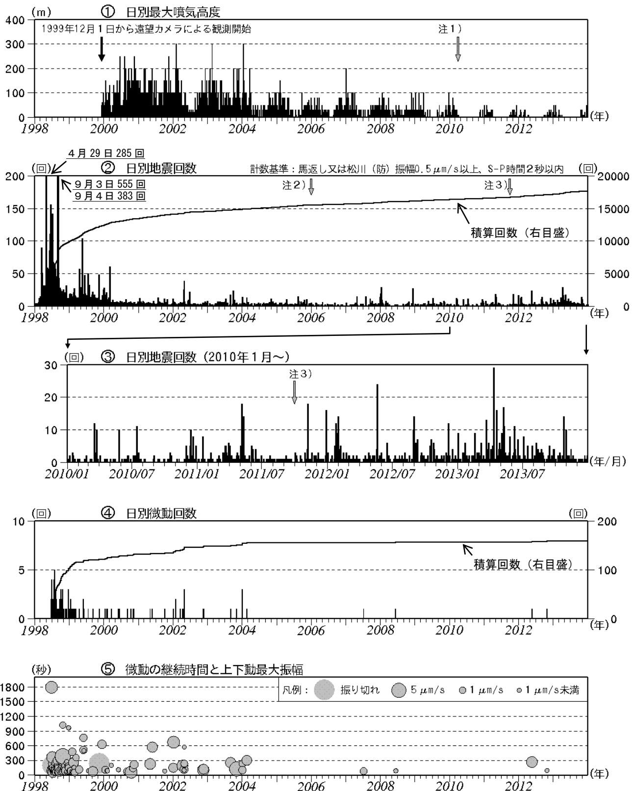
図6 岩手山 火山活動経過図（1998年1月～2013年12月）
