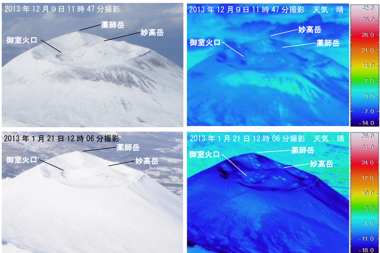
図3 岩手山 山頂部の地表面温度分布 1) と可視画像
