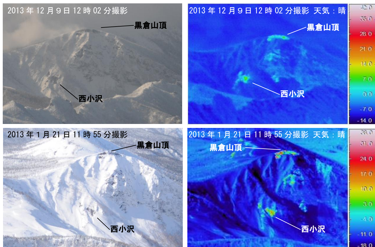
図 4 岩手山 黒倉山東側崖面と西小沢の可視画像（左）と地表面温度分布 1) （右）
