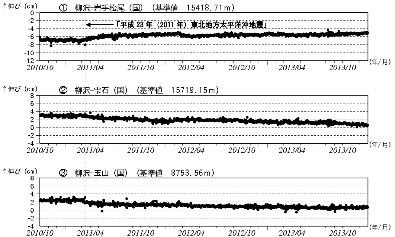
図8 岩手山 GPS 基線長変化図 (2010 年 10 月～2013 年 12 月)
