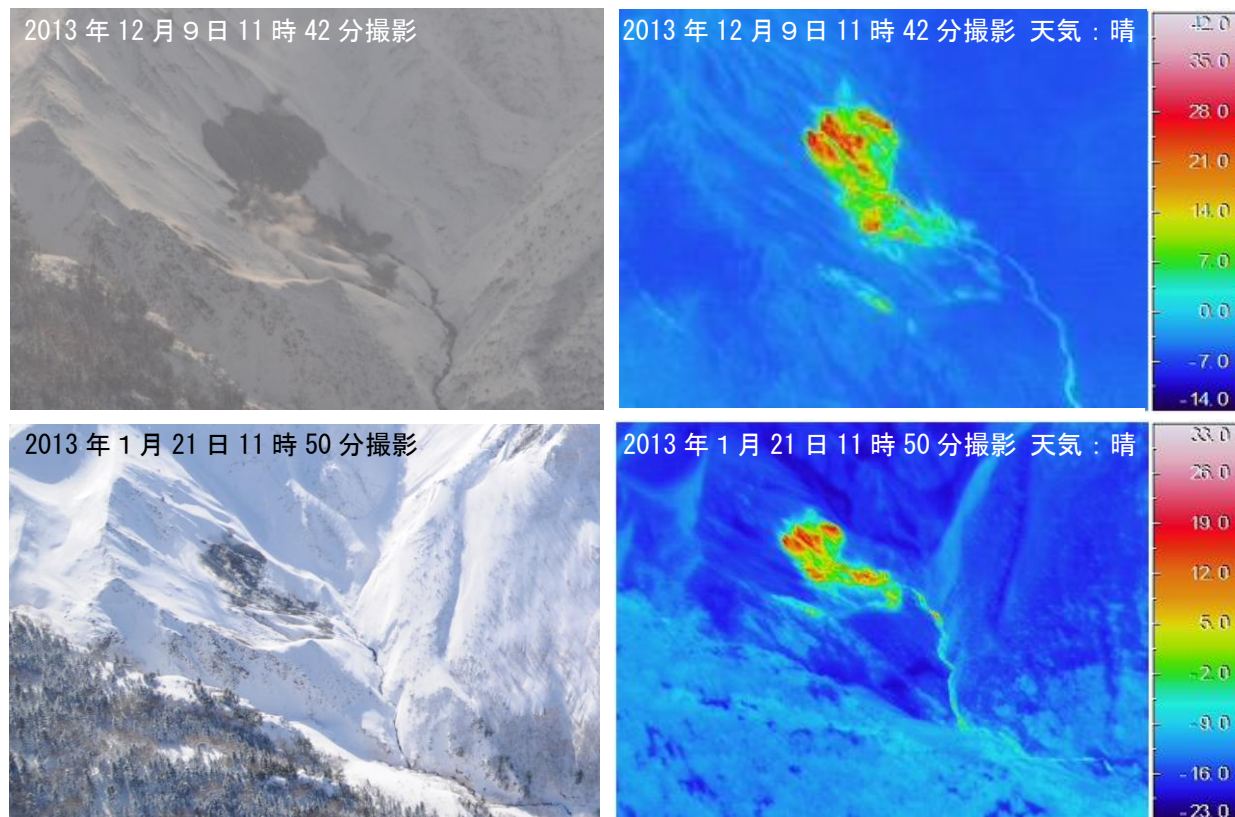
図 5 岩手山 大地獄谷の可視画像と地表面温度分布 1)
