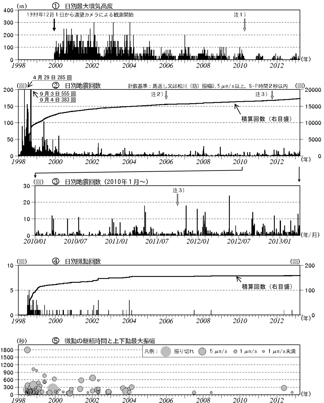
図2※ 岩手山 火山活動経過図（1998年1月～2013年3月）
