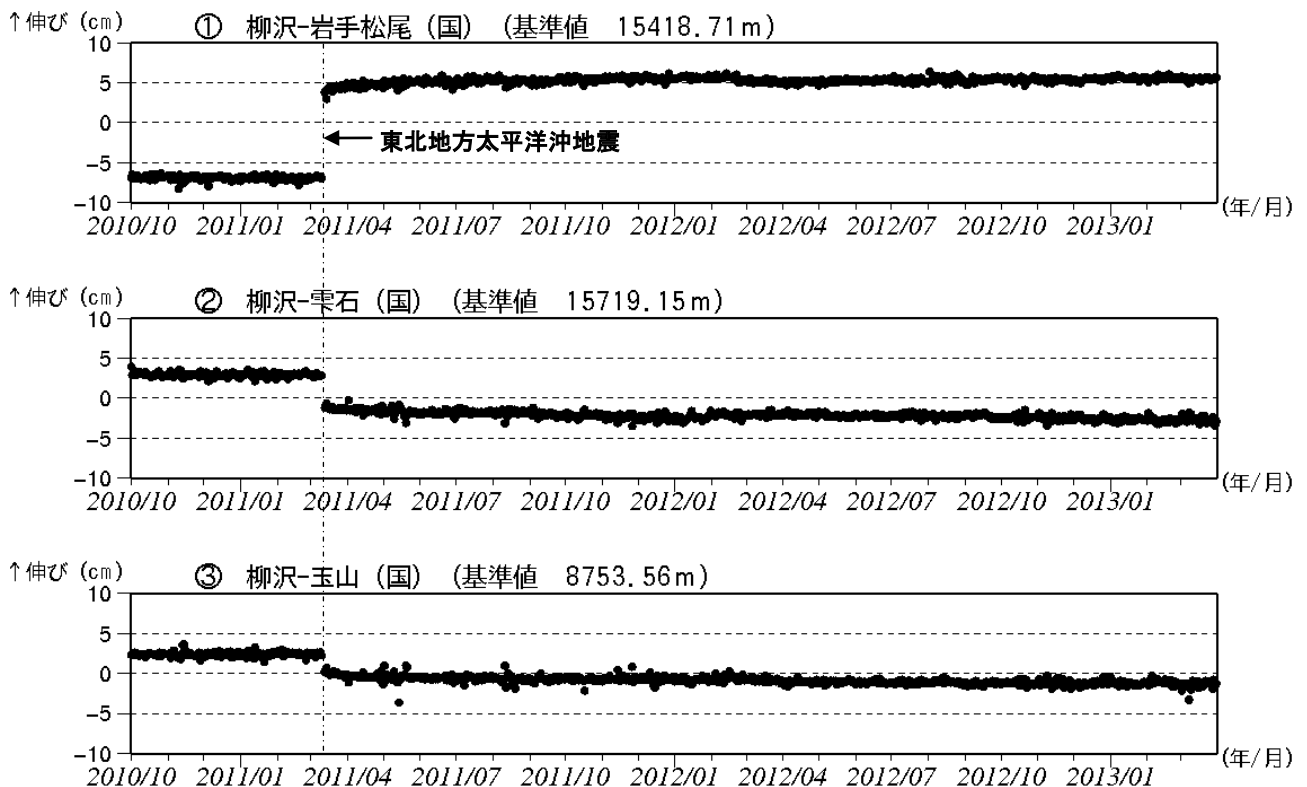
図4※ 岩手山 GPS 基線長変化図（2010 年 10 月～2013 年 3 月）
