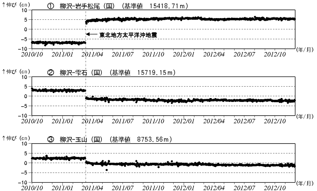
図4※ 岩手山 GPS 基線長変化図（2010年10月～2012年11月）
