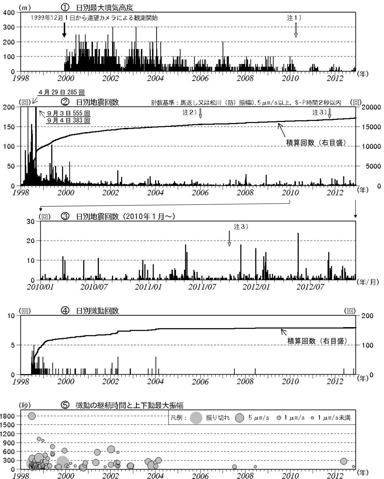
図2※ 岩手山 火山活動経過図（1998年1月～2012年11月）
