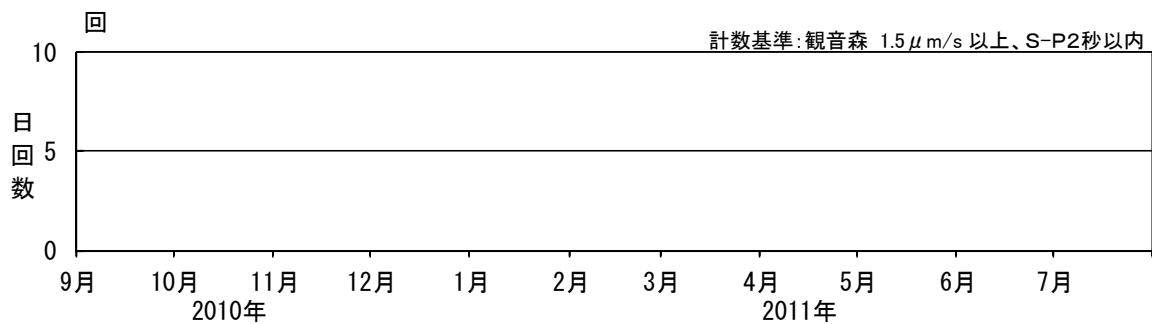
図3 鳥海山 火山性地震の日別回数（2010年9月～2011年7月）
