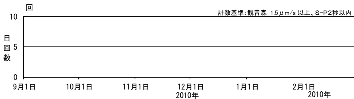
図3 鳥海山 火山性地震の月別回数（2010年9月～2011年2月）
