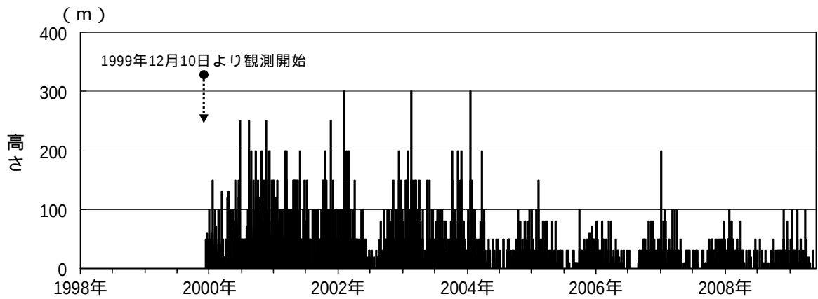
図 2 岩手山 日最大噴気の高さ（黒倉山）（1999 年 12 月～2009 年 5 月）
