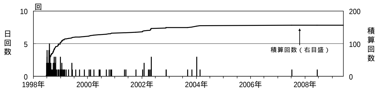
図 4 岩手山 日別微動回数（1998 年 1 月～2009 年 5 月）
