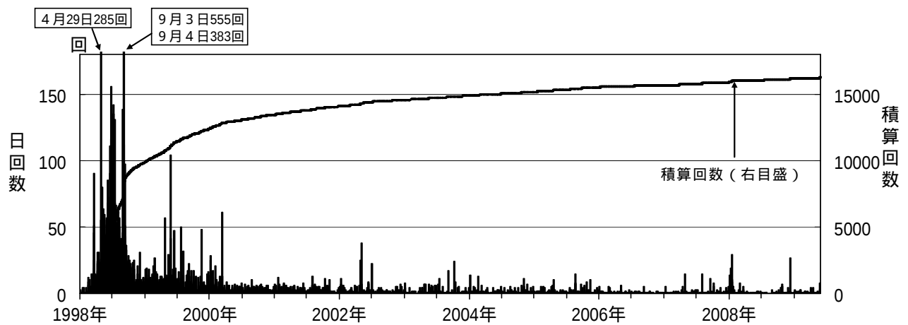
図 3 岩手山 日別地震回数（1998 年 1 月～2009 年 5 月）
